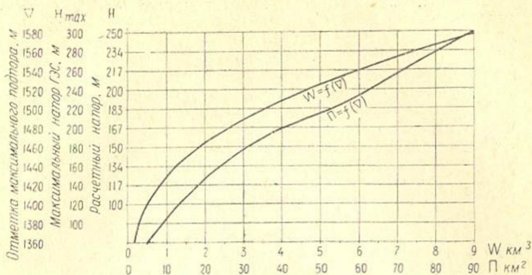
Рис. 58. Емкость W и площадь зеркала P проектируемого водохранилища многолетнего регулирования стока в зависимости от отметки подпора
