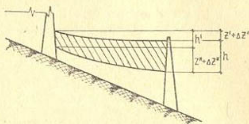
Рис. 18. К определению коэффициента потерь напора.
