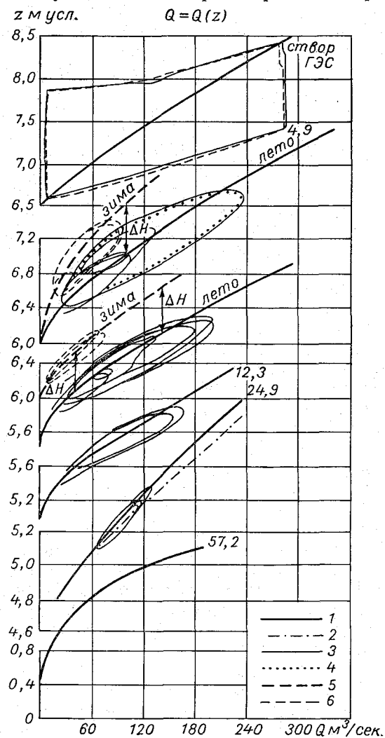
Рис. 9.2. Кривые связи расходов и уровней воды для Верхней Волги.
