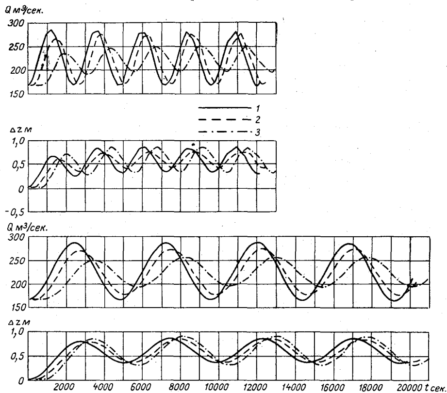
Рис. 10.12. Изменение во времени расходов и уровней для задачи 4г ( T=2400 сек. и T=4800 сек.). Усл. обозначения см. рис. 10.5.
