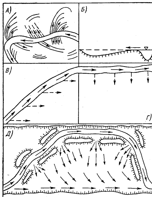
Рис. 8.17. Особенности затекания воды на пойму сложного строения.
