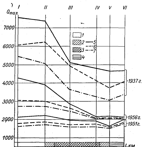
Рис. 8.13. Снижение максимальных (5), максимальных пентадных (6) и максимальных декадных (7) расходов вдоль пойменного участка р. Иртыша в характерные по водности годы.
