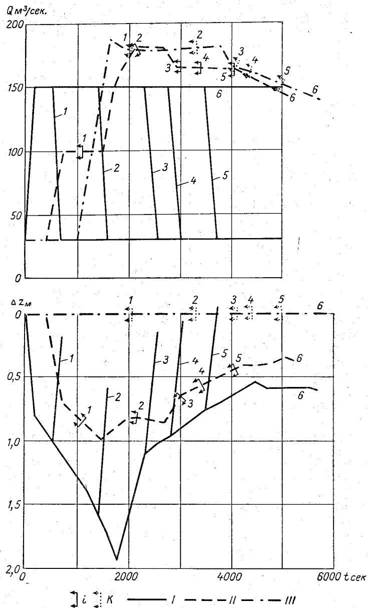
Рис. 10.3. Совмещенные кривые хода расходов и уровней для задачи 1б.
