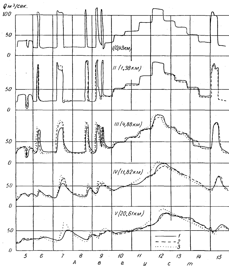
Рис. 9.5А. Гидрографы для р. Тверцы.
