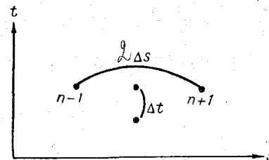
Рис. 4.3. Неявная схема Института гидродинамики СО АН СССР (схема ИГ).
