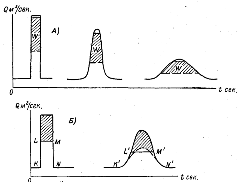
Рис. 8.10. Схема изменения формы частей объема попуска от створа к створу (А) и схема изменения формы гидрографа для полного и усеченного попуска (Б).
