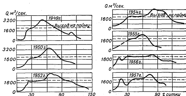
Рис. 10.27. Гидрографы половодья у подпота Черлак на р. Иртыше за различные годы.
