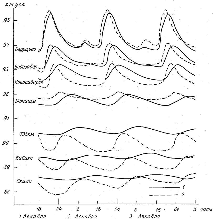
Рис. 9.10. Изменение во времени уровней в нижнем бьефе Новосибирской ГЭС (1) и результаты расчета для первого варианта (2).
