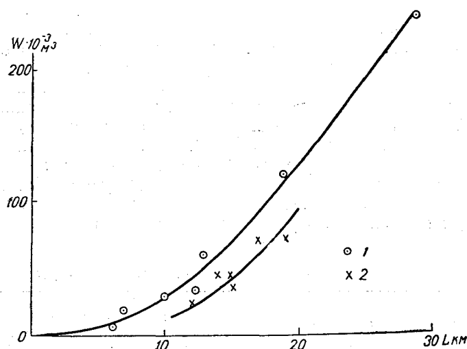
Рис. 10.20. Влияние объема попуска на расстояние выклинивания петель.
