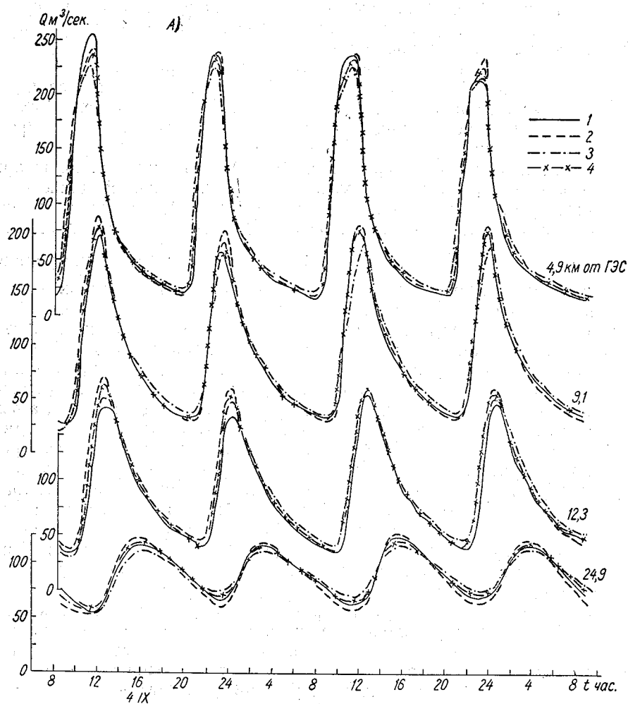
Рис. 9.3. Графики хода уровней (А) и расхода 1 — натурные данные; 2—4 — расчет: 2 — задание K по t_{ср} ,
