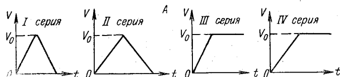
Рис. 11.1. Графики воспроизведения волн.
