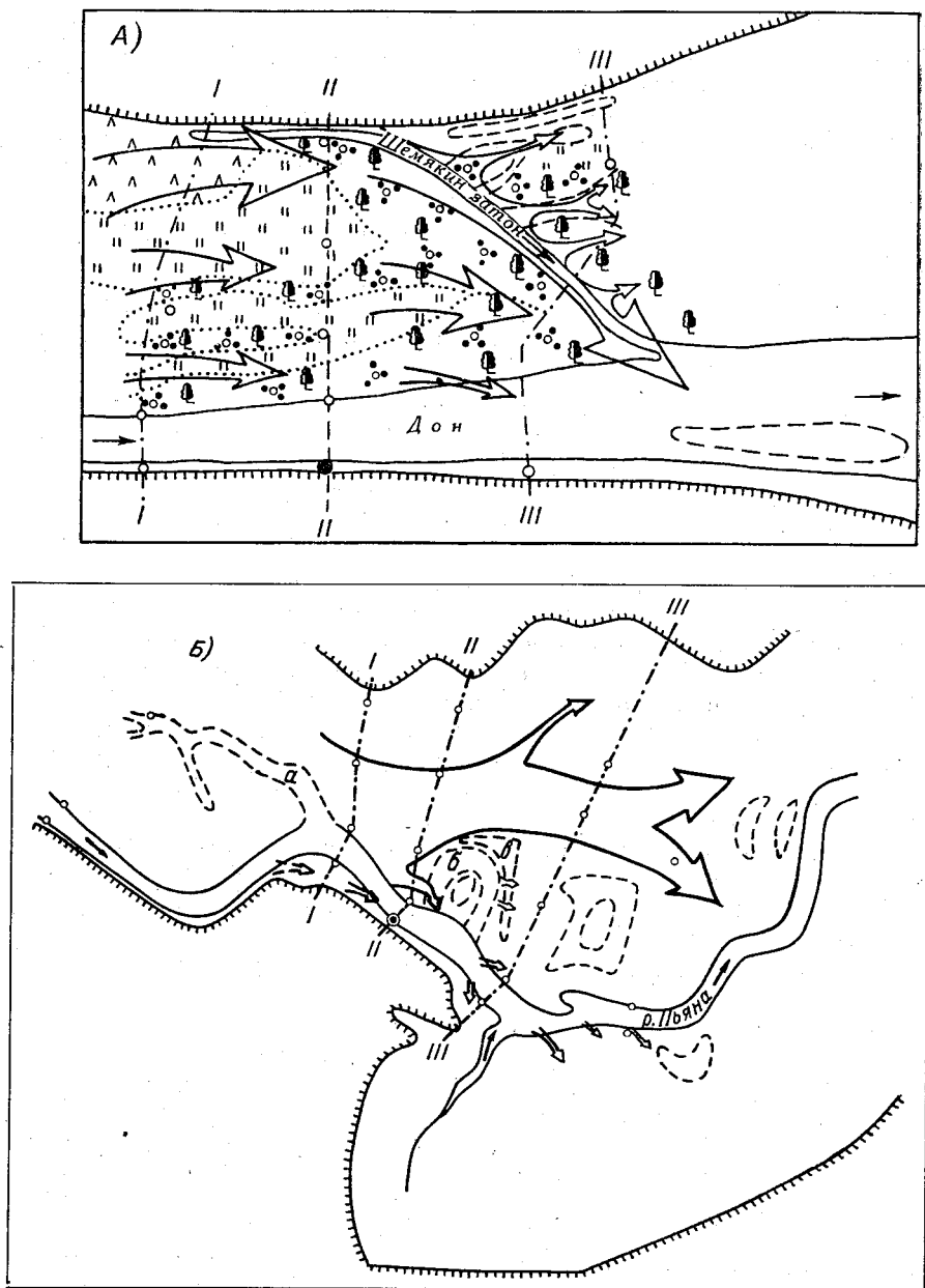
Рис. 8.18. Схематические планы участков природных исслед. А — на р. Дону у х. Хованского, Б — на р. Пьяна у с. Камкино, В — на р. Луге главного русла, притоков, рукавов, озер, 3 — контуры основных повышений рельефа, течений, 6 — основной водпост, 7 — уклонные водпосты, 8 — гидро
