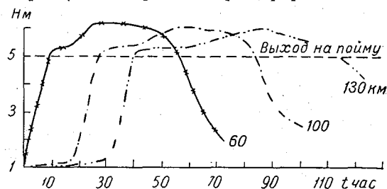
Рис. 10.29. Профиль волны в створах 60, 100 и 130 км.
