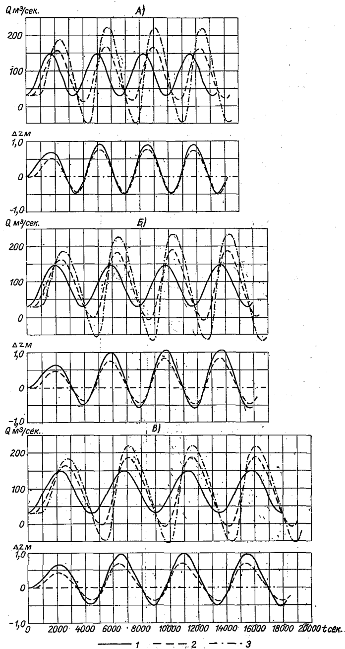
Рис. 10.10. Изменение во времени расходов и уровней для задачи 2г.
