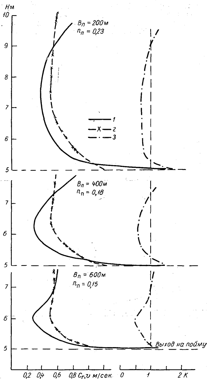
Рис. 10.21. Зависимости c_r и k от H при различной ширине поймы ( \beta=0,45 ; n_n \neq \text{const} ). 1 — c_r , 2 — v , 3 — k .
