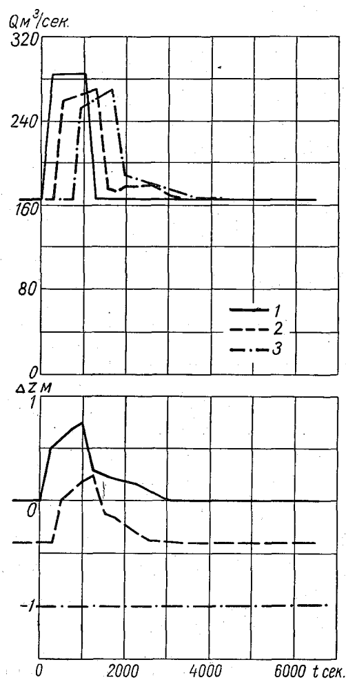
Рис. 10.7. Изменение во времени расходов и уровней для задачи 36. Усл. обозначения см. рис. 10.5.
