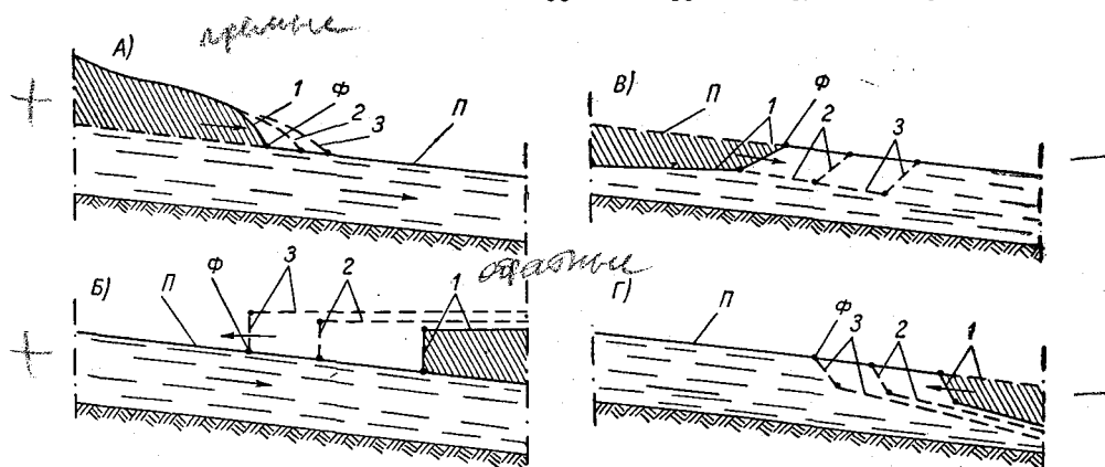
Рис. 1.2. Типы волн при неустановившемся движении воды в открытых руслах. А — волна наполнения, Б — волна подпора, В — волна отлива, Г — волна излива; 1—3 — последовательные положения свободной поверхности, П — ее начальное положение, Ф — фронт волны.
