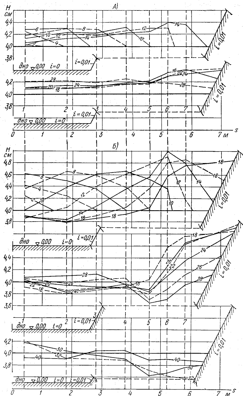
Рис. 11.5. Мгновенные профили волн при наклонном дне с уклоном i=0,01 .
