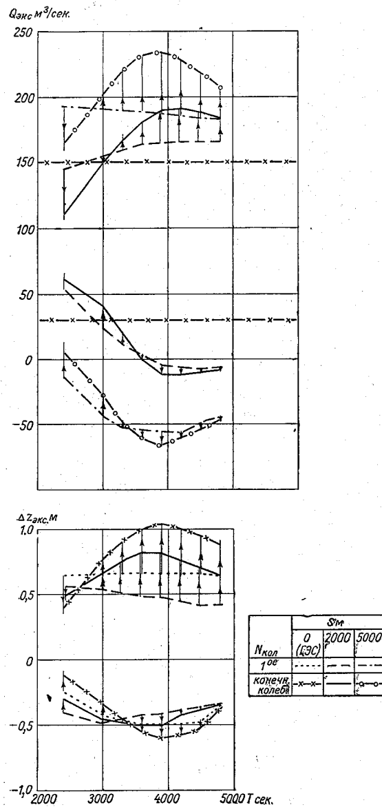
Рис. 10.11. Экстремальные значения Q и \Delta z для первого и конечного колебаний в функции от T (задача 2г).
