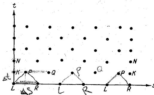
Рис. 4.1. Разностная шахматная схема.
