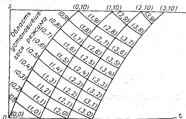
Рис. 4.5. Порядок построения сетки характеристик.
