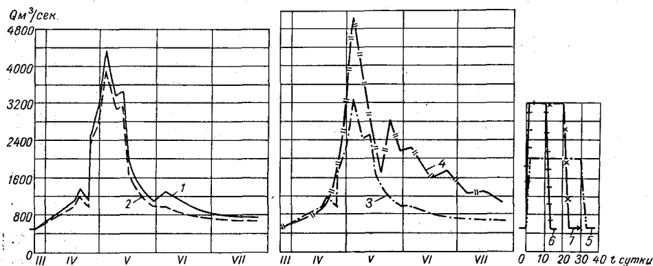
Рис. 9.7. Расчетные варианты входного гидрографа у с. Шульбы.
