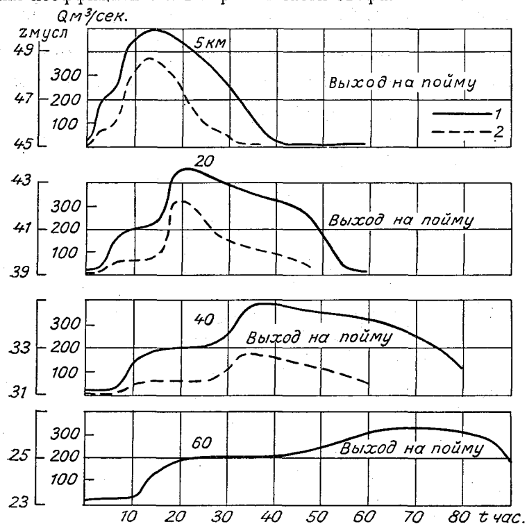
Рис. 10.26. Графики изменения во времени уровней (1) и гидрографы (2).
