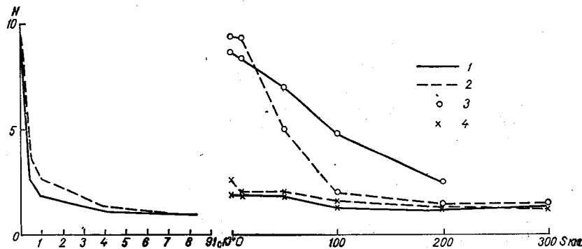
Рис. 10.19. Влияние i_0 и n на параметр N . 1 — n=0,02 ; 2 — n=0,05 ; 3 — i_0=0,00001 ; 4 — i_0=0,0001 .
