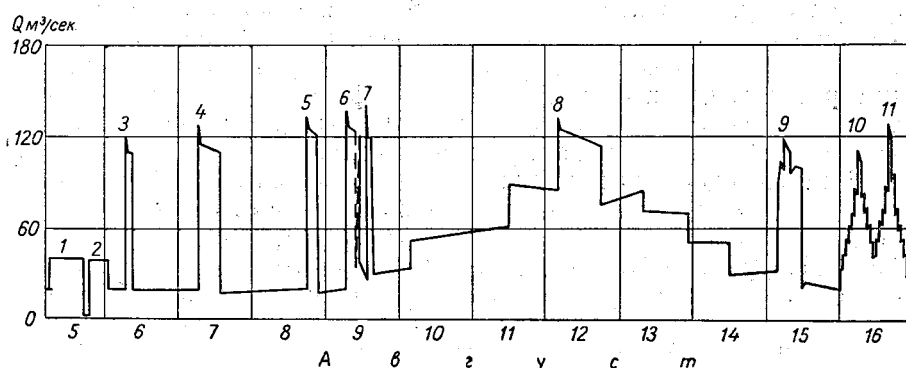
Рис. 7.4. График попусков на р. Тверце. 1—11 — номера попусков.
