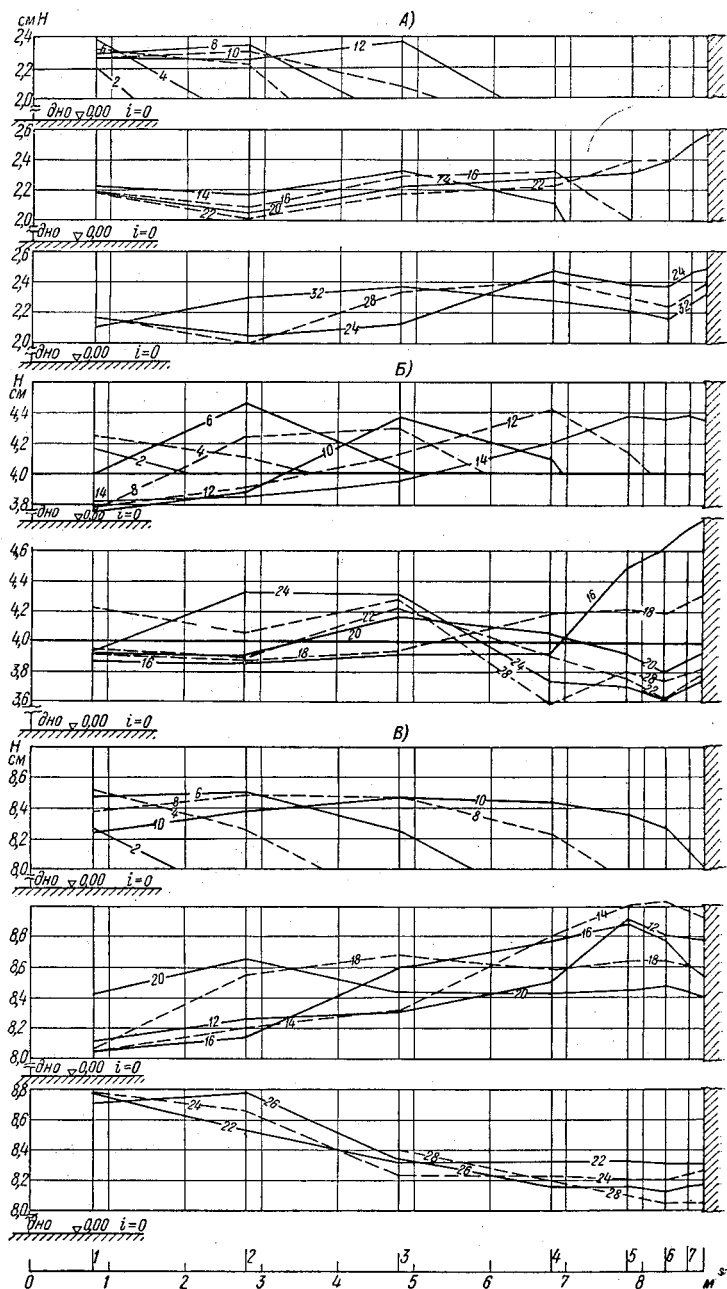
Рис. 11.4. Мгновенные профили волн в канале с горизонтальным дном.
