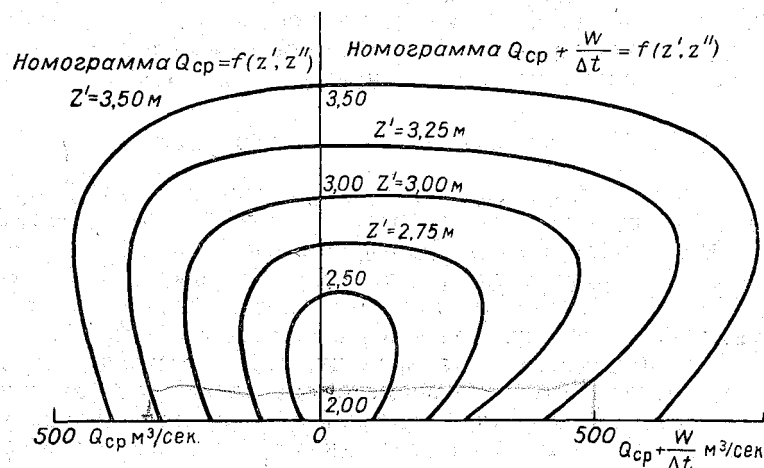
Рис. 4.4. Номограммы Я. Д. Гильденблата для метода мгновенных режимов.
