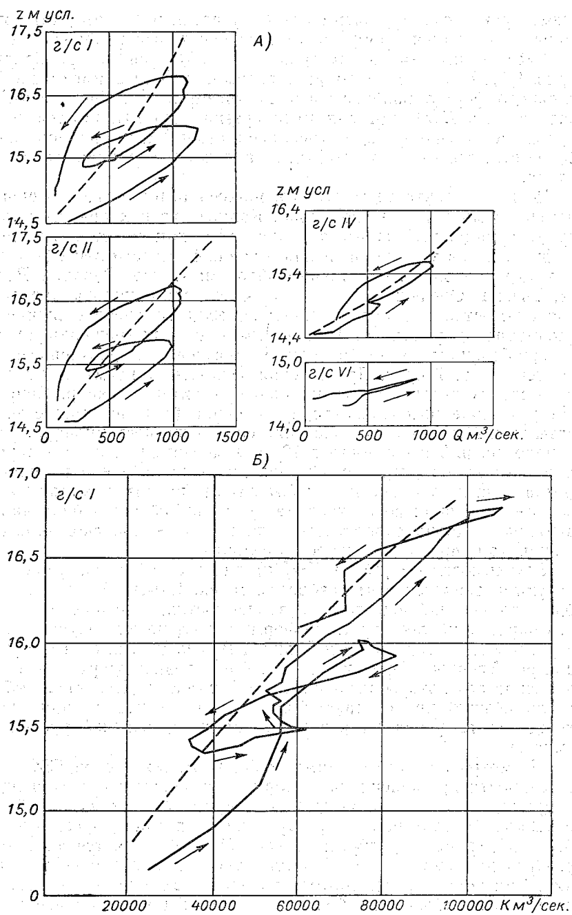
Рис. 8.5. Синхронные связи расходов (А) и модулей расходов (Б) с уровнями для р. Свири.
