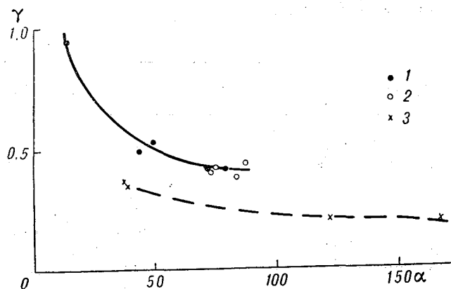
Рис. 8.7. Связь величин \alpha и \gamma (на конце экспериментального участка) для нижнего бьефа Ивановской ГЭС. 1 — лето, Q_{\max} \approx 140 м³/сек.; 2 — лето, Q_{\max} \approx 280 м³/сек.; 3 — зима, Q_{\max} \approx 130 м³/сек.
