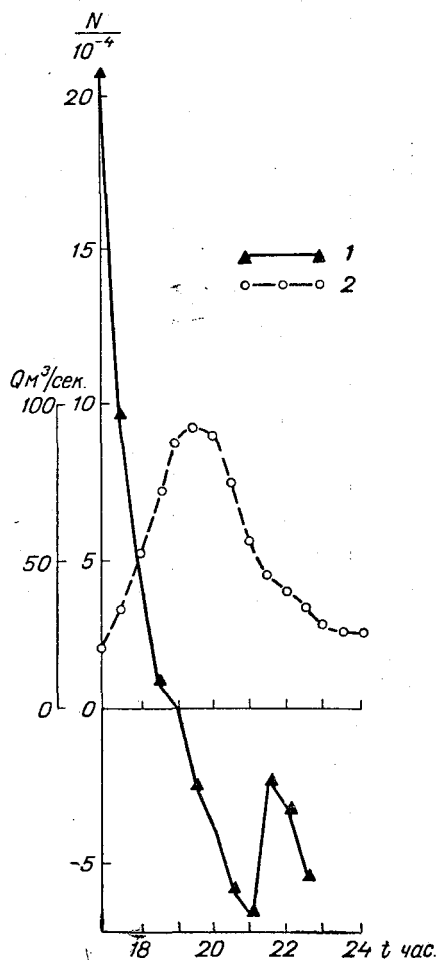
Рис. 8.1. Зависимости параметра нестационарности и расходов воды от времени для гидроствора I в нижнем бьефе Ивановской ГЭС. 1 — N=f(t) ; 2 — Q=f(t) .
