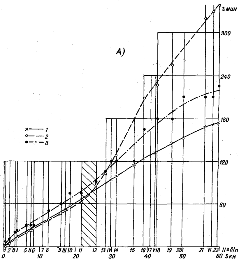
Рис. 8.20А. График времени добегания начала возмущения вдоль р. Свири. А — зима; 1 — теоретическая кривая и расчетные точки, 2 — эмпирические точки и кривые добегания по наполненному руслу, 3 — эмпирические точки и кривые добегания по опорожненному руслу.
