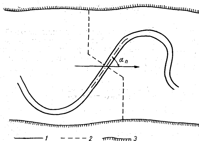
Рис. 8.19. Схема к определению угла пересечения руслового и пойменного потоков.
