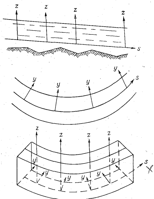
Рис. 1.1. Координатная система русла.
