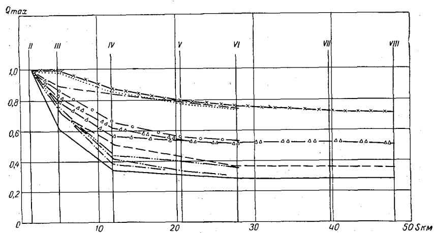
Рис. 8.9. Снижение Q_{max} и изменение c_T вдоль р. Тверцы.
