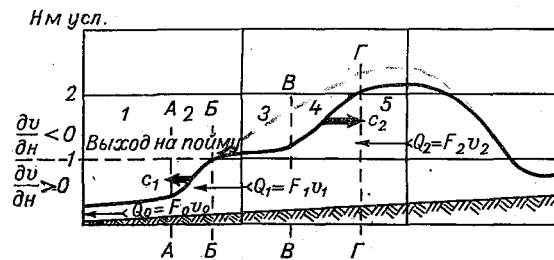
Рис. 12.2. Схематический профиль волны в русле с поймой.
