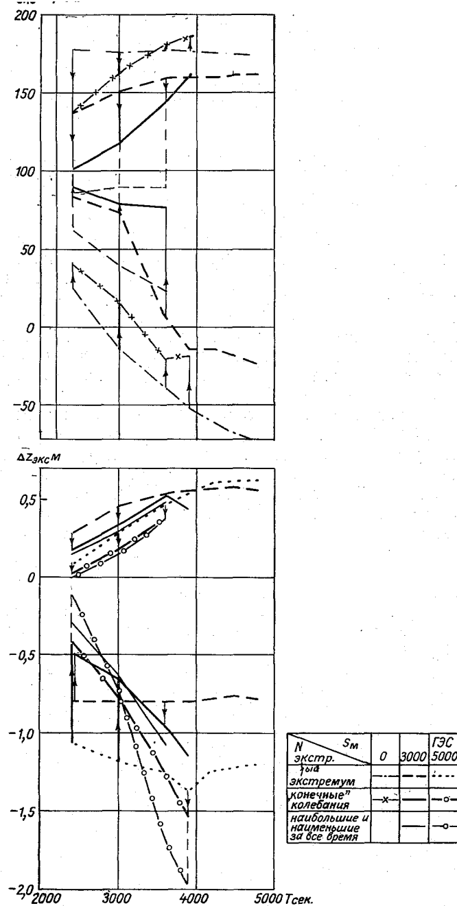
Рис. 10.9. Экстремальные значения Q и \Delta z для первого, наиболее резкого и конечного колебаний в функции от T (задача 1 г).
