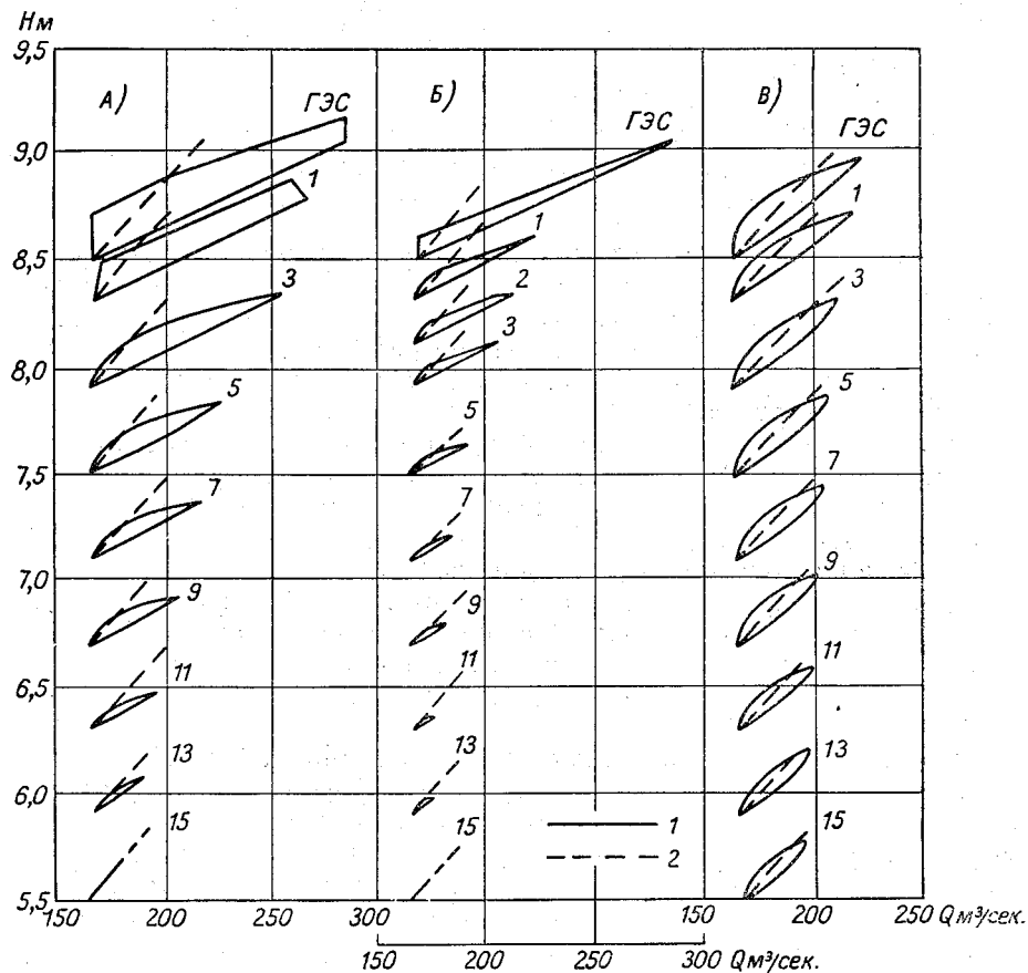
Рис. 10.16. Трансформация петель попусков по длине канала.
