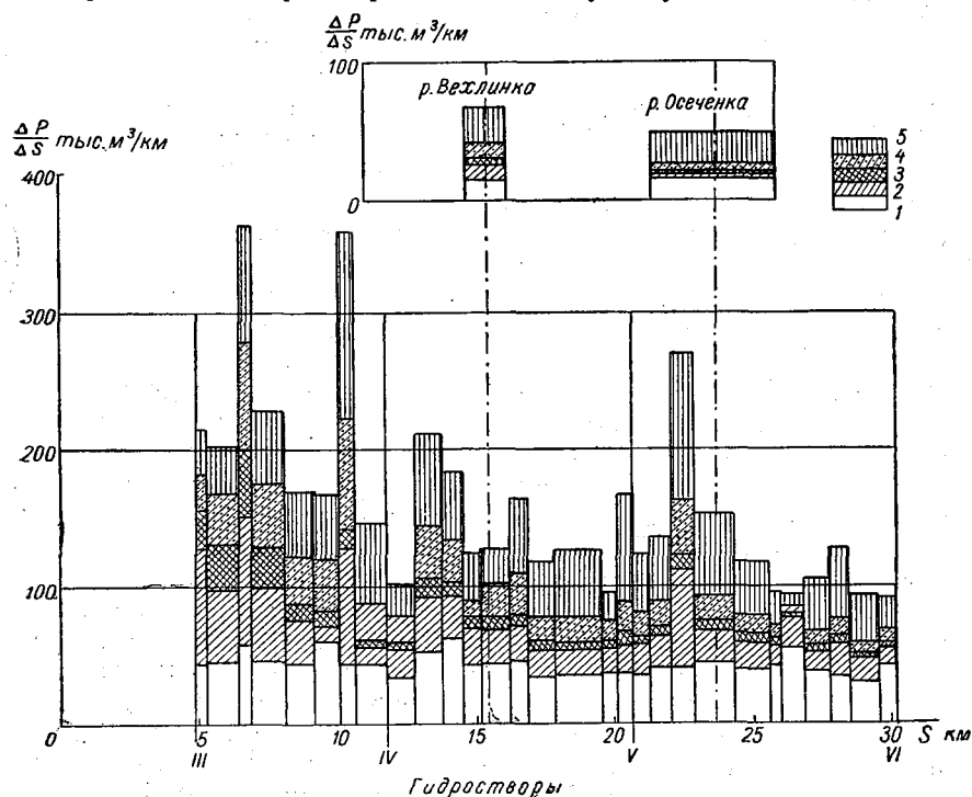
Рис. 8.12. Объемы затопления участков русла и поймы между гидропостами III и VI на р. Тверце.
