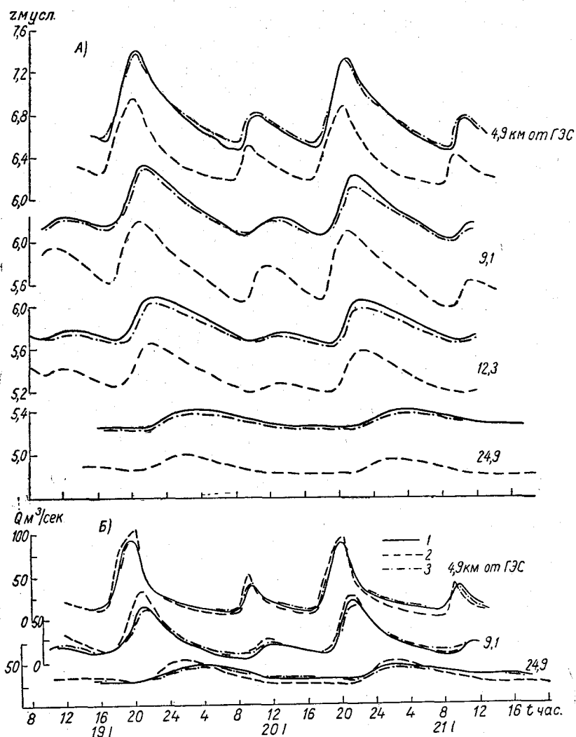
Рис. 9.4. Графики хода уровней (А) и расходов воды (Б) для Верхней Волги в зимних условиях.
