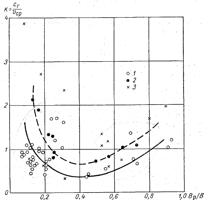
Рис. 8.14. Зависимость k от отношения ширины русла к суммарной ширине русла и поймы. 1 — р. Иртыш; 2 — р. Тверца; 3 — данные Г. В. Железнякова.
