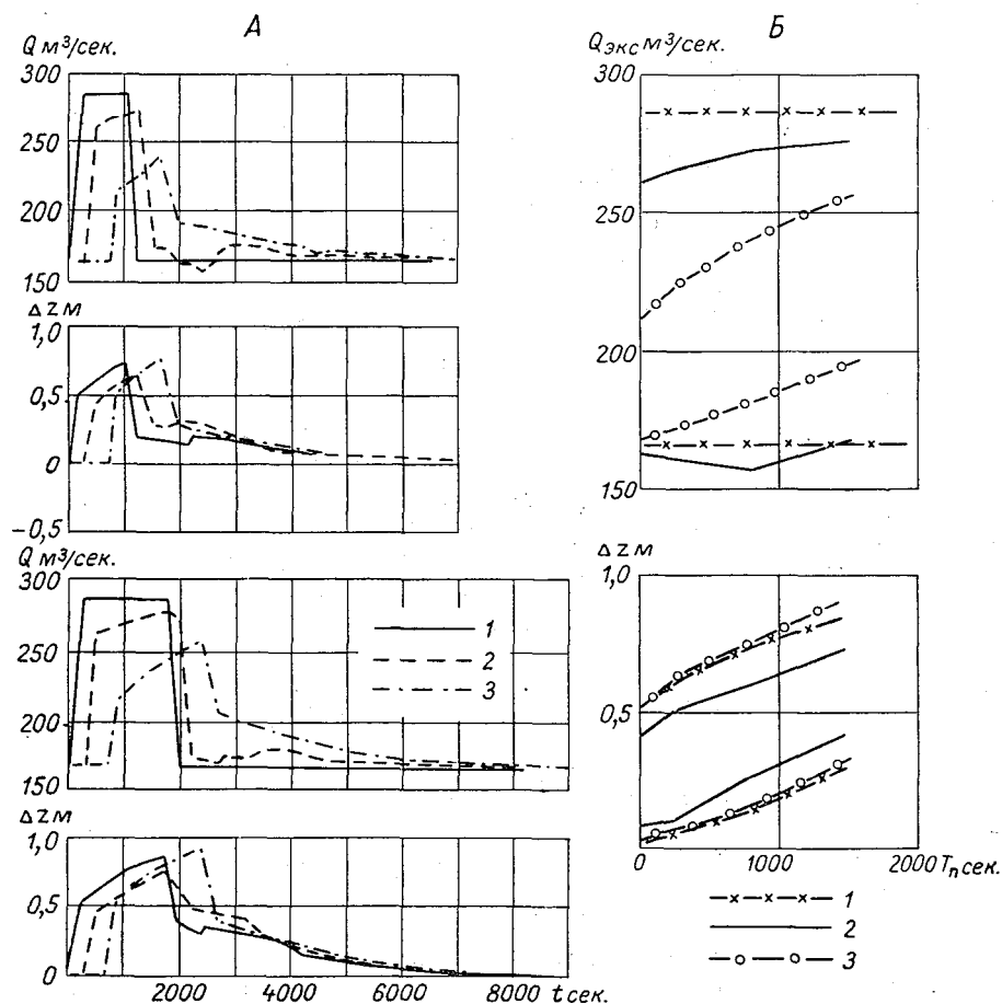
Рис. 10.6. А — изменение во времени расходов и уровней для задачи 4б ( T_n = 800 сек. и T_n = 1500 сек.); Б — экстремальные значения расходов и отклонений уровня для первого колебания в функции от T_n . 1 — s=0 , 2 — s=2000 м, 3 — s=5000 м.
