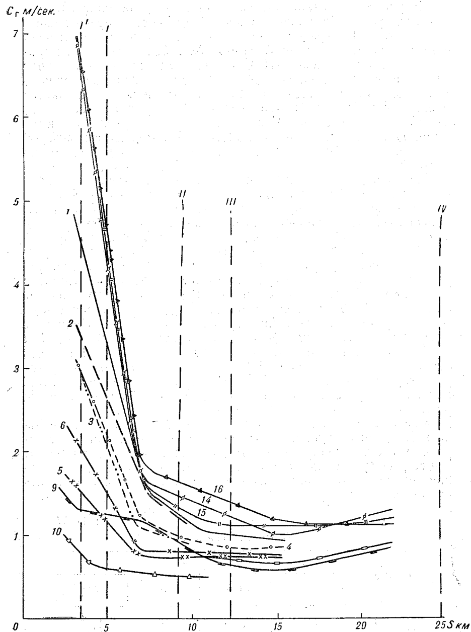
Рис. 8.8. Изменение c_T вдоль нижнего бьефа Ивановской ГЭС. Цифры у линий — номера пусков.
