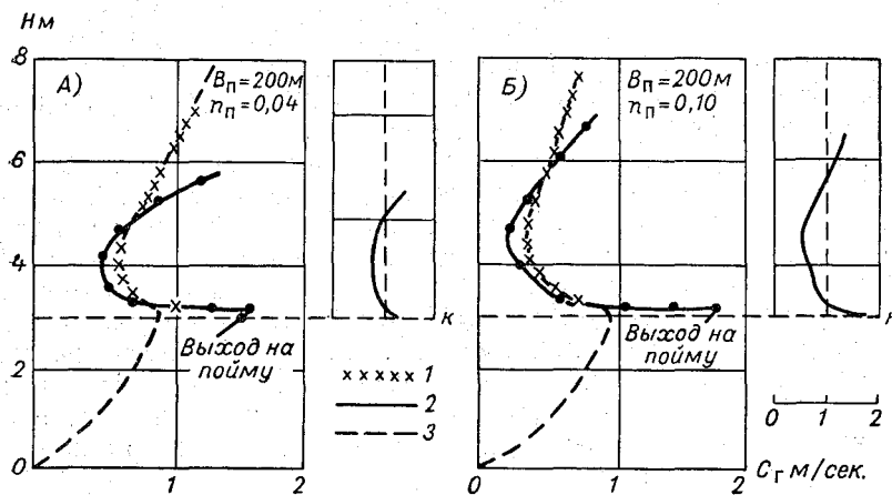
Рис. 10.24. Зависимости c_T и k от H при различной шероховатости поймы.
