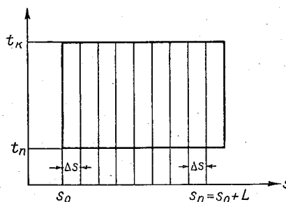
Рис. 4.7. Метод прямых.
