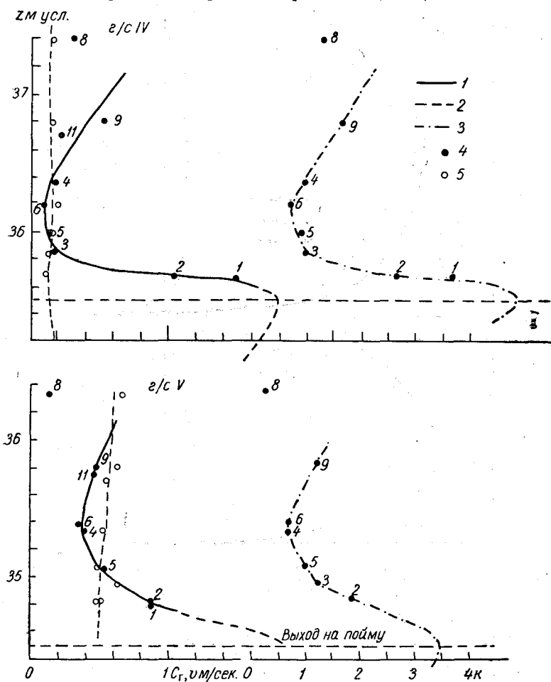
Рис. 10.22. Зависимости c_T и v от H для р. Тверцы. 1 — c_T , 2 — v , 3 — k , 4 — точки для c_T и k (числа у точек — номера попусков), 5 — точки для v .
