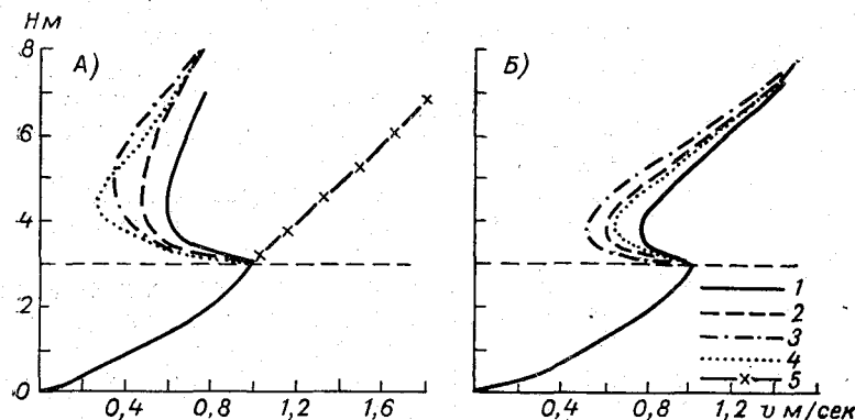
Рис. 10.23. Графики v=v(H) .
