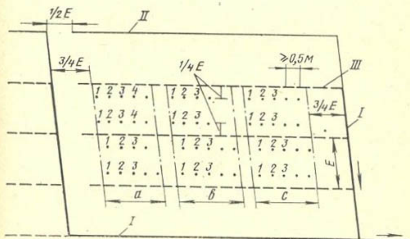
Рис. 1. Опытная дренажная система для исследования почвенной влажности:
