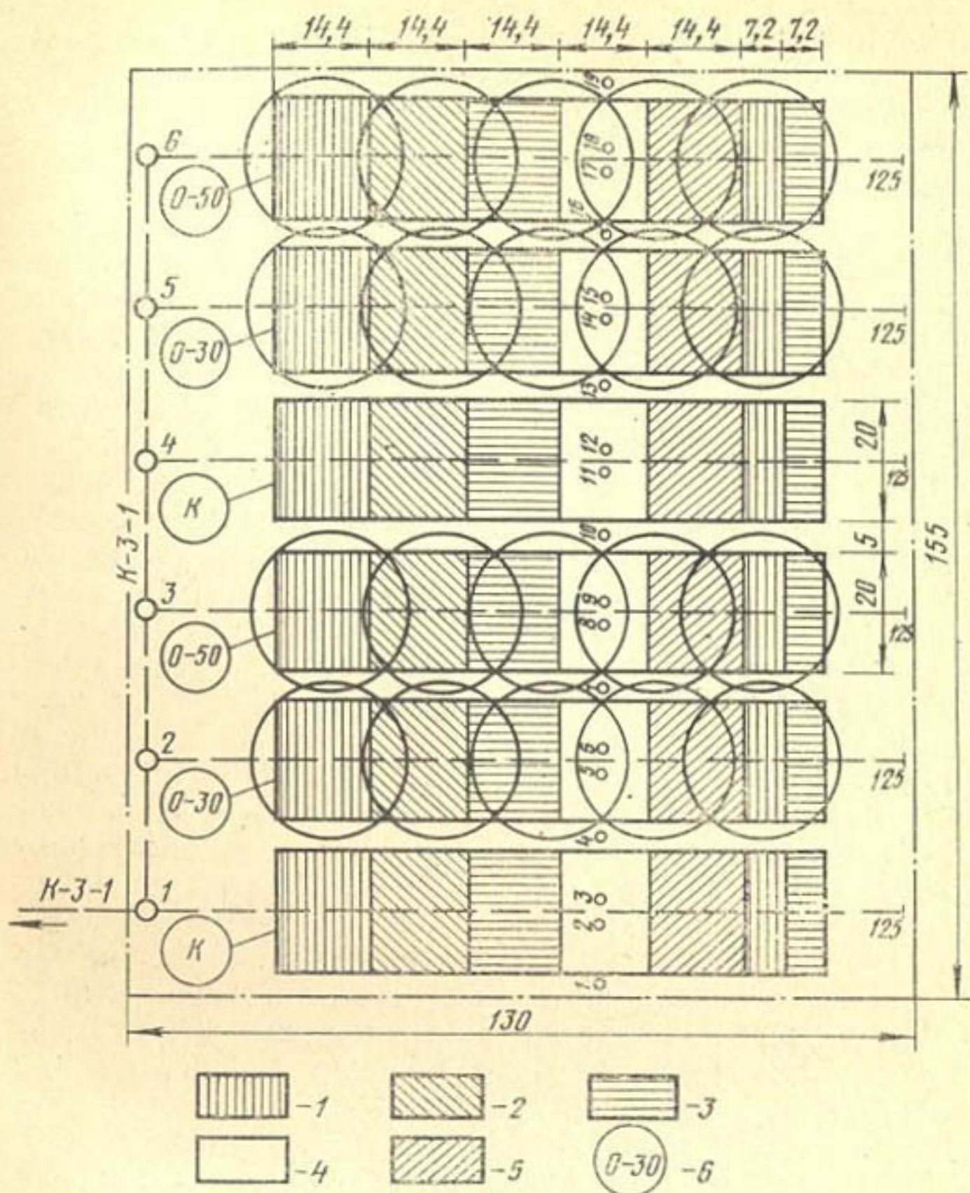
Рис. 3. Схема опытного участка «Грасенки»: 1 — ежа сборная; 2 — костер безостый; 3 — овсяница.
