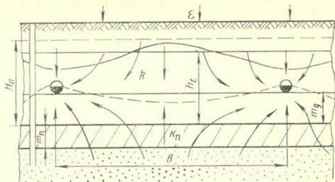
Рис. 1. Схема к расчету динамики уровня грунтовых вод при одновременном напорном и инфильтрационном питании: l — дрена.
