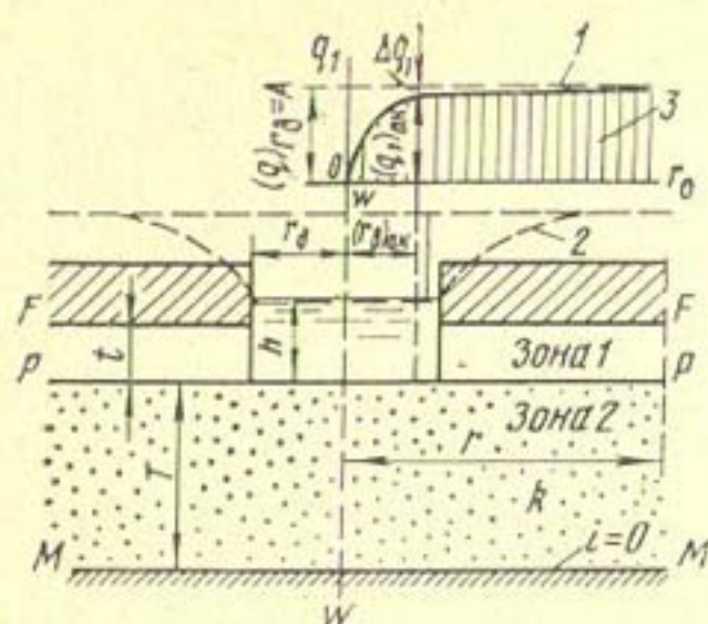
Рис. 11. Изменение расхода q_1 в зависимости от радиуса колодца r_0 : 1 — асимптота; 2 — кривая напоров; 3 — эпюра q_1 = f(r_0) .
