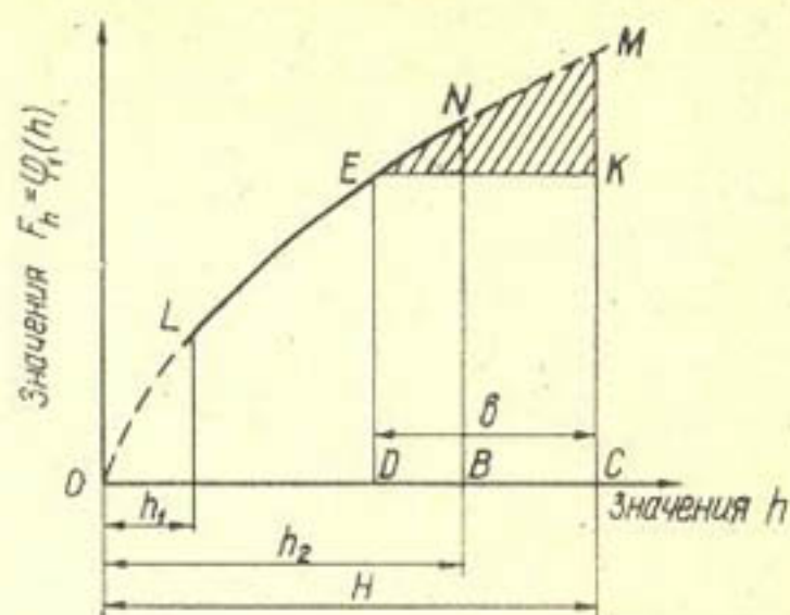
Рис. 2. Определение потенциала H . К. Гиринского в зависимости от положения водоупора.
