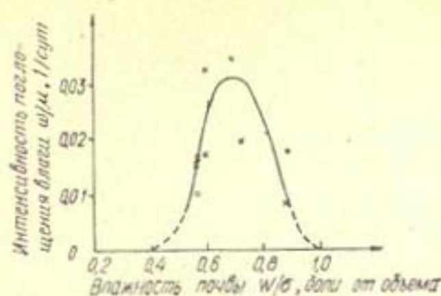
Рис. 7. Зависимость интенсивности поглощения влаги корнями растений \omega/\mu от влажности почвы \omega .
