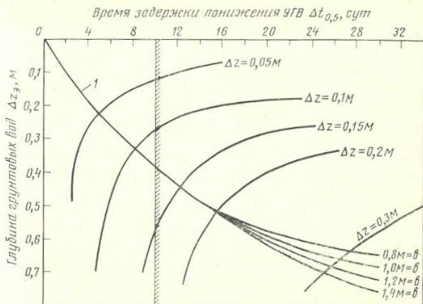
Рис. 1. Ход понижения уровня грунтовых вод в середине между дренами при расчетном режиме и зависимость \Delta z = f(z_0, \Delta t_{0,5}) :
