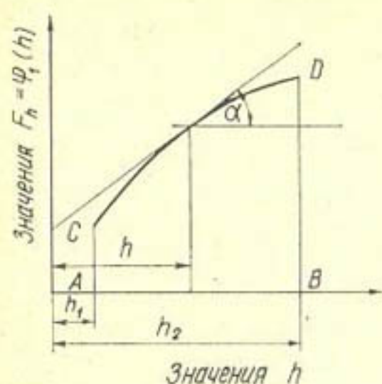
Рис. 1. Определение точечного значения k .
