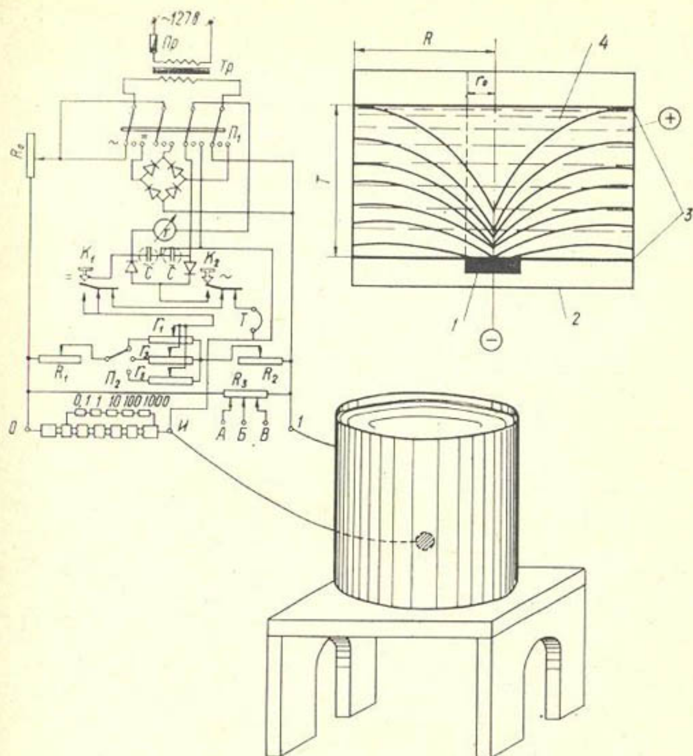
Рис. 4. Схема (а) и вертикальное сечение модели (б) опыта по определению расхода q_1 методом ЭГДА:
