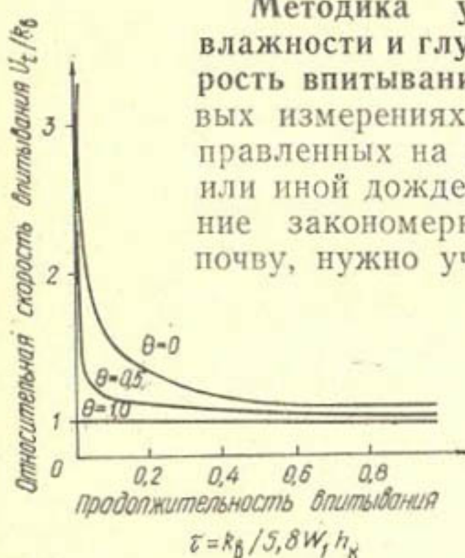
Рис. 8. Изменение динамики впитывания в зависимости от начальной влажности \omega_n :
