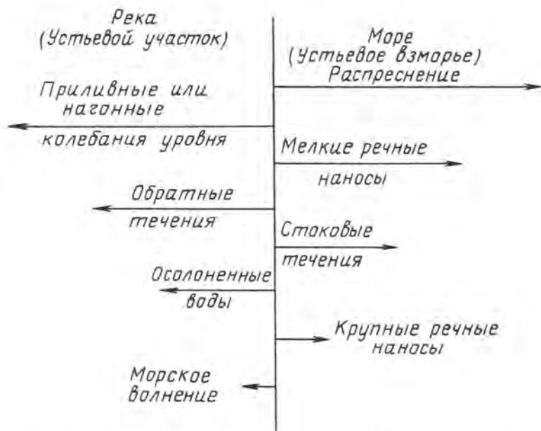
Рис. 1.10. Схема взаимодействия реки и моря в устьевой области реки
