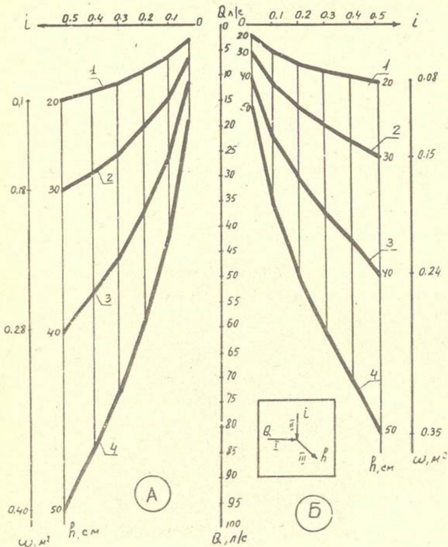
Рис. 3.15. Номограмма для гидравлического расчета водосборной канавки с гравийной засыпкой: А - при b = 20 см; Б - b = 0,30 м; 1 - при H_g = 20 см; 2 - H_g = 0,30 м; 4 - H_g = 50 см.
