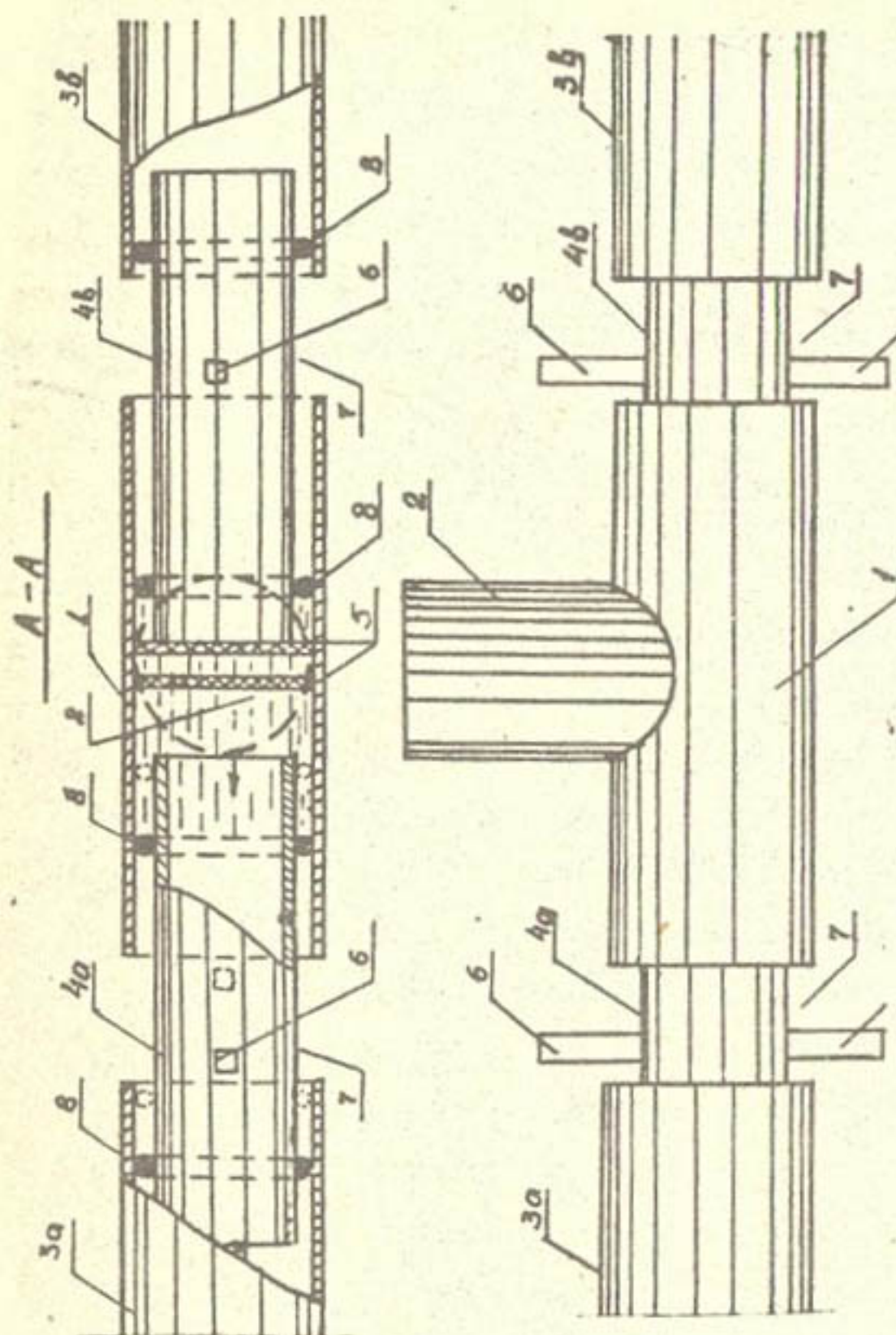
Рис. 3.21. Запорное устройство для подачи воды из трубчатой сети в поливные трубопроводы.
