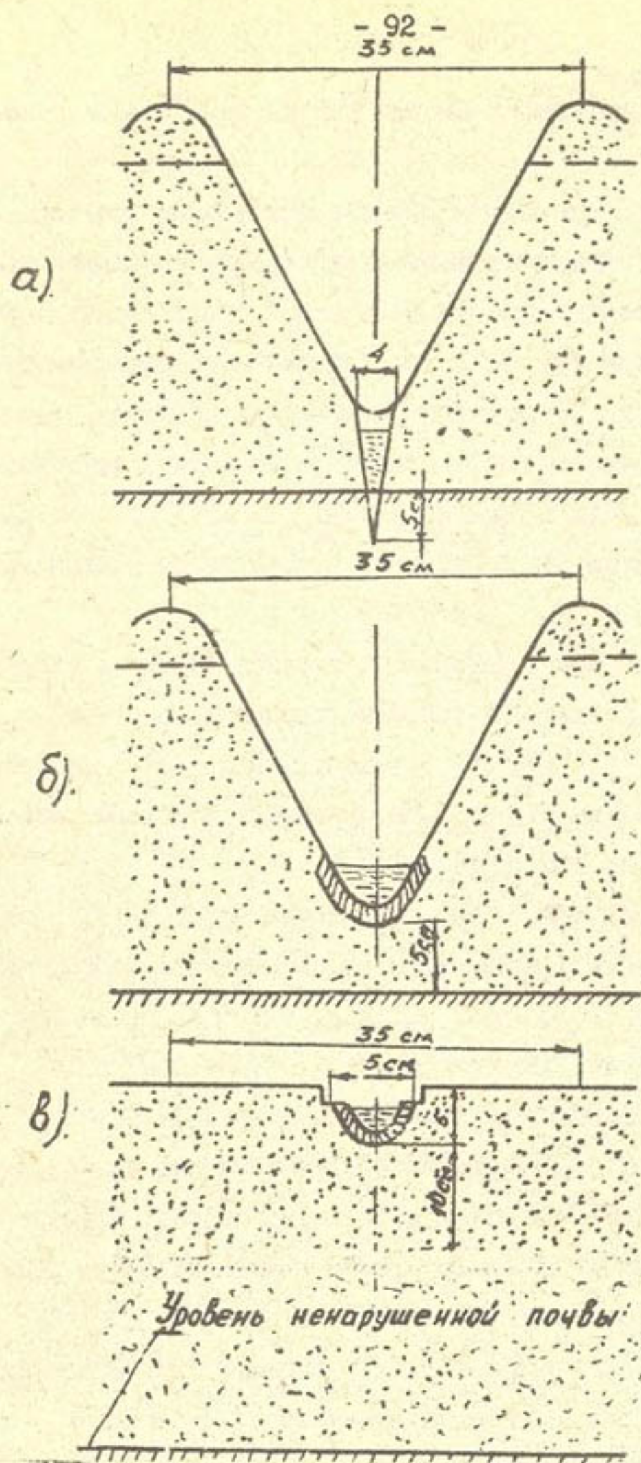
Рис. 2.3. Поперечное сечение поливных борозд: а - обычная, нарезанная окучником НО-27А; б - обычная с прикатанным дном; в - микроборозда, вдавленная катками.
