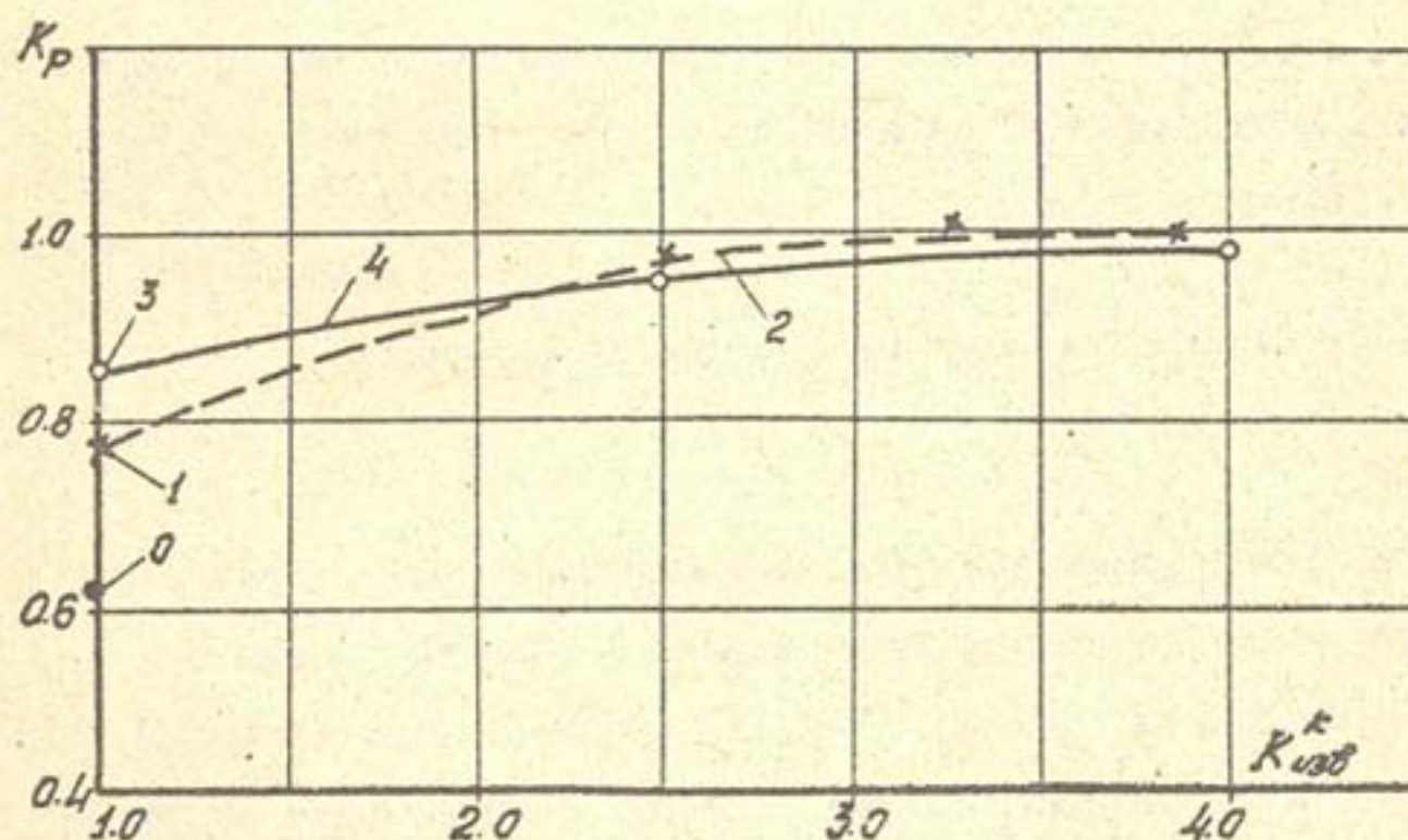
Рис. 2.14. Зависимость K_p = \varphi(K_{изб}^K) 0 - обычная борозда, 1 - прямолинейная микроборозда; 2 - зигзагообразная микроборозда (данные полевых экспериментов); 3 - прямолинейная микроборозда; 4 - зигзагообразная микроборозда (расчет на ЭВМ по методике АФИ).
