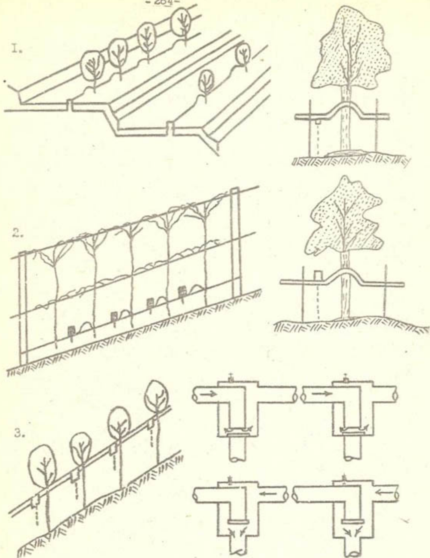
Рис. 4.2 Низконапорные капельные системы: 1 - Таджикистан-I (непрерывная); 2 - Таджикистан-Im (импульсная); 3 - Таджикистан-2 (импульсная).
