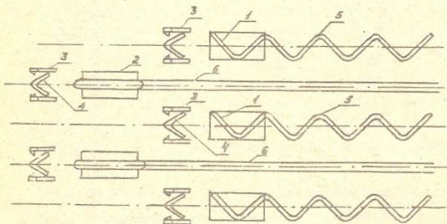
Рис. 2.19. Схема установки катков-бороздоделов КБ-I на культиваторе Крх-4. 1 - катки с извилистыми выступами; 2 - то же с прямолинейными выступами; 3 - комплект культивирующих органов; 4 - стрелчатые лапки; 5 - извилистые микроборозды на междурядьях, где проходят колеса трактора; 6 - прямолинейные микроборозды, где не проходят колеса трактора.
