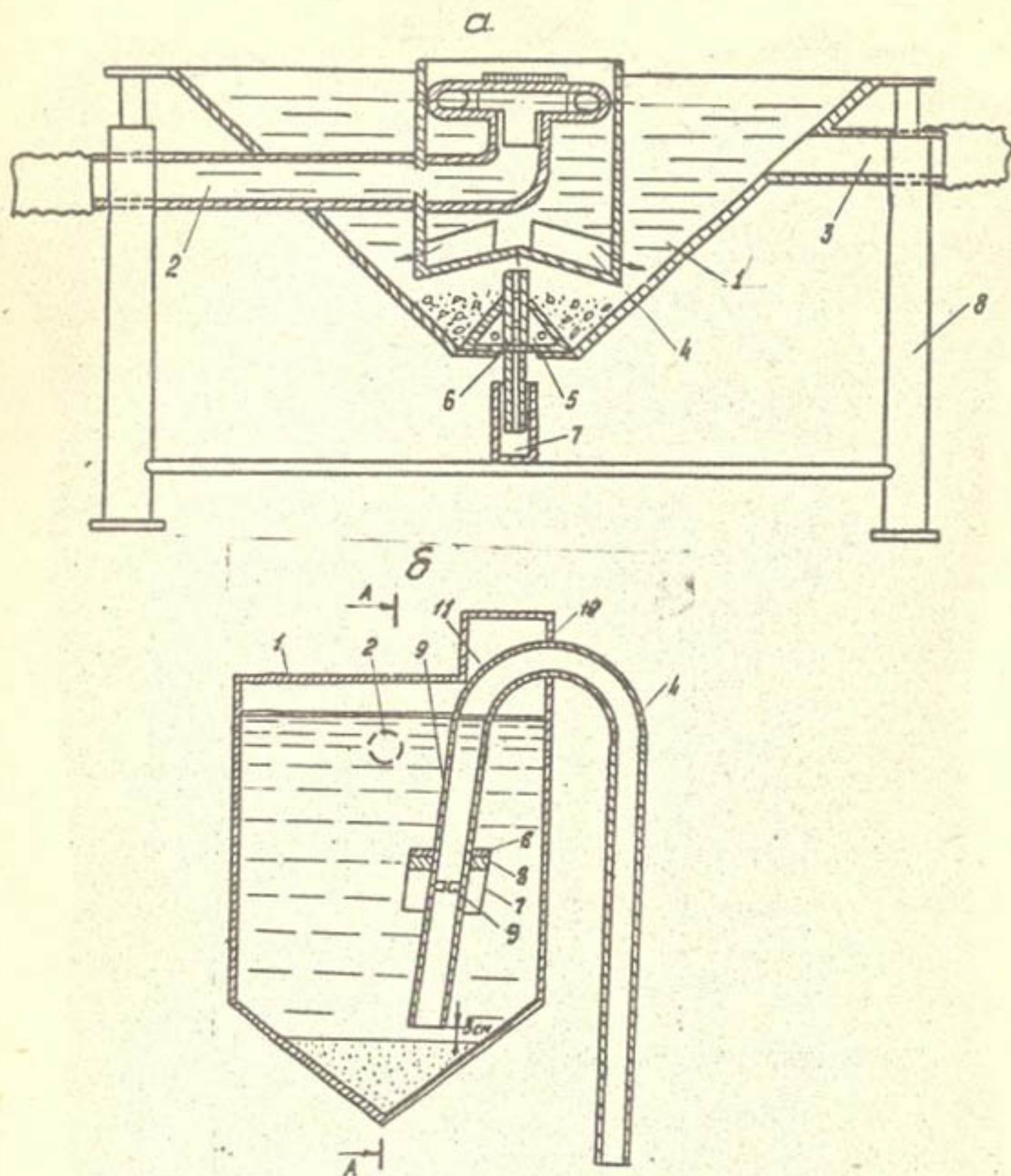
Рис. 4.4. Отстойники-автоматы:
