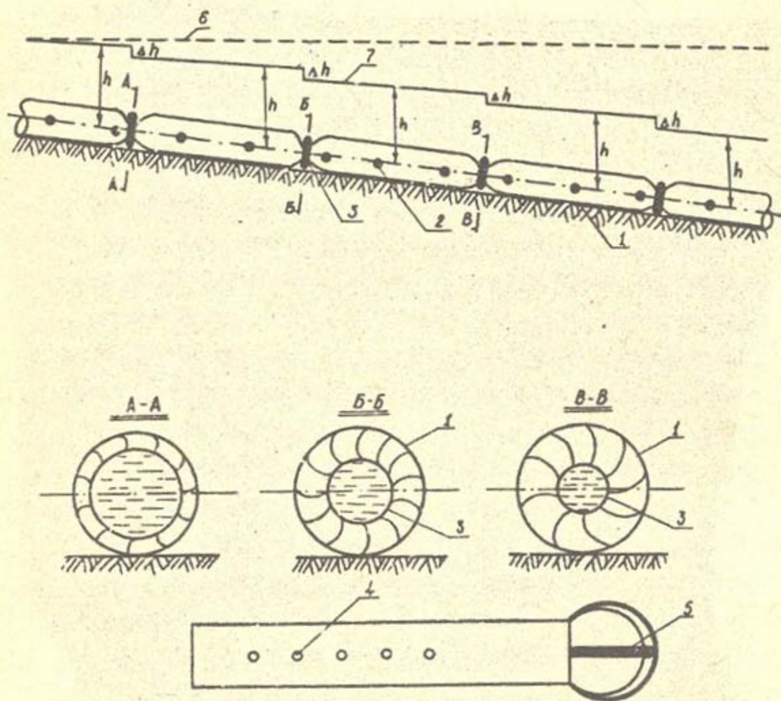
Рис. 3.6. Поливной планг с напорорегулирующими кольцами: 1 - поливной планг, 2 - поливные отверстия; 3 - напорорегулирующие кольца; 4 - отверстия; 5 - выступ для регулировки размера кольца; 6 - статический горизонт; 7 - пьезометрическая линия напора; h - напор; \Delta h - потери напора.
