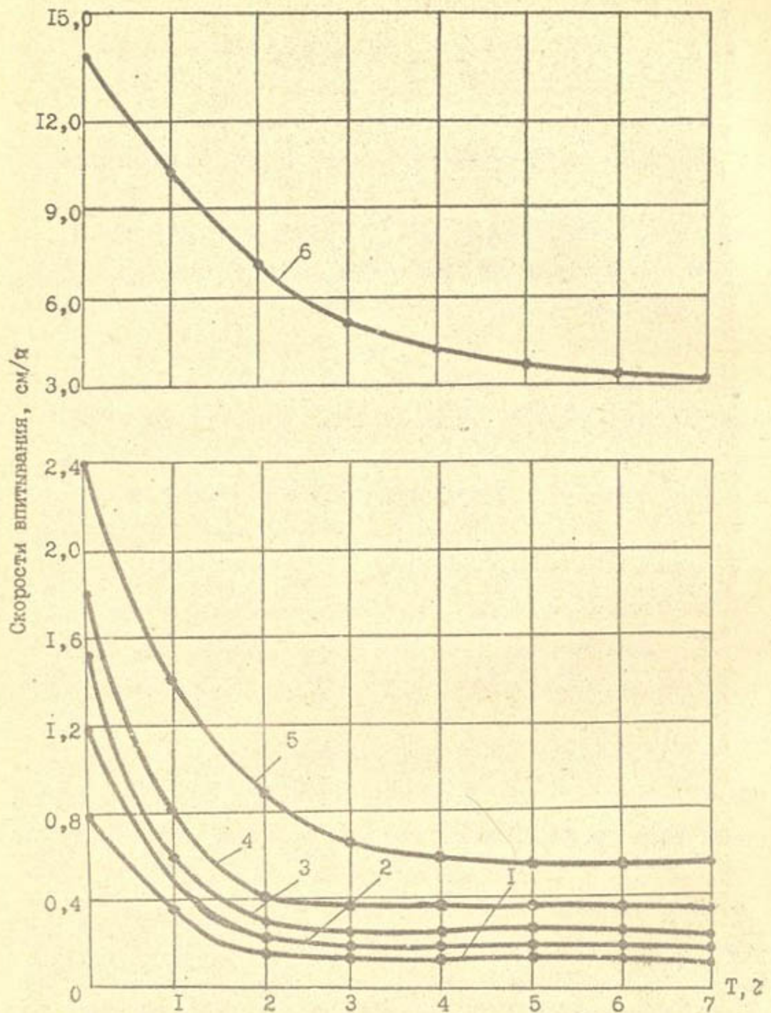
Рис. 1.3 Скорости впитывания воды на различных типах почв Таджикской ССР. 1 - коричневые карбонатные; 2 - обыкновенные сероземы; 3 - светлые сероземы; 4 - темные сероземы; 5 - типичные сероземы; 6 - серобурые каменистые.
