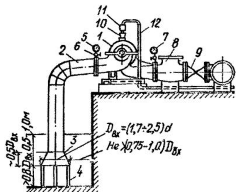
Рис. 5.4. Схема оборудования арматурой горизонтального центробежного насоса
