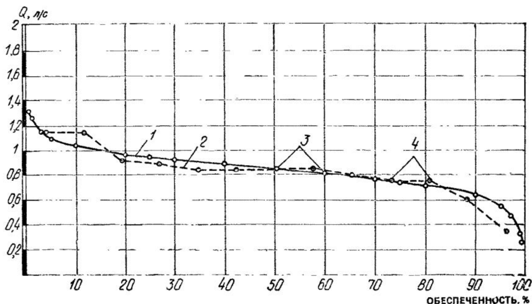
Рис. 11.5. Кривая обеспеченности минимальных дебитов источника 1 — кривая обеспеченности по функциям Шарлье; 2 — кривая обеспеченности по фактическим точкам; 3 — точки вычисления по функциям Шарлье; 4 — точки по фактическим данным
