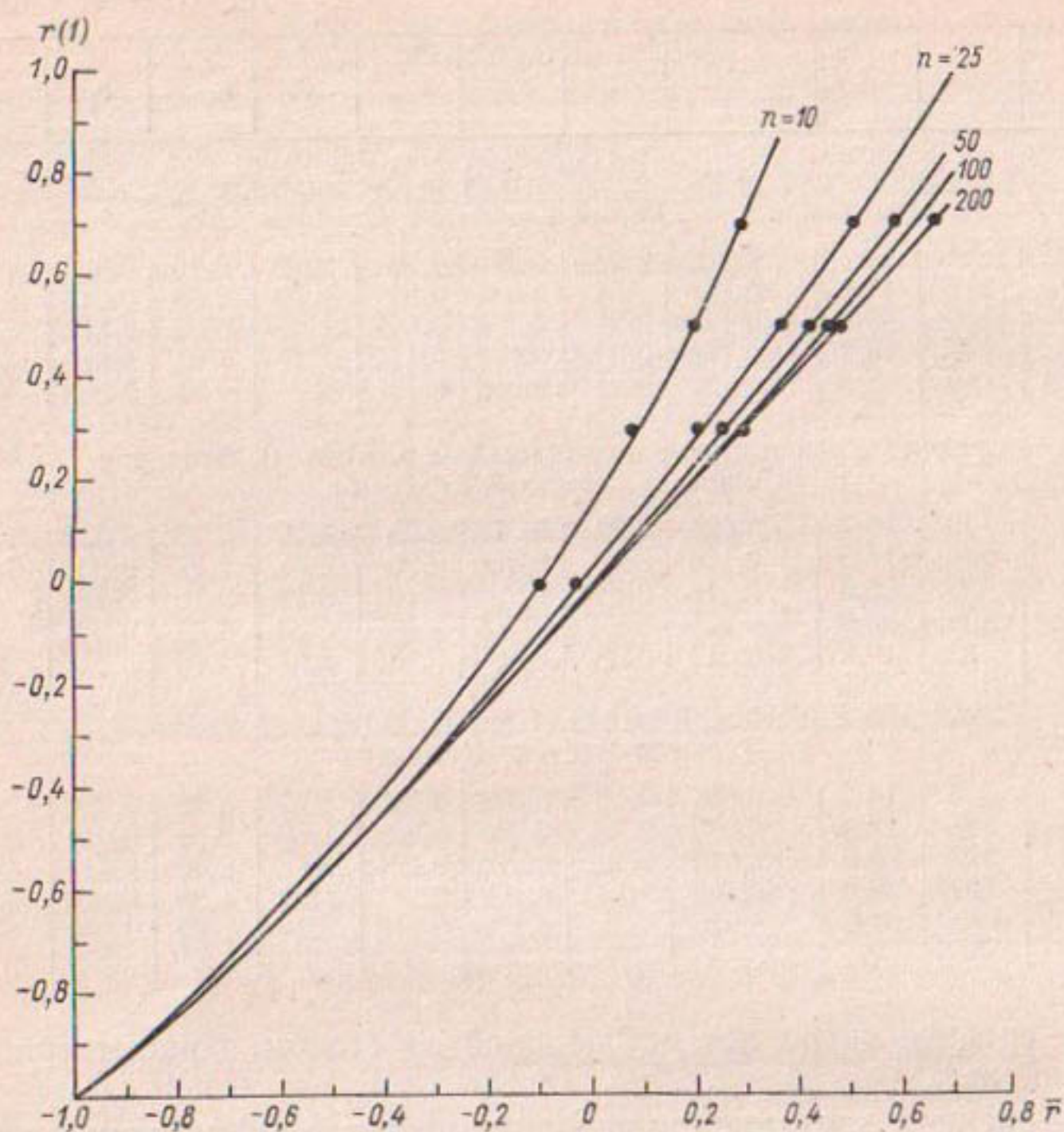
Рис. 2.10. Зависимость r(1)=f(\bar{r}) .
