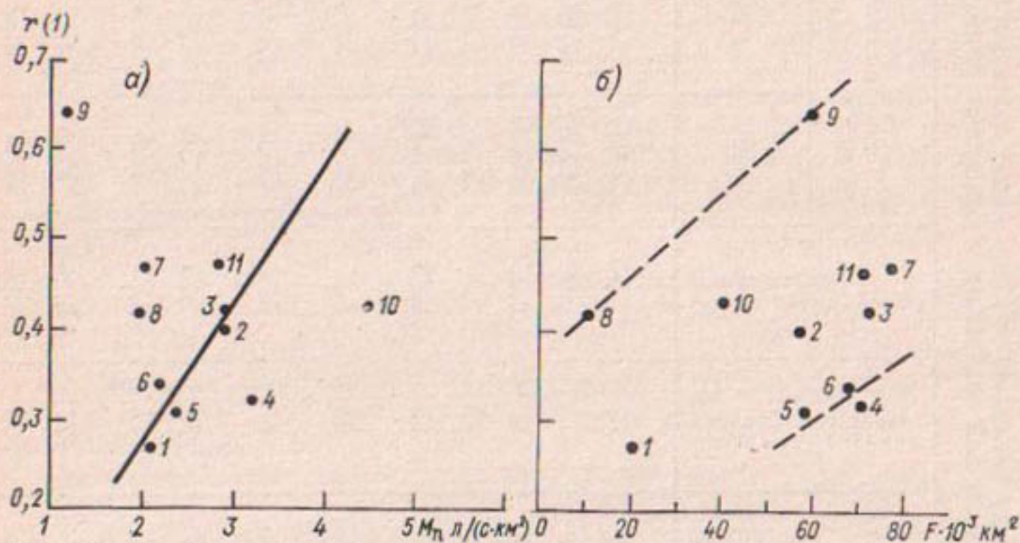
Рис. 5.7. Зависимость коэффициентов корреляции между подземным стоком смежных лет r(1) от модуля подземного стока (а) и площади водосбора (б). Цифры у точек — номера районов по табл. 5.16.
