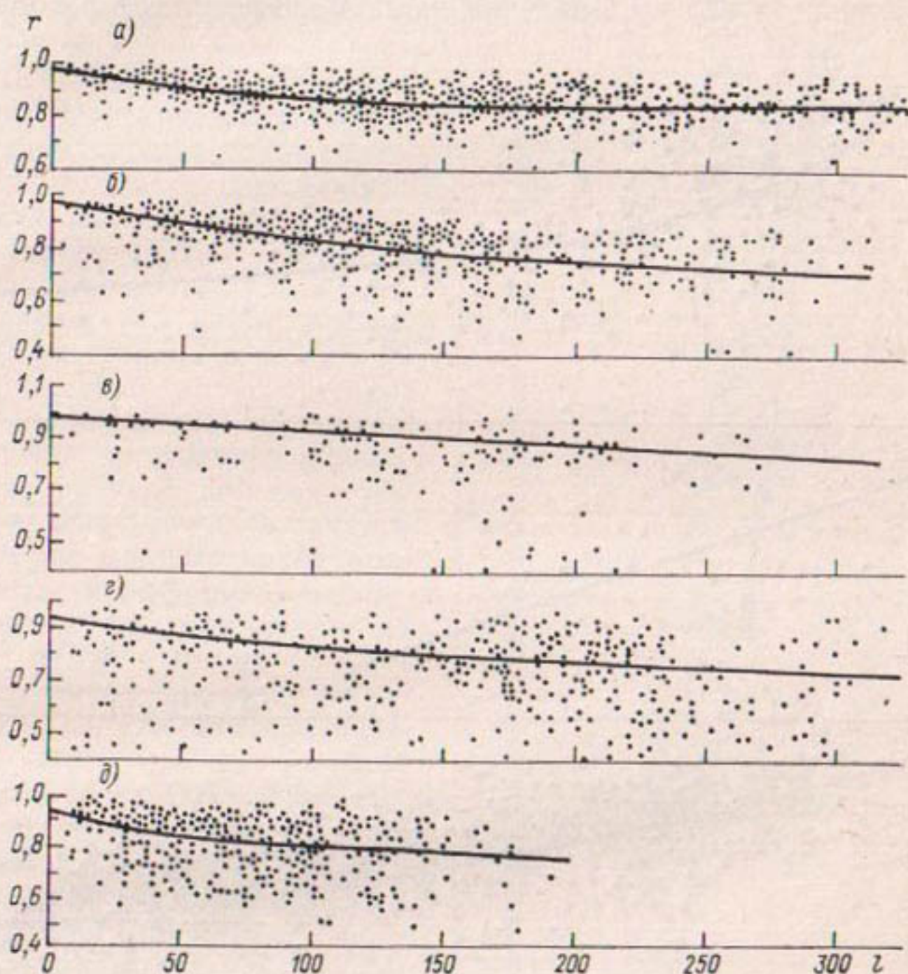
Рис. 2.27. Пространственная корреляционная функция годового стока рек бассейна Волхова (левобережье), бассейна р. Луги, р. Нарвы, озер Чудского и Ильмень (а), бассейна Волхова (правобережье) и бассейна рек Сясь, Паши, Оять (б), бассейна рек Ловать, Полы, Великой и оз. Ильмень (в), бассейнов рек между Финским заливом и Ладожским озером, Ладожским и Онежским озером и бассейна р. Свири (г) и рек Северо-Запада ЕТС, впадающих в Белое море (д).
