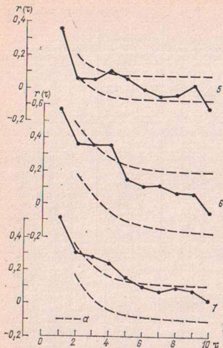
Рис. 5.6. Автокорреляционные функции для различных совокупностей временных рядов подземного стока.
