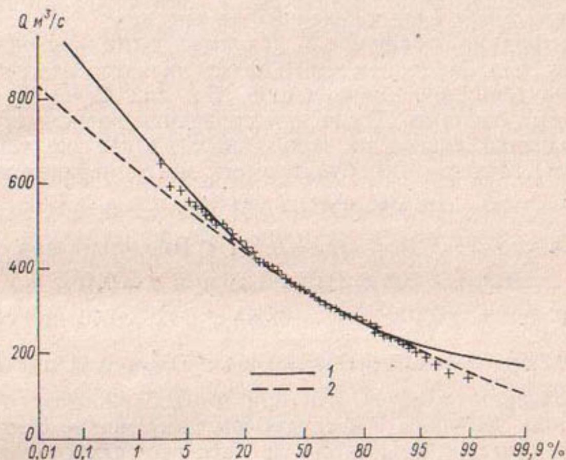
Рис. 1.6. Эмпирическое распределение максимальных расходов воды на р. Онеге у д. Надпорожский Погост и его аналитическая аппроксимация распределением Пирсона III типа.
