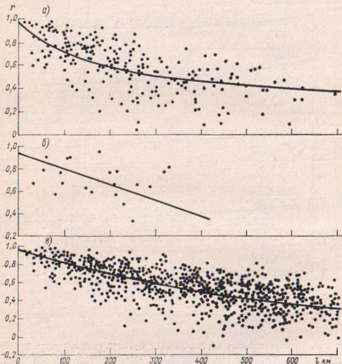
Рис. 2.28. Пространственная корреляционная функция годового стока бассейна р. Печоры (а), бассейна р. Усы (б) и бассейна р. Онеги (в).
