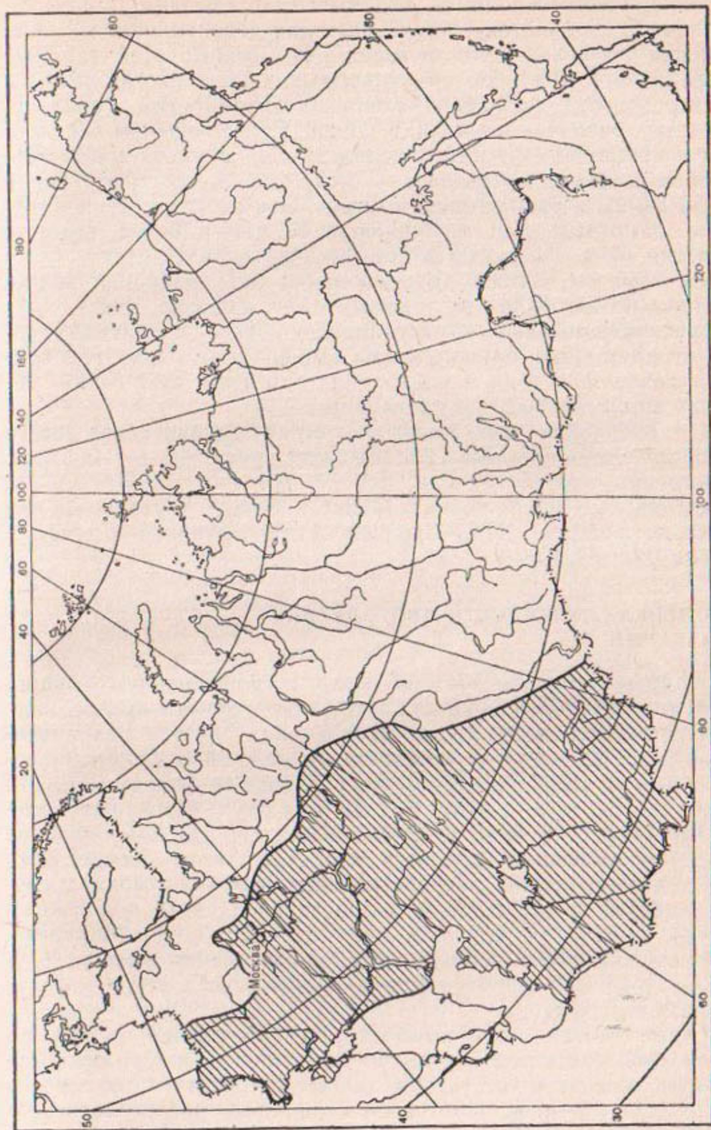
Рис. 3.1. Районы со средней длительностью группировок более 2,7 лет в колебаниях наименьших расходов воды.
