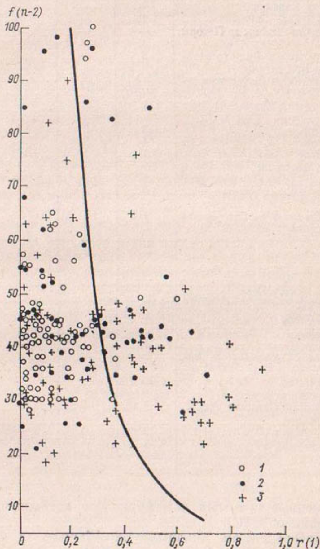
Рис. 4.8. Зависимость r(1)=f(n-2) при \alpha=5\% .
