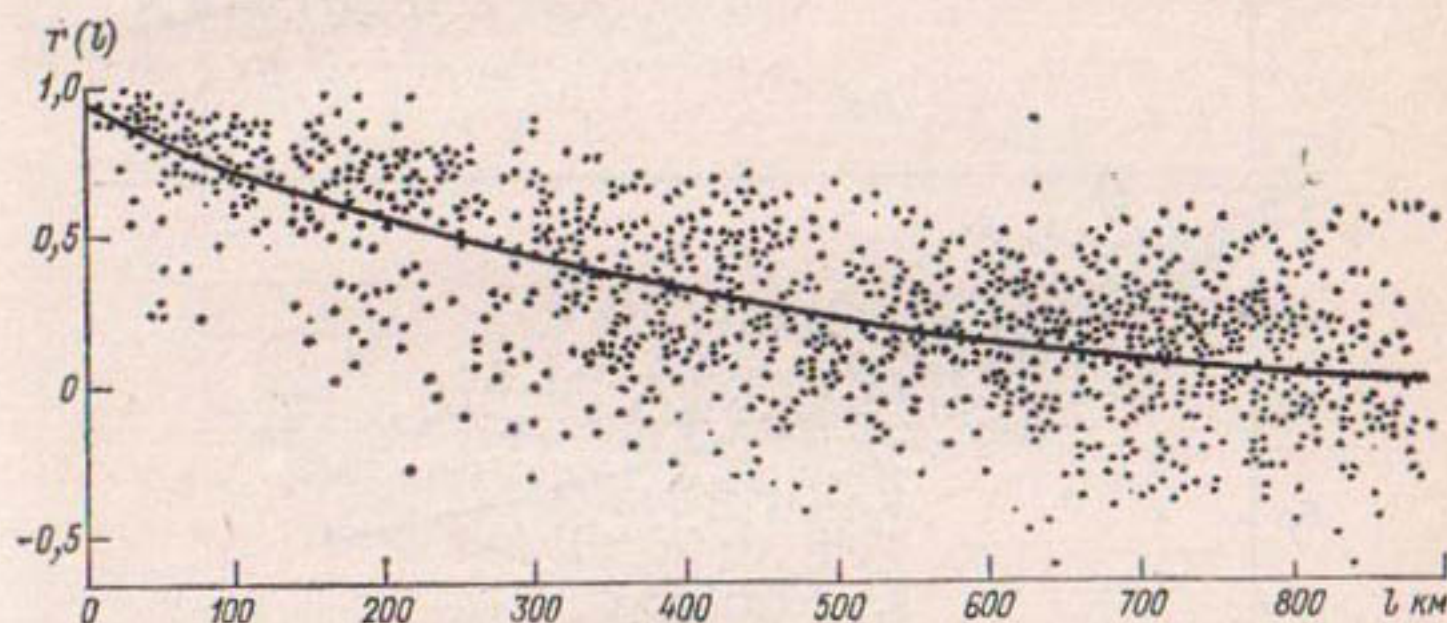
Рис. 2.31. Обобщенная пространственная корреляционная функция годового стока рек бассейна Днепра.
