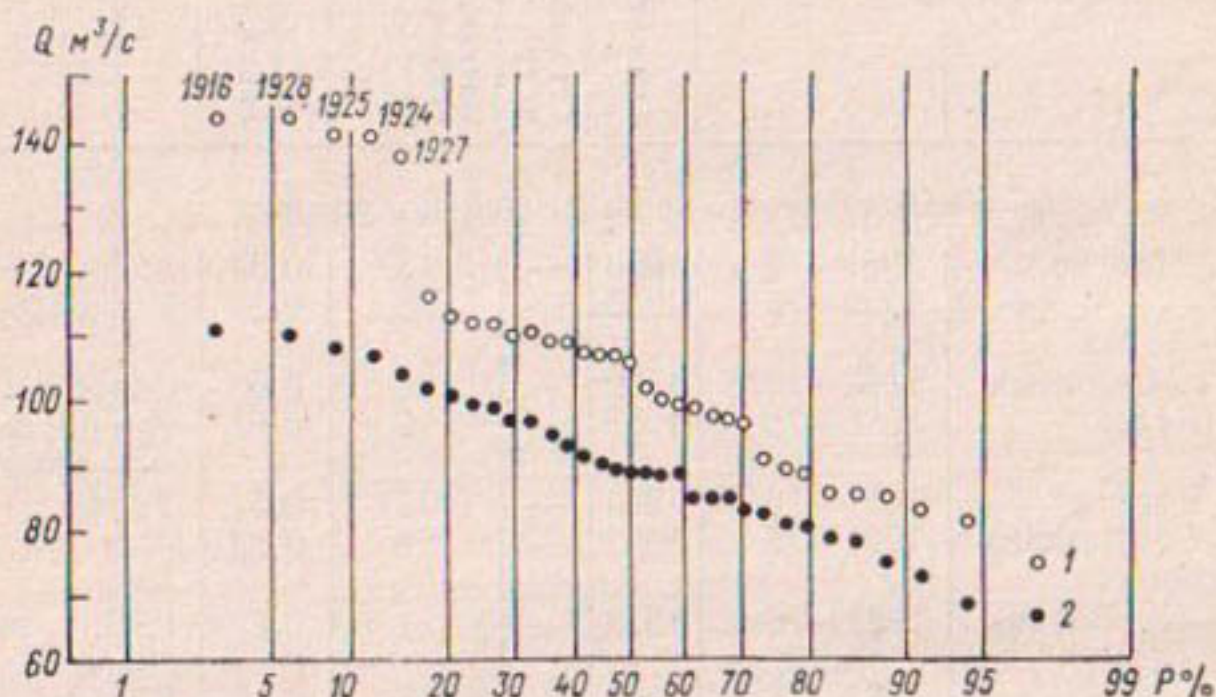
Рис. 5.12. Эмпирические кривые обеспеченности подземного стока за полупериоды наблюдений 1902—1934 (1) и 1935—1967 гг. (2) для нестационарного по дисперсии и среднему временного ряда р. Вишера — д. Митракова.
