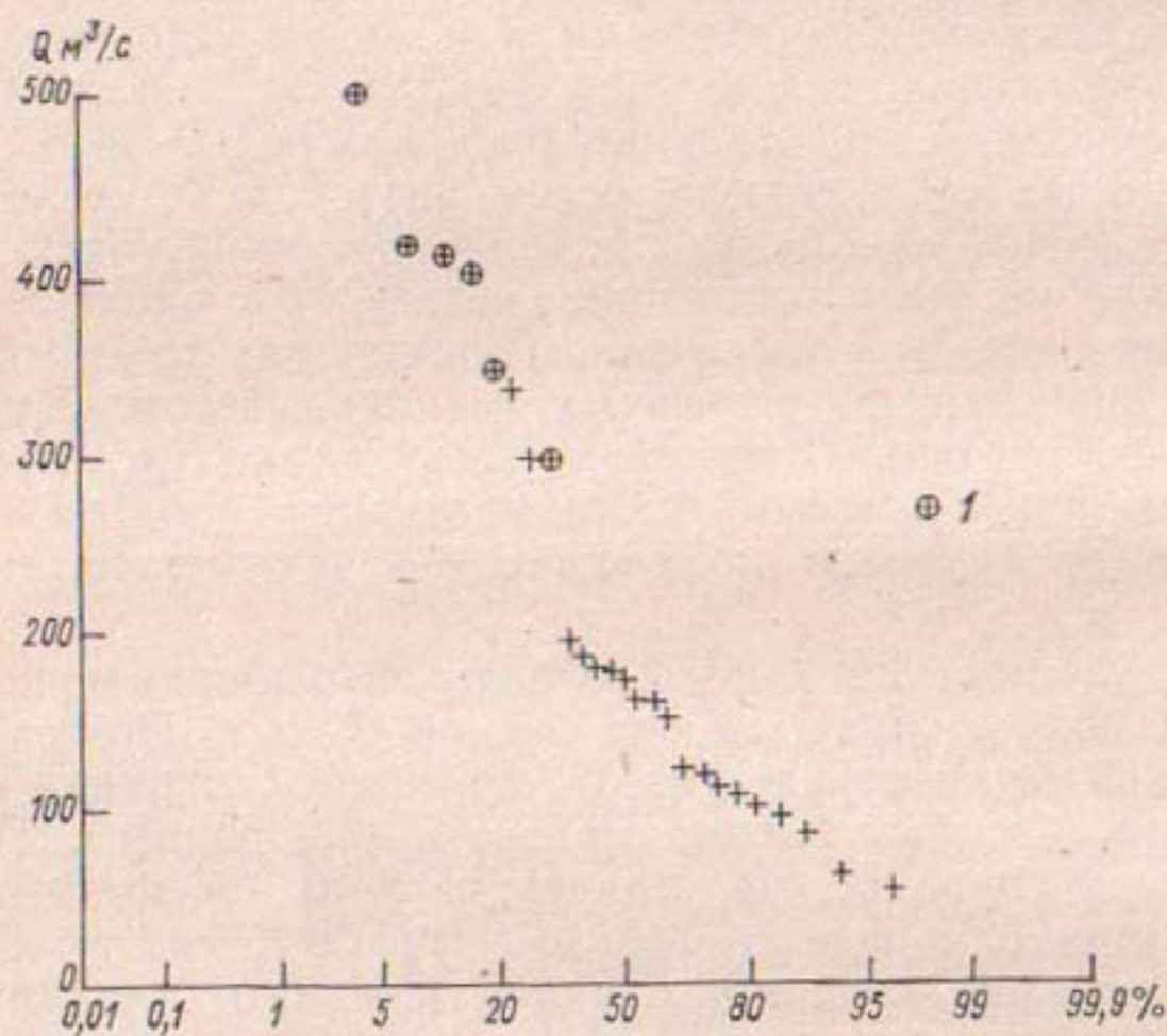
Рис. 1.7. Эмпирическое распределение максимальных расходов воды на р. Остер у с. Ходунь.
