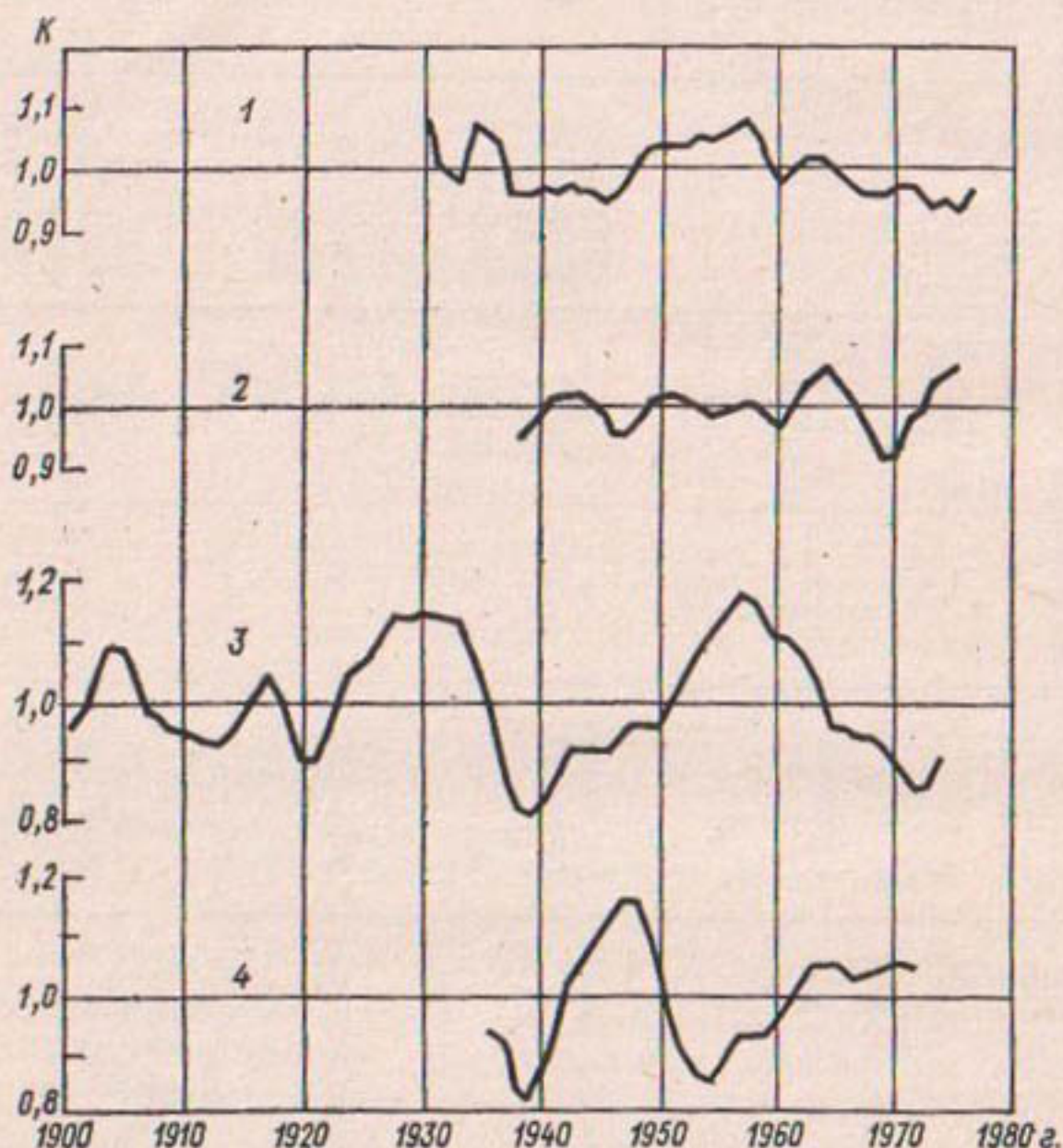
Рис. 5.13. Многолетние колебания динамических средних подземного стока в модульных коэффициентах для отдельных физико-географических районов. 1—4 — номера районов по табл. 5.23.
