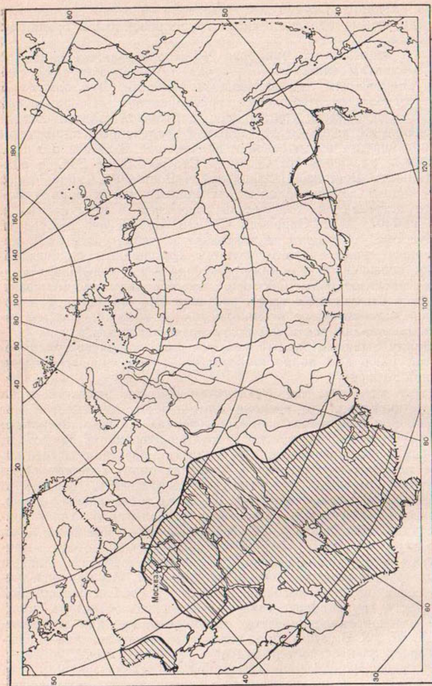
Рис. 3.2. Районы, в которых более половины рядов характеризуются неслучайным группированием лет различной водности в колебаниях наименьших расходов воды. (Критерий серий. Уровень значимости 5 %.)
