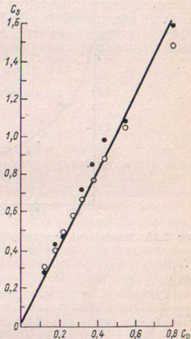
Рис. 2.21. Зависимость коэффициента асимметрии от коэффициента вариации.
