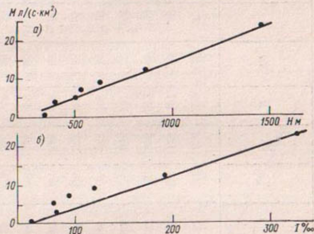
Рис. 2.20. Зависимость среднего многолетнего стока от средней высоты (а) и от среднего уклона (б) водосбора.
