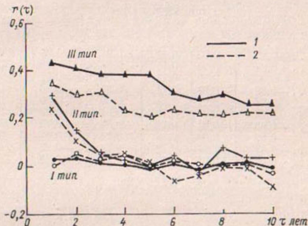
Рис. 3.16. Средние автокорреляционные функции осадков (1) и температуры воздуха (2) теплого периода.
