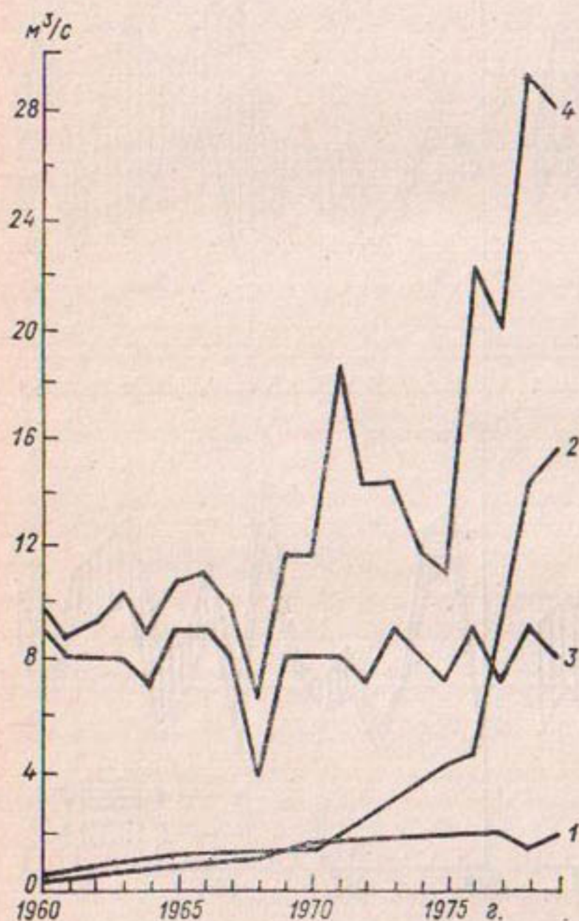
Рис. 3.20. Динамика безвозвратных потерь стока при различных видах водопотребления в бассейне р. Ишима.
