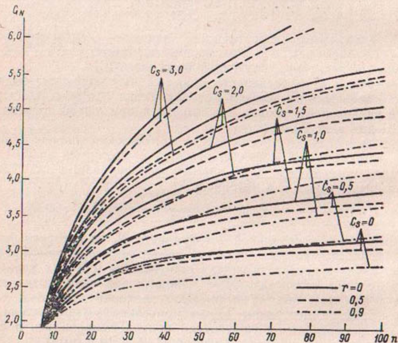
Рис. 1.4. Влияние асимметрии и автокорреляции на статистику G_N критерия Смирнова — Граббса при \alpha = 5\% .
