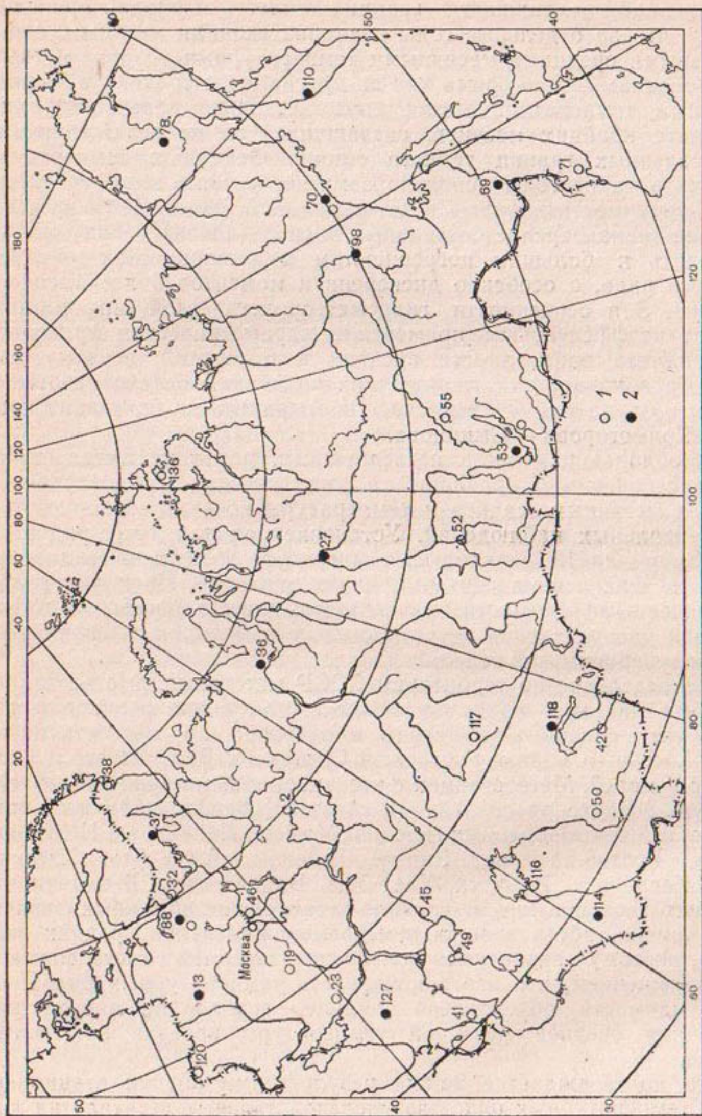
Рис. 3.17. Метеостанции с нестационарными рядами наблюдений по осадкам (1) и температуре воздуха (2) теплого периода.
