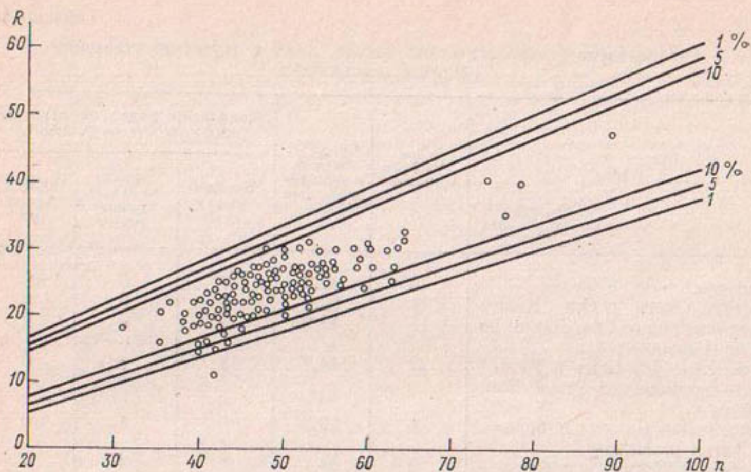
Рис. 4.6. Оценка гипотезы случайности рядов минимального летне-осеннего стока рек АТС по общему числу серий ( R ).
