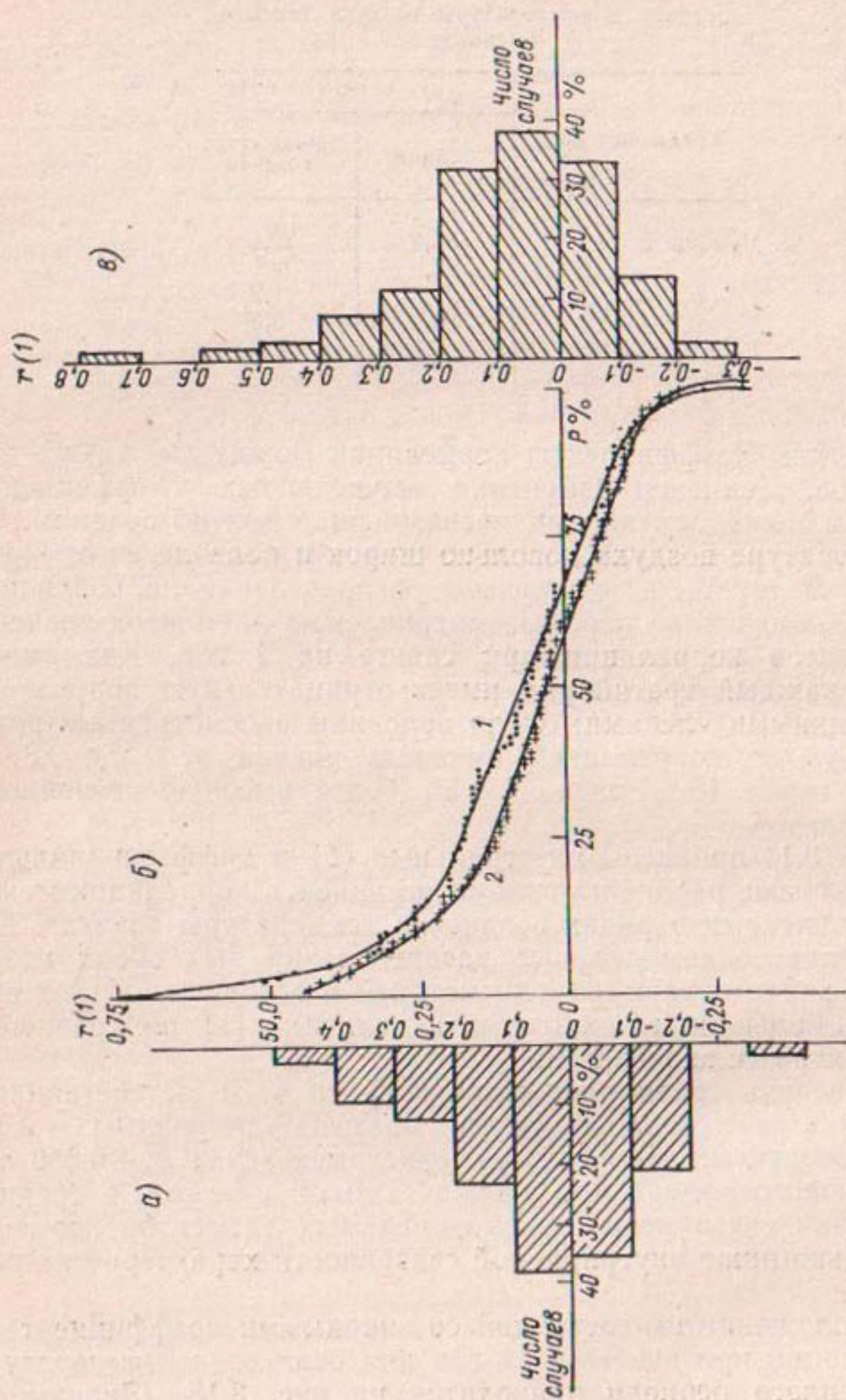
Рис. 3.14. Дифференциальные (а, б) кривые распределения и кривые распределения r(1) (б) в рядах температуры и осадков. 1) r(1) для осадков, 2) r(1) для температуры воздуха.
