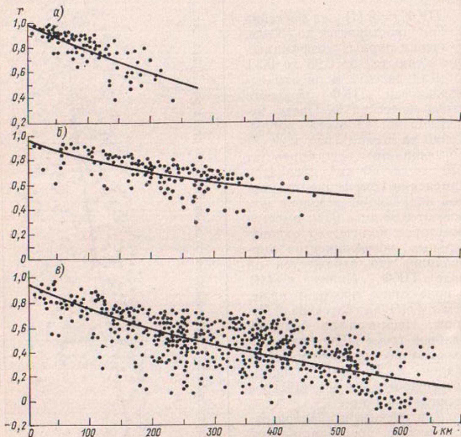
Рис. 2.30. Пространственная корреляционная функция годового стока рек Эстонии (а), рек Латвии (б) и рек Литвы и Калининградской обл. (в).
