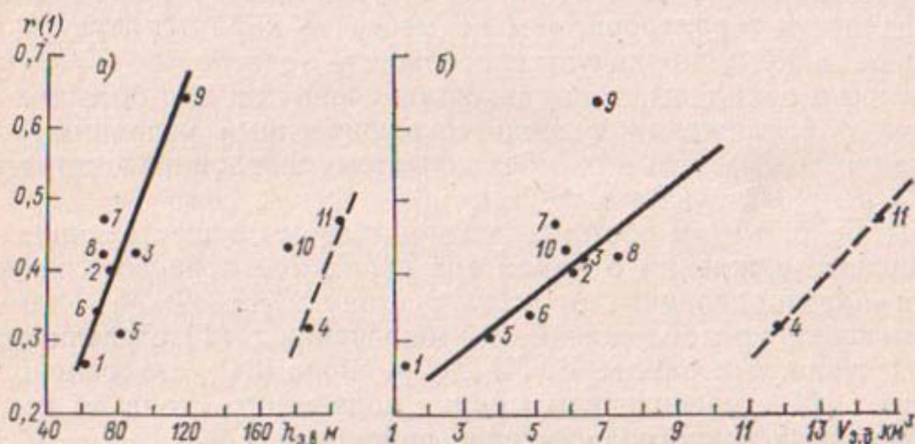
Рис. 5.8. Зависимость коэффициентов корреляции между подземным стоком смежных лет r(1) от глубины эрозионного вреза речного русла (а) и объема дренируемой зоны речного бассейна (б). Цифры у точек — номера районов по табл. 5.16.
