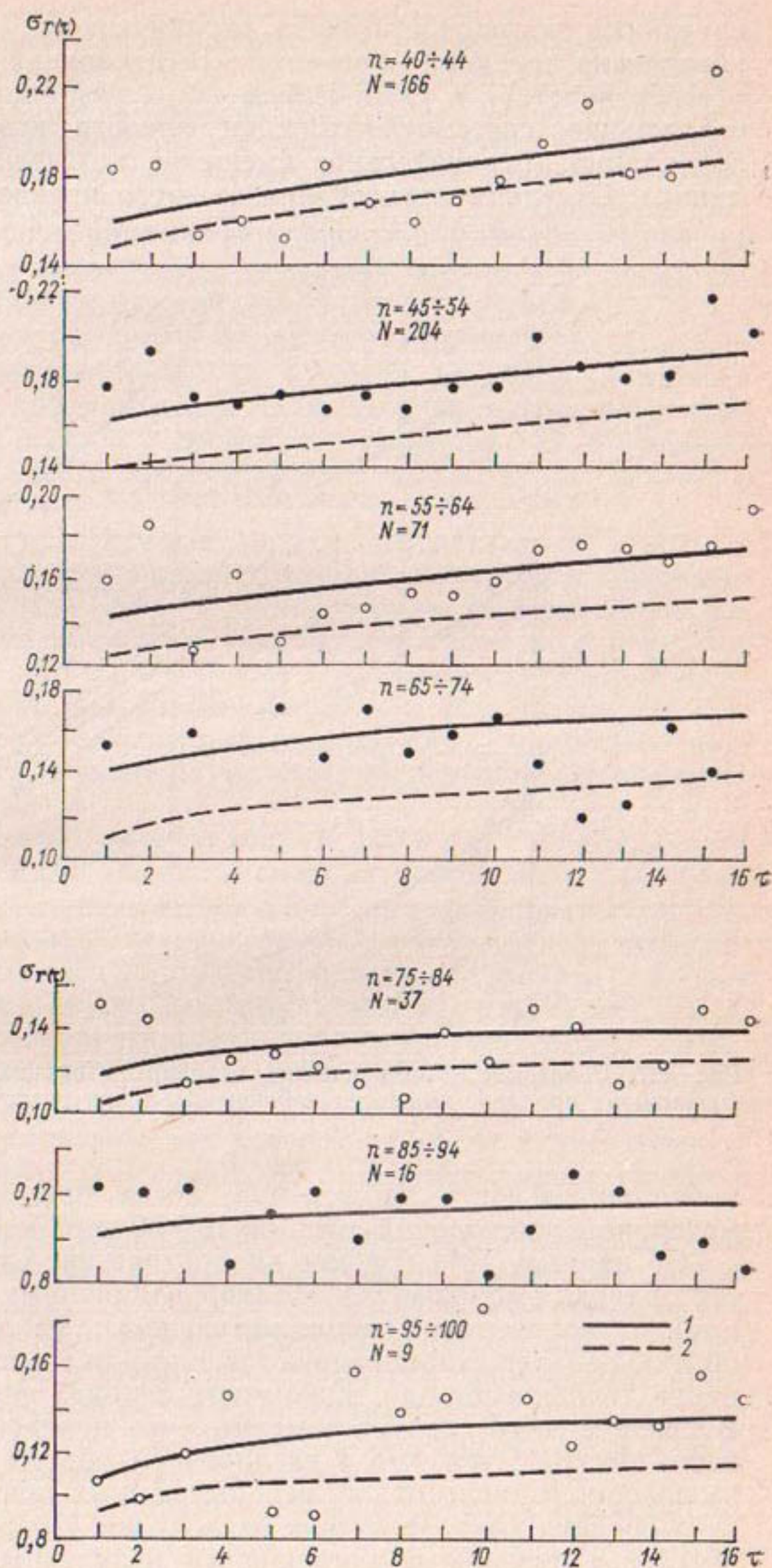
Рис. 2.6. Зависимость эмпирических средних квадратических отклонений ординат автокорреляционных функций от сдвига \tau при различной продолжительности рядов наблюдений.
