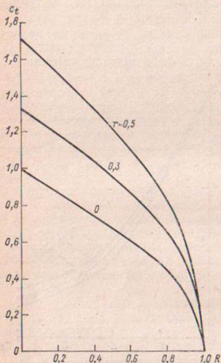
Рис. 1.9. Зависимость c_t = f(R, r) .
