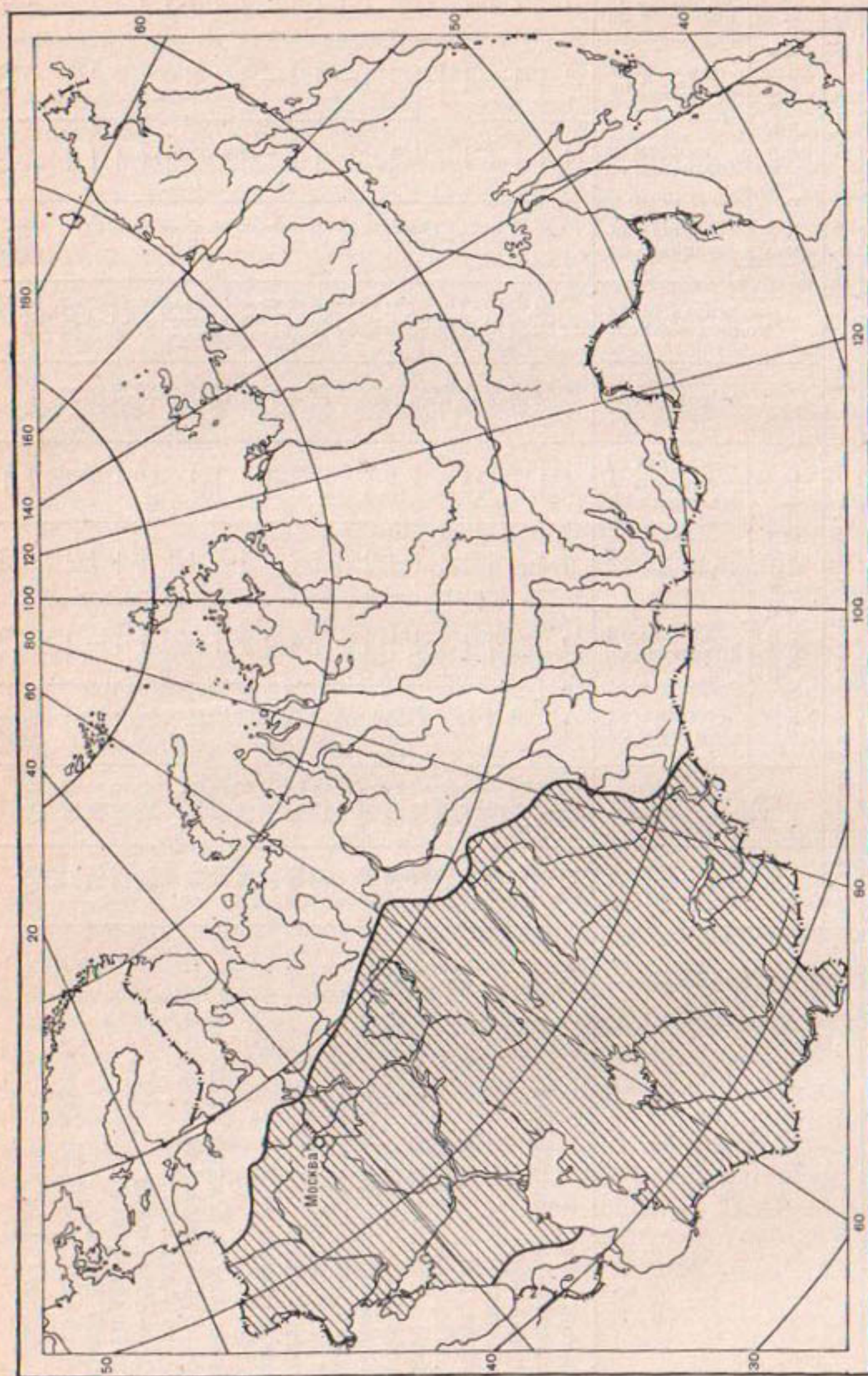
Рис. 3.8. Районы, в которых более 25 % рядов характеризуются нестационарностью минимального стока.
