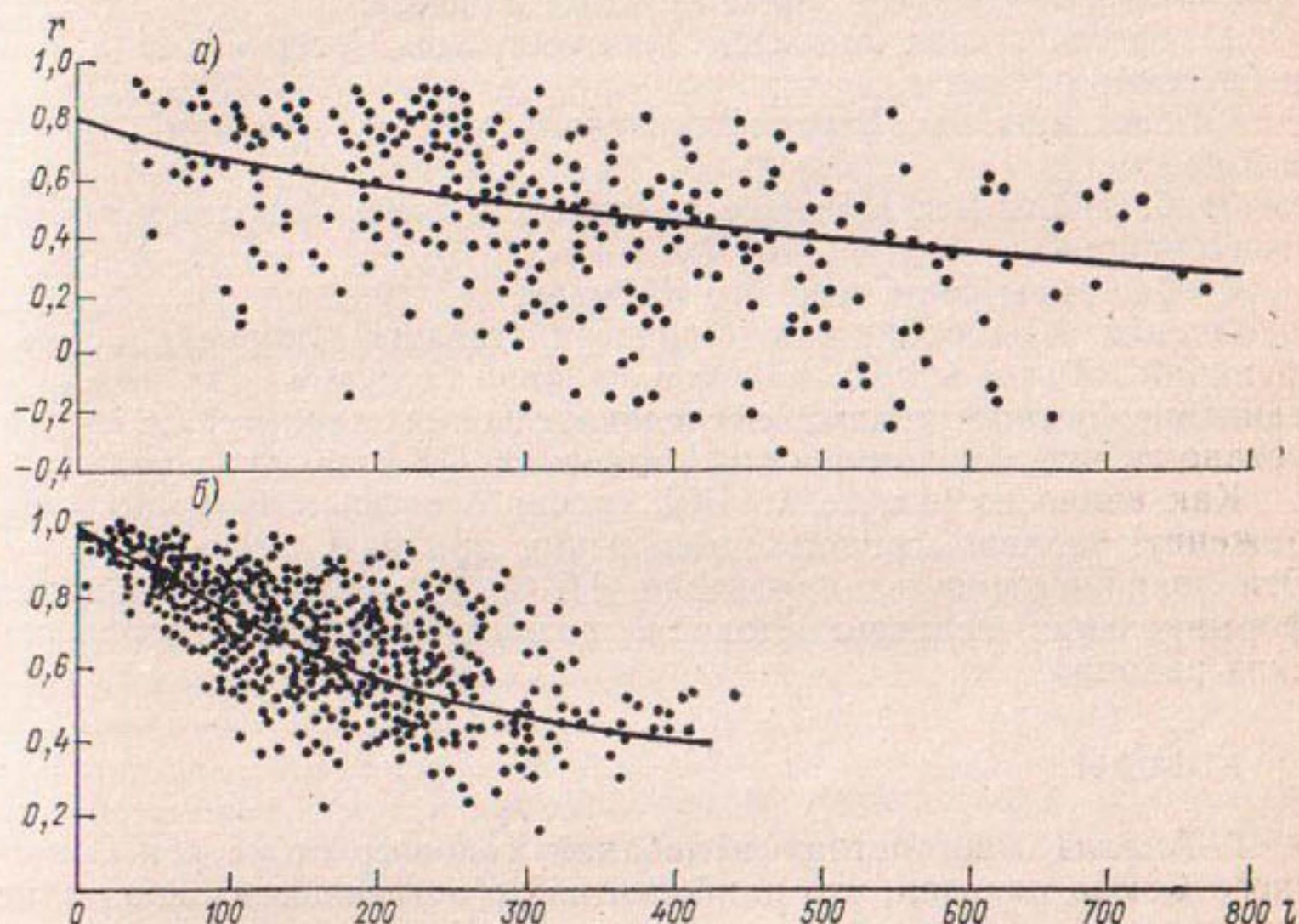
Рис. 2.38. Пространственная корреляционная функция годового стока рек Ангара-Енисейского района (а) и рек Приморья (б).
