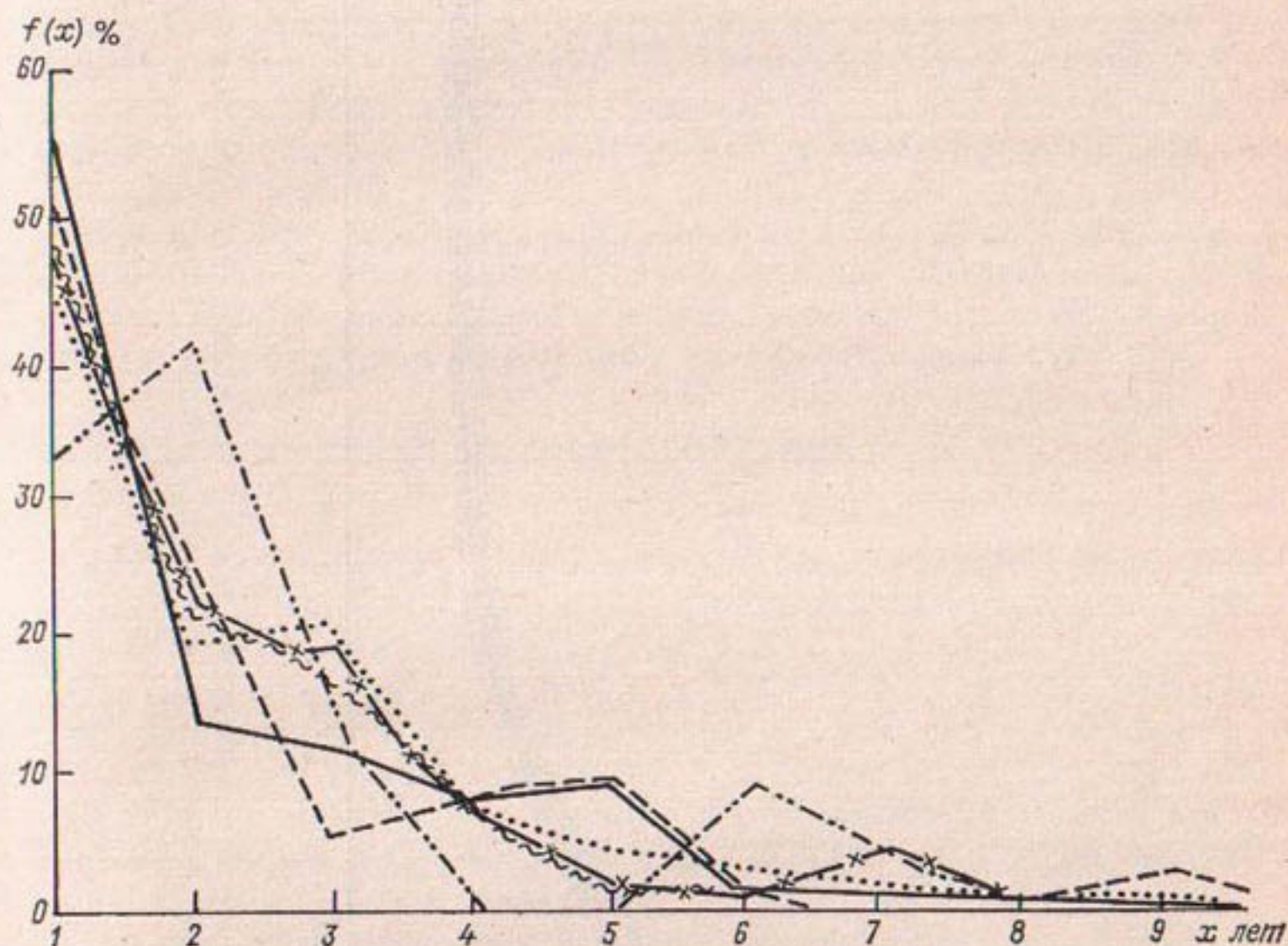
Рис. 4.2. Гистограмма вероятностей появления серий пониженной водности различной продолжительности для рядов средних месячных расходов воды.
