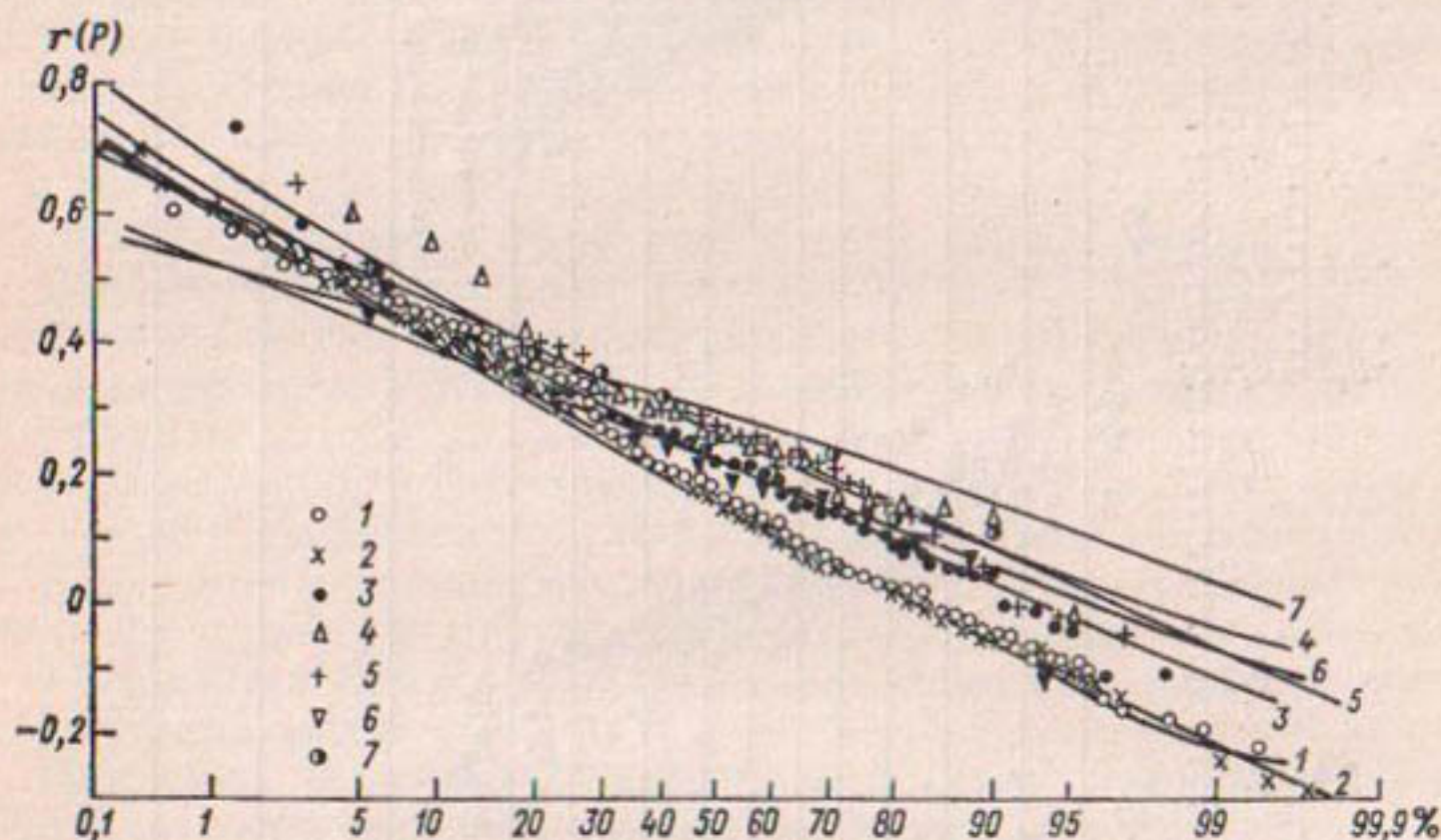
Рис. 2.5. Совмещенные кривые обеспеченности коэффициентов корреляции при \tau=1 при различном объеме исходных данных.
