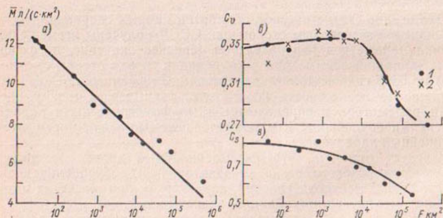
Рис. 2.16. Зависимость среднего многолетнего стока (а), коэффициента вариации (б) и коэффициента асимметрии (в) от площади водосбора.
