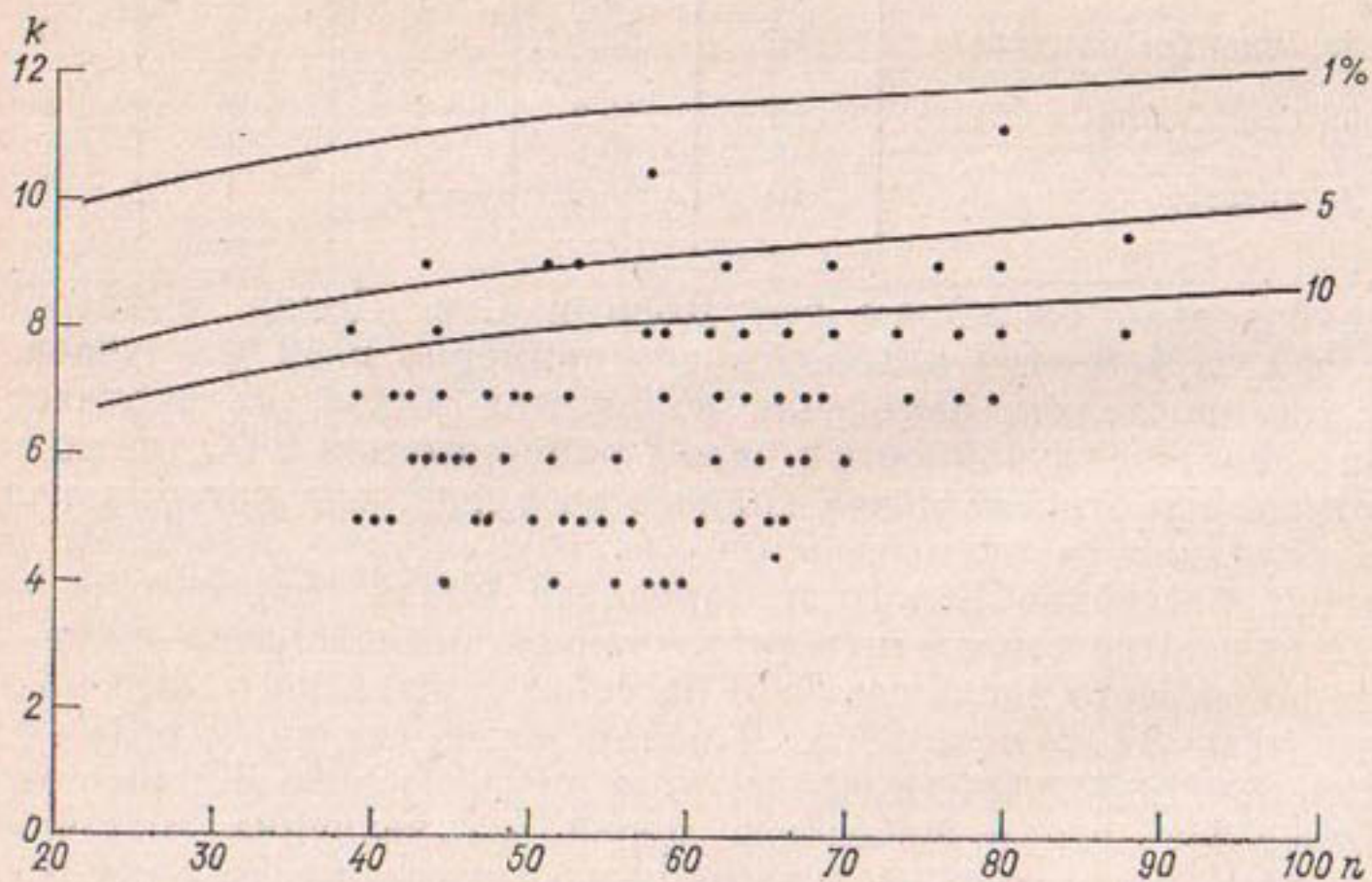
Рис. 4.7. Оценка гипотезы случайности рядов минимального летне-осеннего стока рек АТС по максимальной длине серий ( k ).
