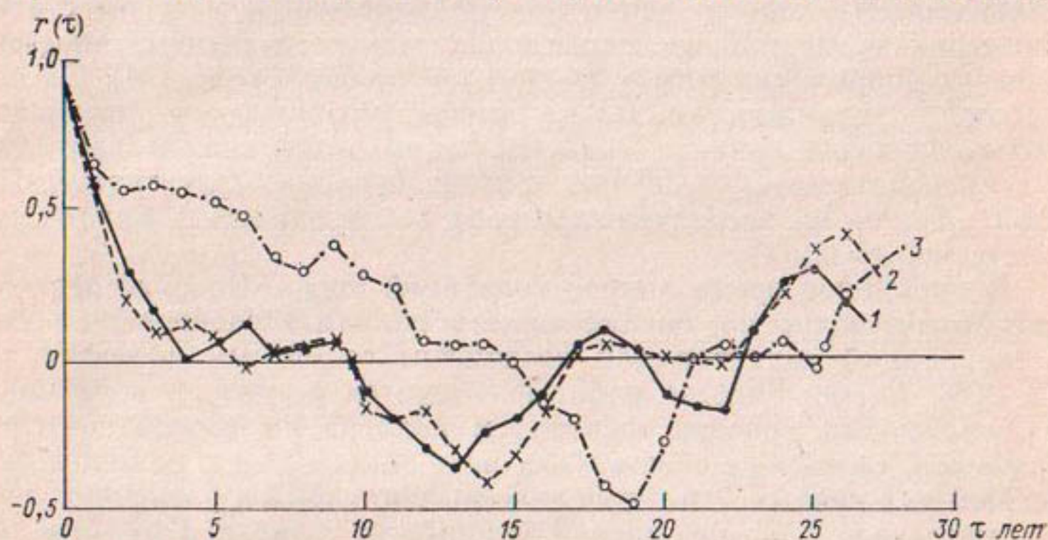
Рис. 6.6. Автокорреляционные функции среднегодовых значений уровня озера Селлигер.
