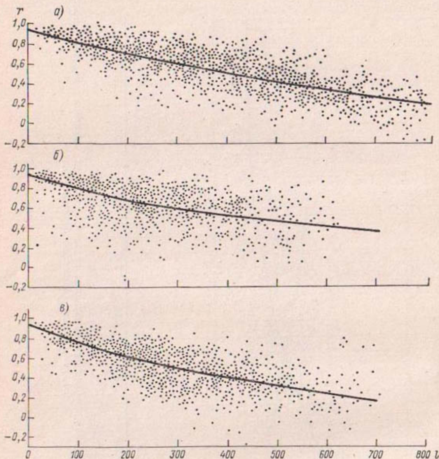
Рис. 2.36. Пространственная корреляционная функция годового стока рек Среднего Урала и Приуралья.
