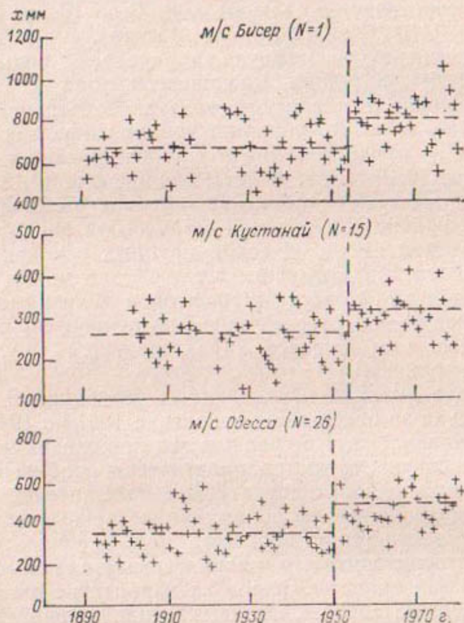
Рис. 2.15. Характерные виды нестационарности за счет замены регистрирующих приборов в рядах годовых сумм осадков.
