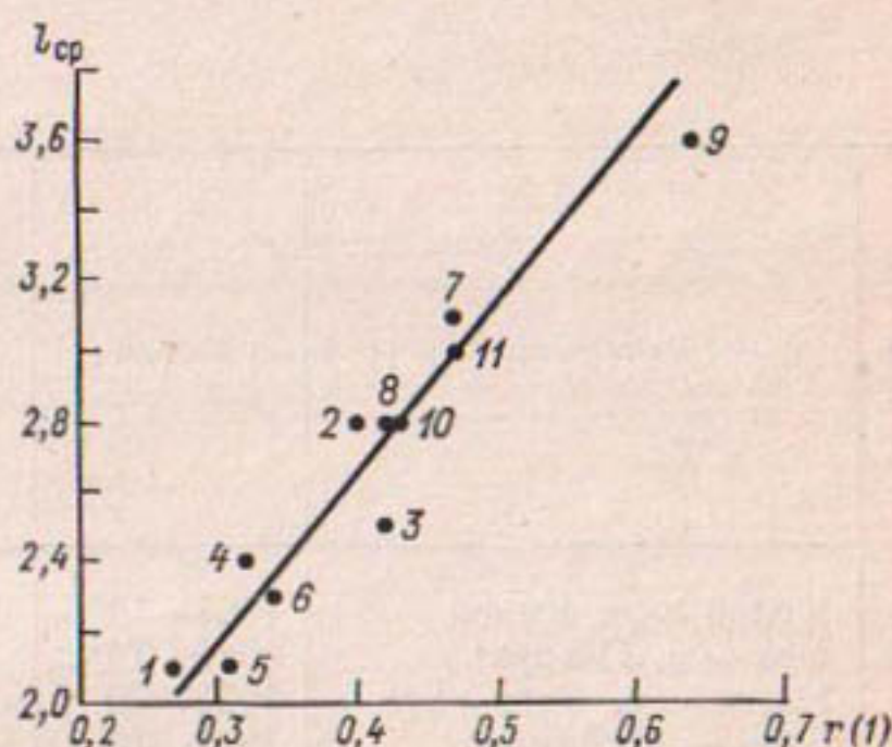
Рис. 5.9. Зависимость средней продолжительности группировок лет различной водности ( l_{\text{ср}} ) от коэффициента корреляции между стоком смежных лет r(1) в рядах подземного стока.
