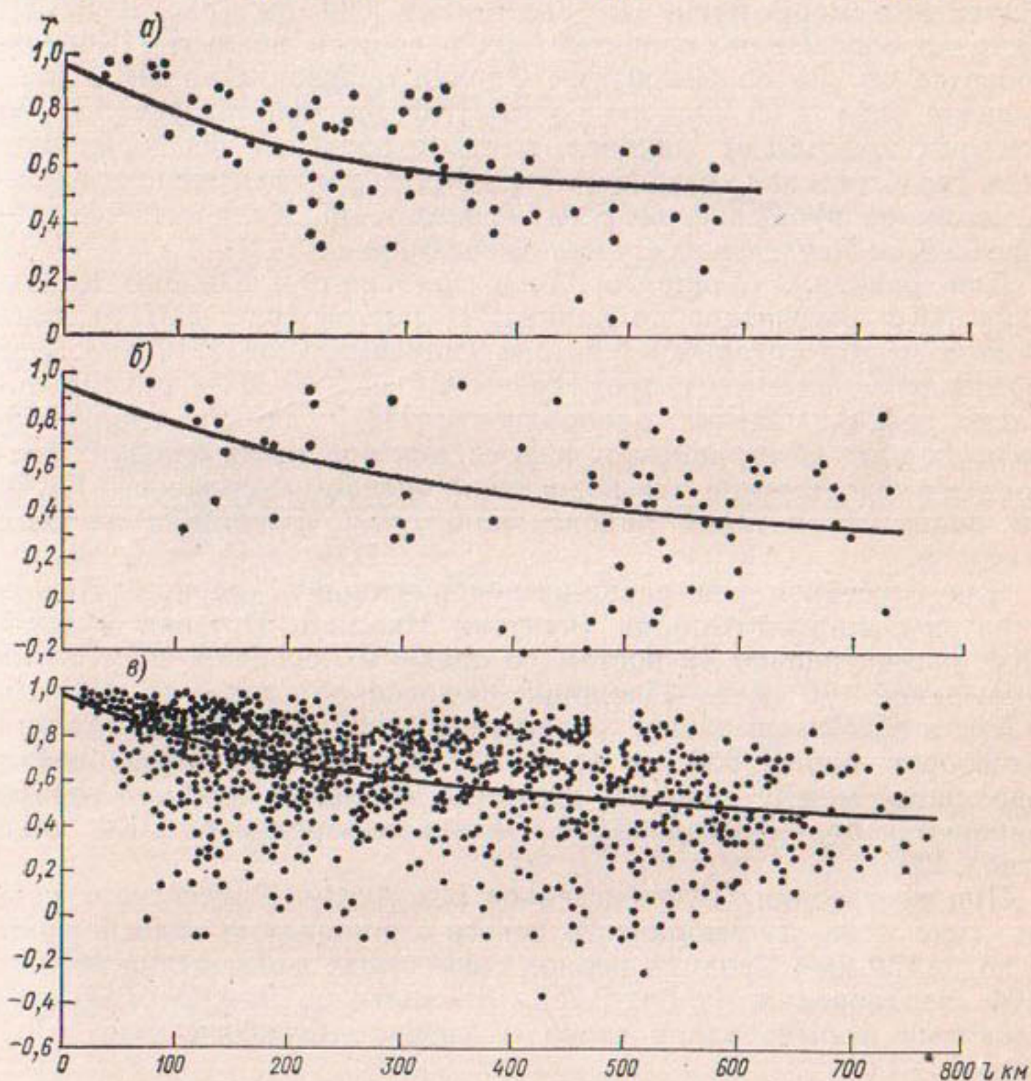
Рис. 2.37. Пространственная корреляционная функция годового стока рек Урало-Эмбинского района (а), рек Центрального и Южного Казахстана (б) и равнинных территорий Северного Казахстана и Западной Сибири (притоки Нижнего Иртыша и Оби) (в).
