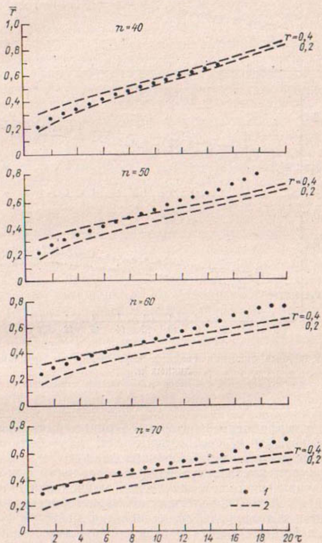
Рис. 2.9. Осредненные значения сводных корреляционных функций при различных n .
