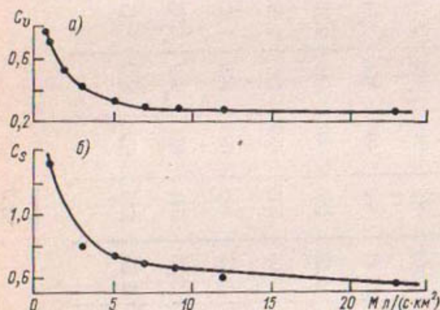
Рис. 2.19. Зависимость коэффициента вариации ( а ) и коэффициента асимметрии ( б ) от среднего многолетнего стока.
