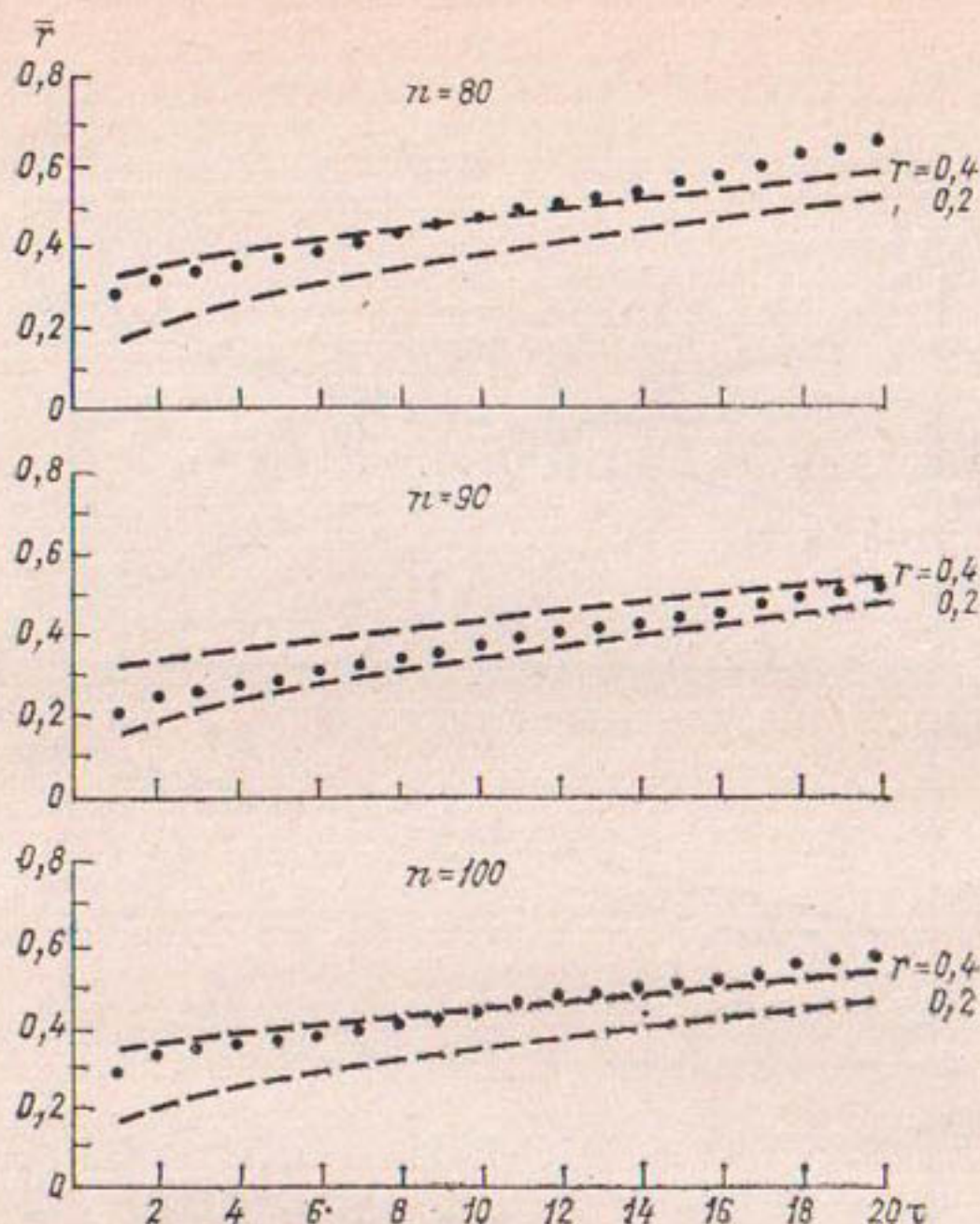
Рис. 2.9. Осредненные значения сводных корреляционных функций при различных n .
