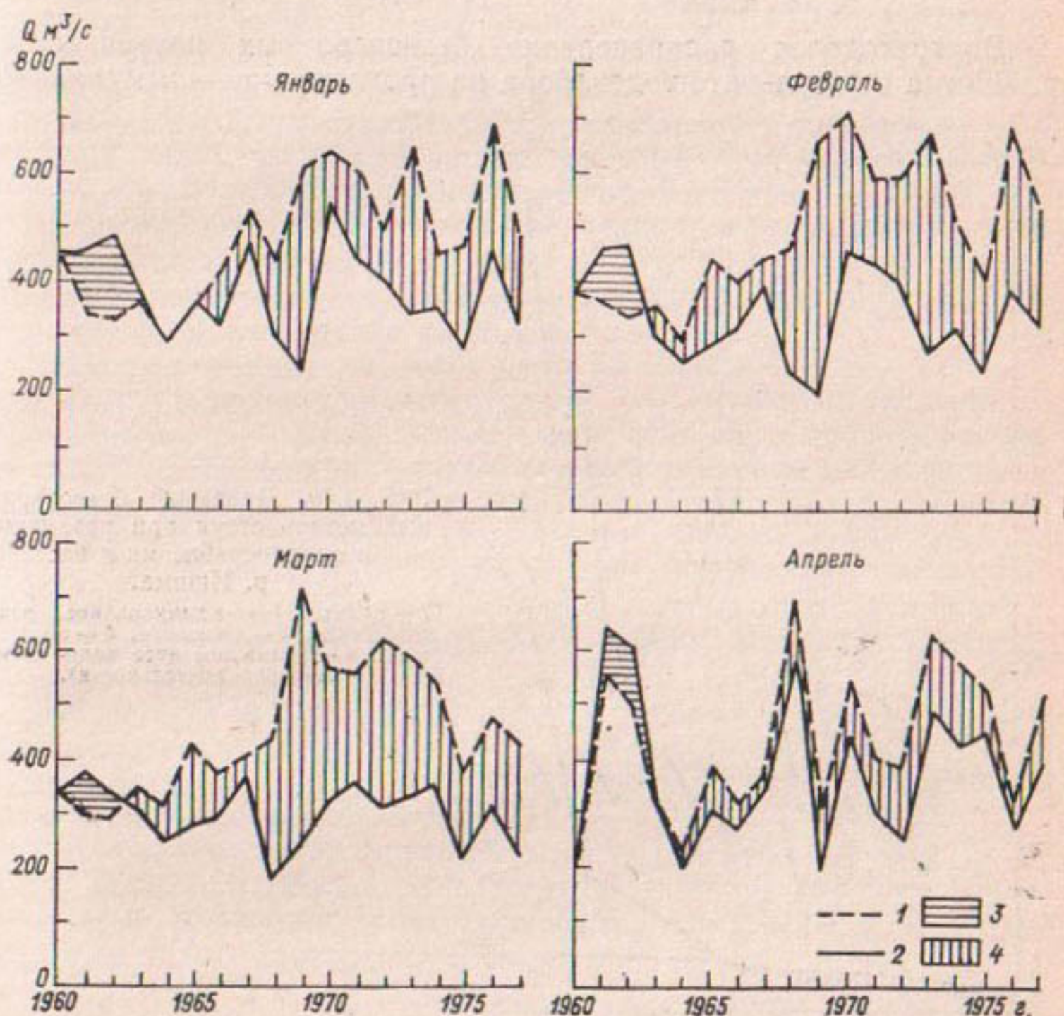
Рис. 3.19. Фактический (1) и восстановленный (2) средний месячный сток р. Иртыша у г. Омска, Антропогенное уменьшение (3) и увеличение (4) стока.
