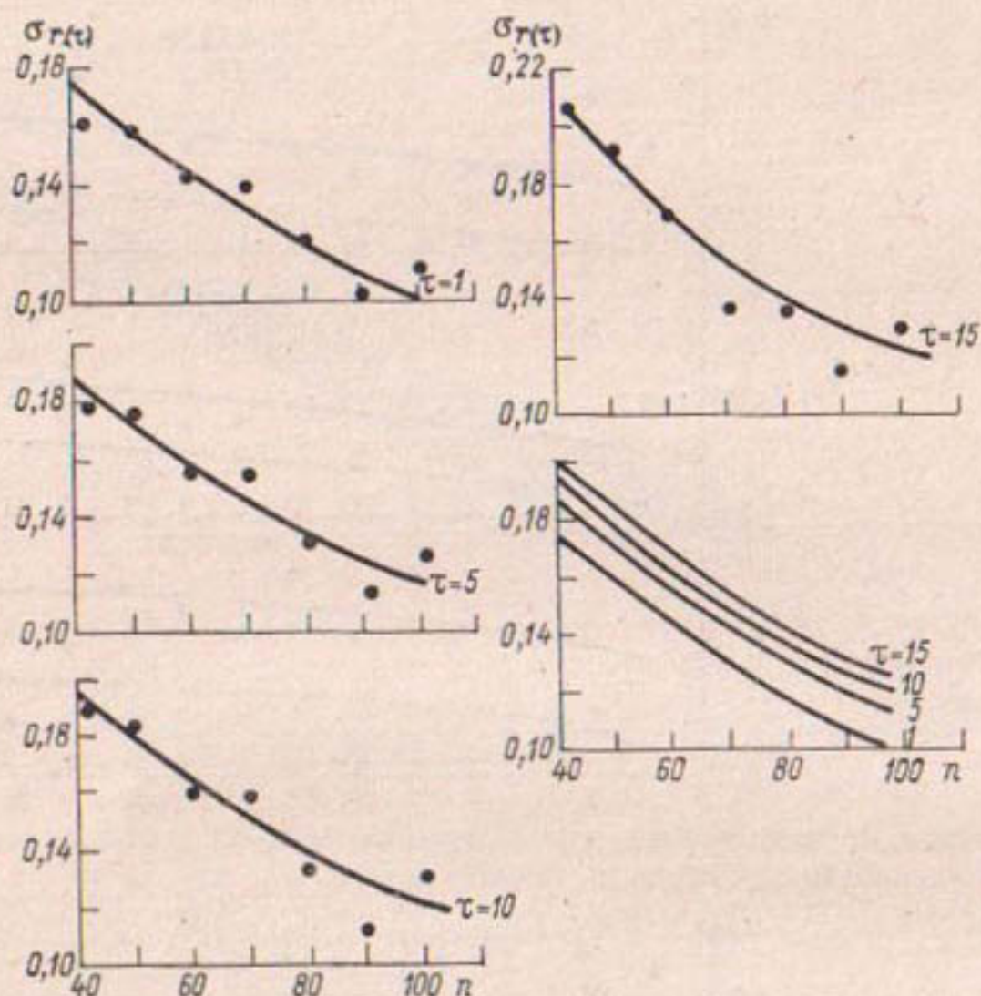
Рис. 2.7. Зависимость эмпирических стандартов ординат автокорреляционных функций от продолжительности наблюдений n при различной сдвиге рядов \tau .
