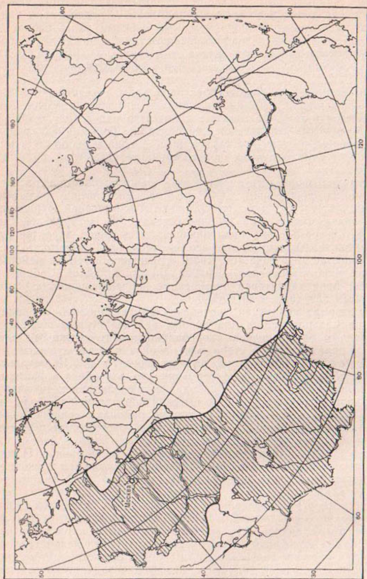
Рис. 3.7. Районы, в которых более 25 % постов имеют АКФ III типа. Наименьшие годовые расходы воды.
