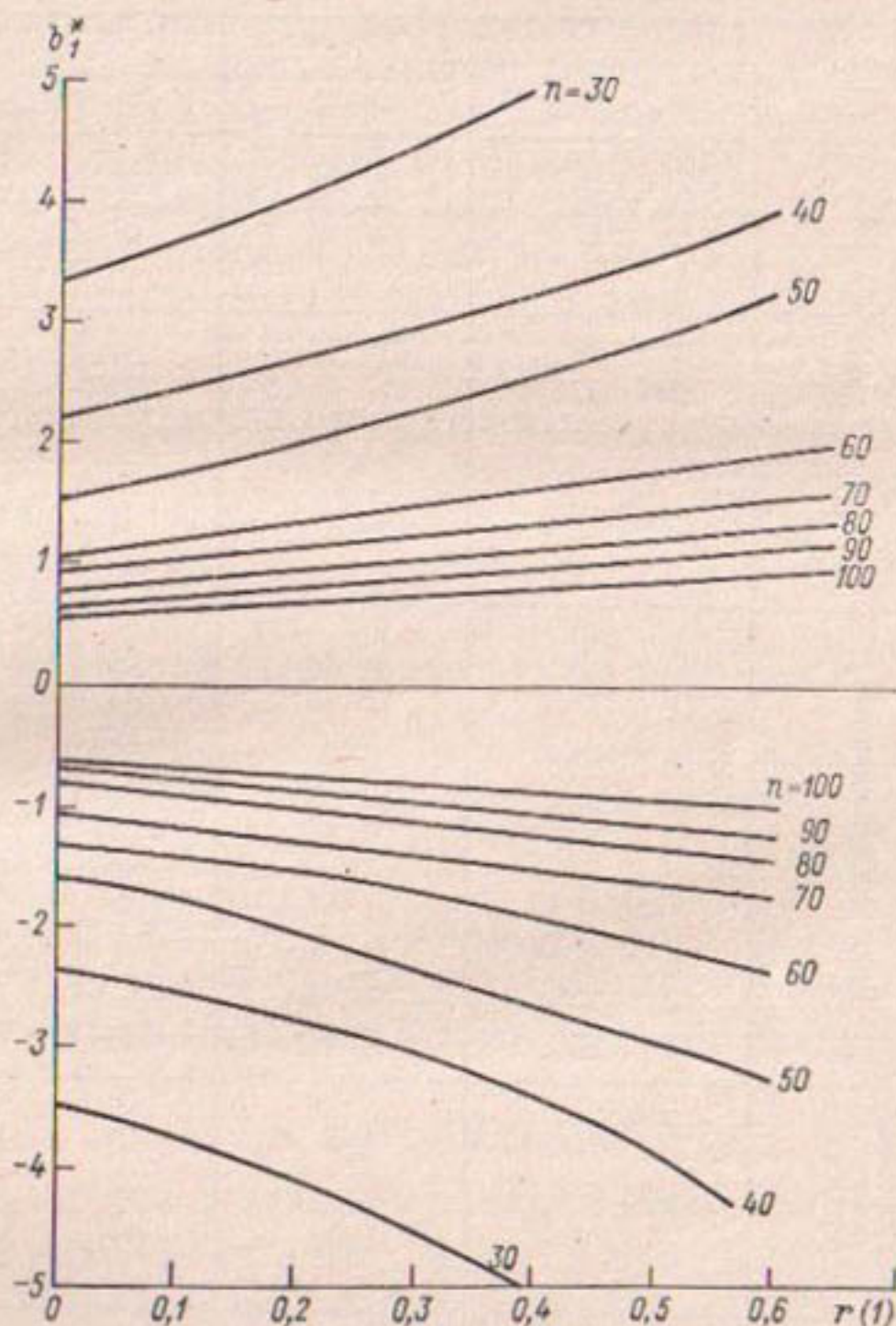
Рис. 1.10. Номограмма критических значений b_1^* для n=30 \div 100 при уровне значимости \alpha=5\% .
