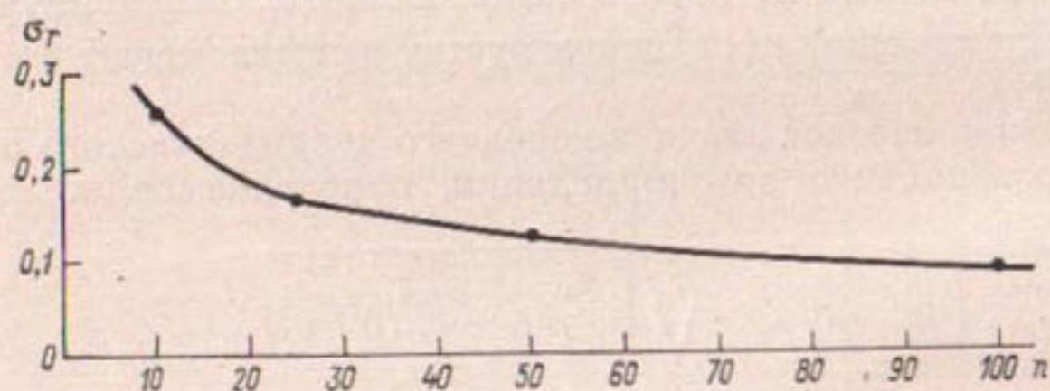
Рис. 2.11. Зависимость \sigma_r=f(n) при r=0,3 .
