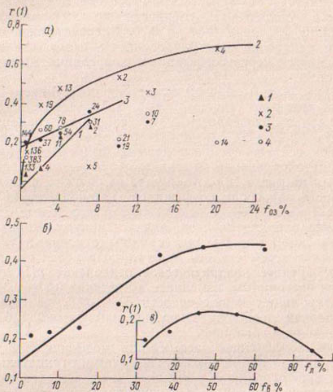
Рис. 2.12. Зависимость коэффициента автокорреляции \bar{r}(1) от озерности бассейна (а), заболоченности (б), залесенности (в).
