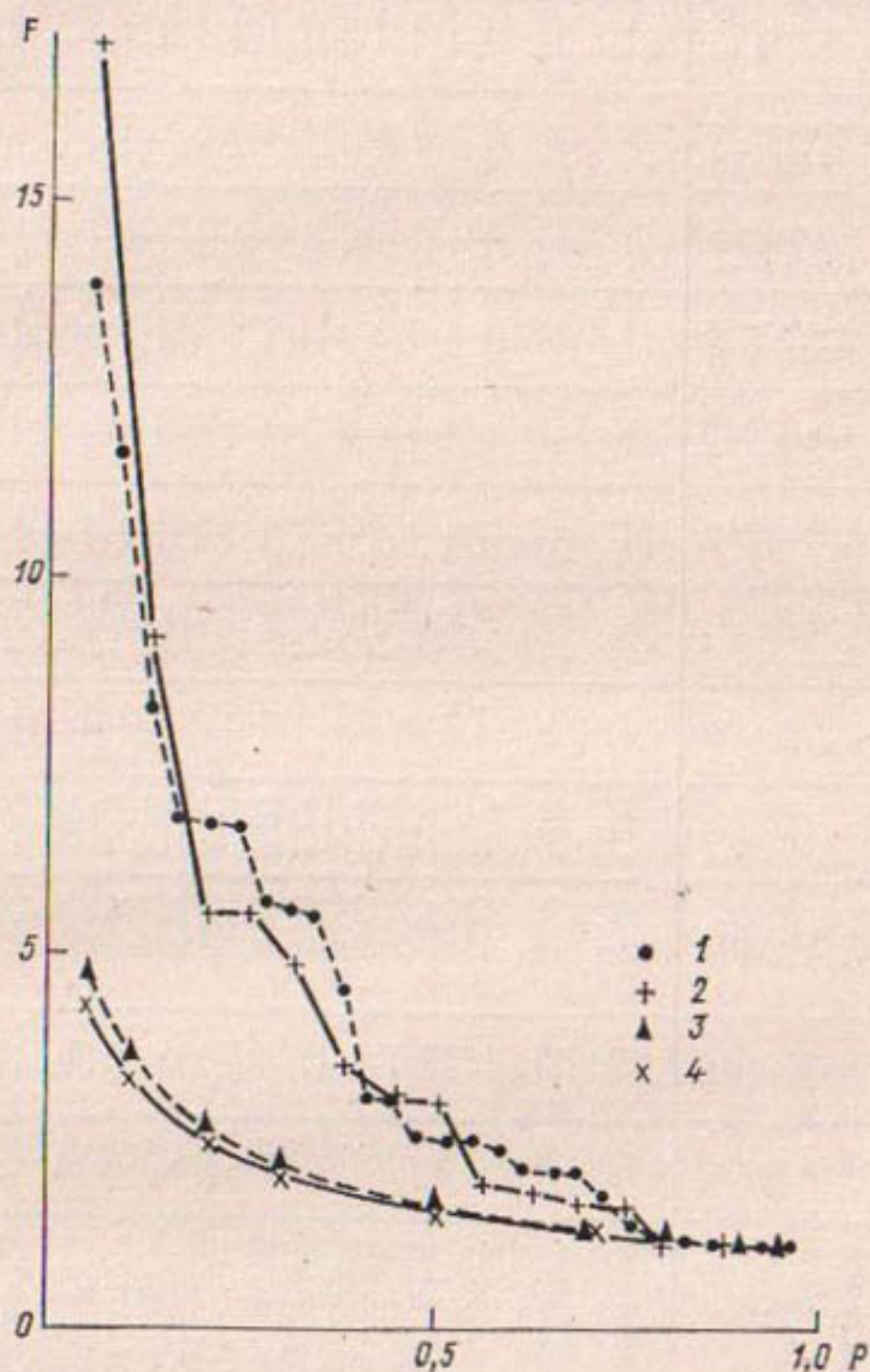
Рис. 3.9. Распределение F-статистик в рядах с непрезентативной величиной. 1 — р. Томь — г. Новокузнецк ( N=85 , r_1=0,41 ), 2 — р. Волга — г. Ельцы ( N=61 , r_1=0,22 ), 3 — теоретическое распределение Фишера с r_1=0,41 , 4 — то же с r_1=0,22 .
