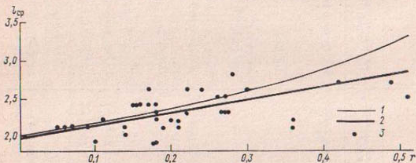
Рис. 2.1. Зависимость средней длительности группировок от коэффициента автокорреляции годового стока.
