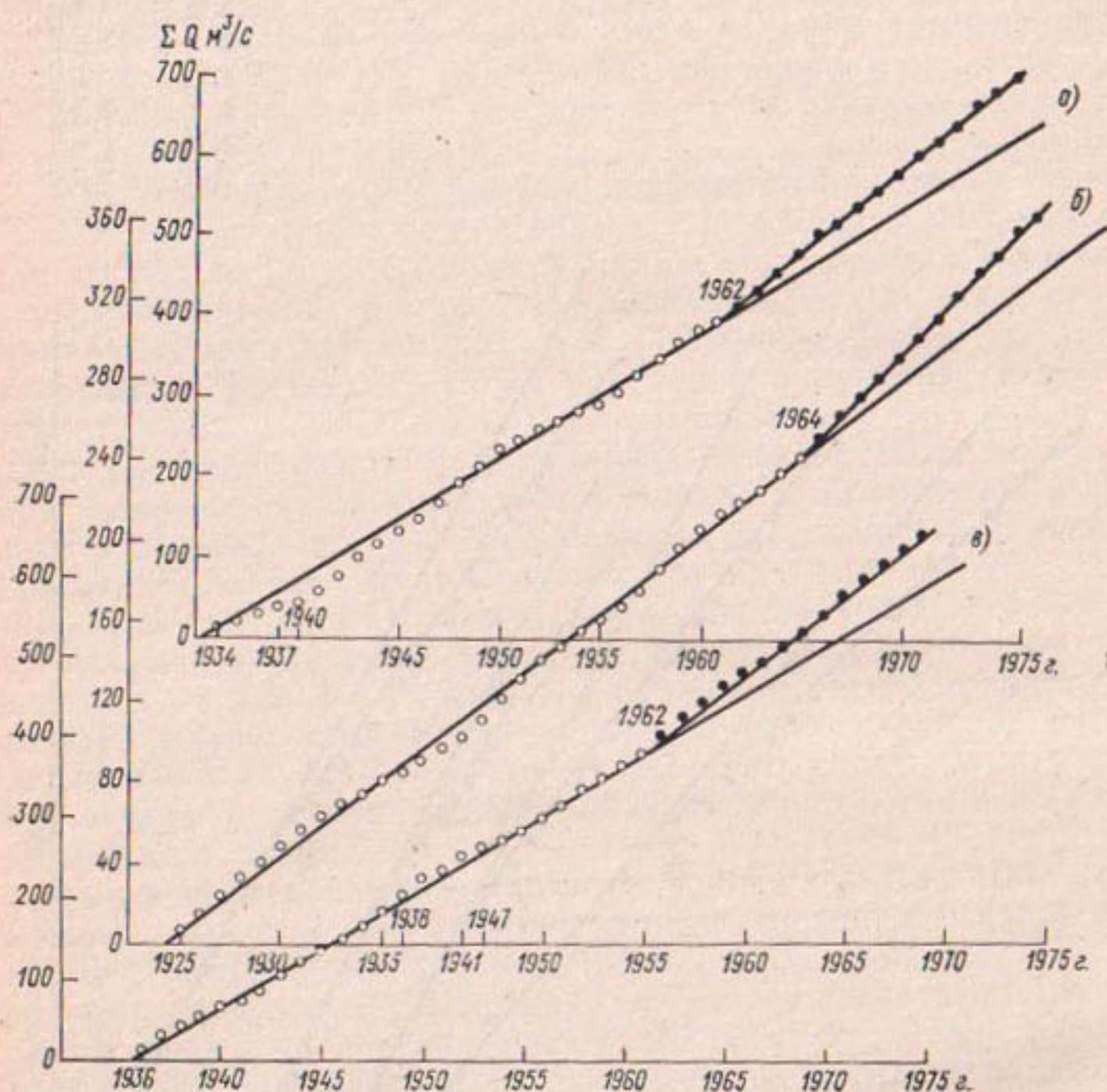
Рис. 5.11. Графики последовательно суммированных по времени значений подземного стока.
