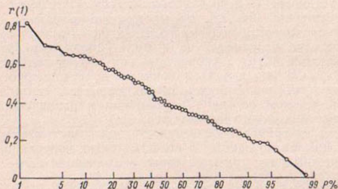
Рис. 5.2. Эмпирическая кривая обеспеченности коэффициентов корреляции между стоком смежных лет r(1) для всей совокупности рядов подземного стока.
