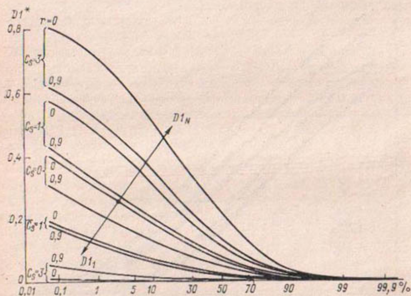
Рис. 1.2. Влияние асимметрии и автокорреляции на распределение критических значений статистики критерия Диксона ( D1 ).
