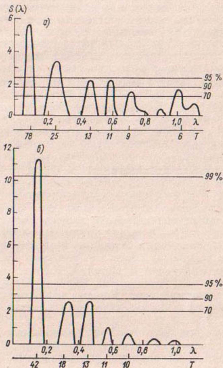
Рис. 6.7. Спектральные плотности уровня озер Байкала (а) и Б. Чаны (б).
