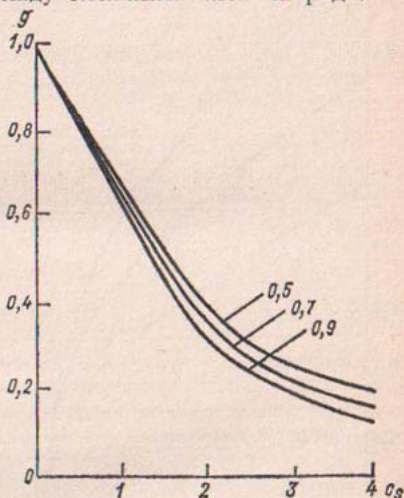
Рис. 1.8. Зависимость g = f(C_s, R) .
