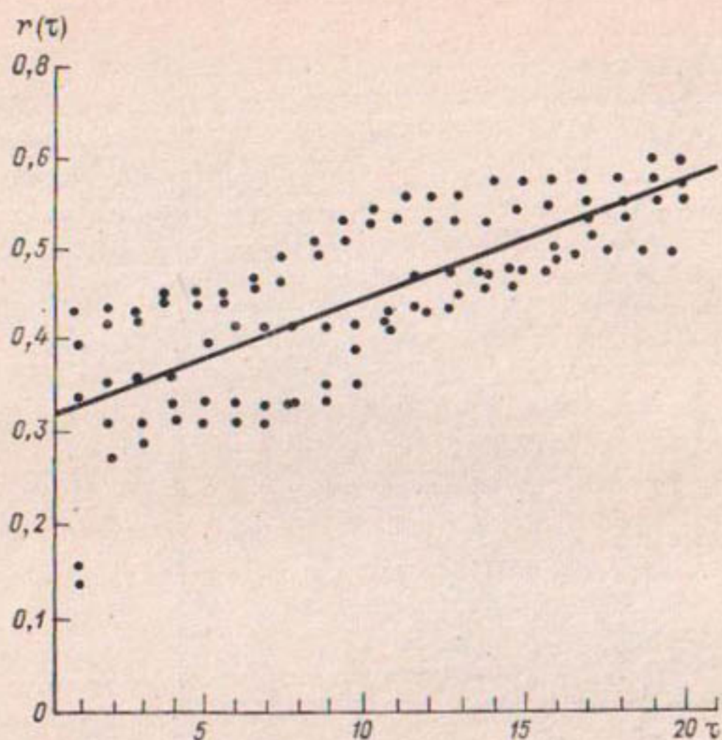
Рис. 2.8. Сводная корреляционная функция для n = 95 \div 104 .
