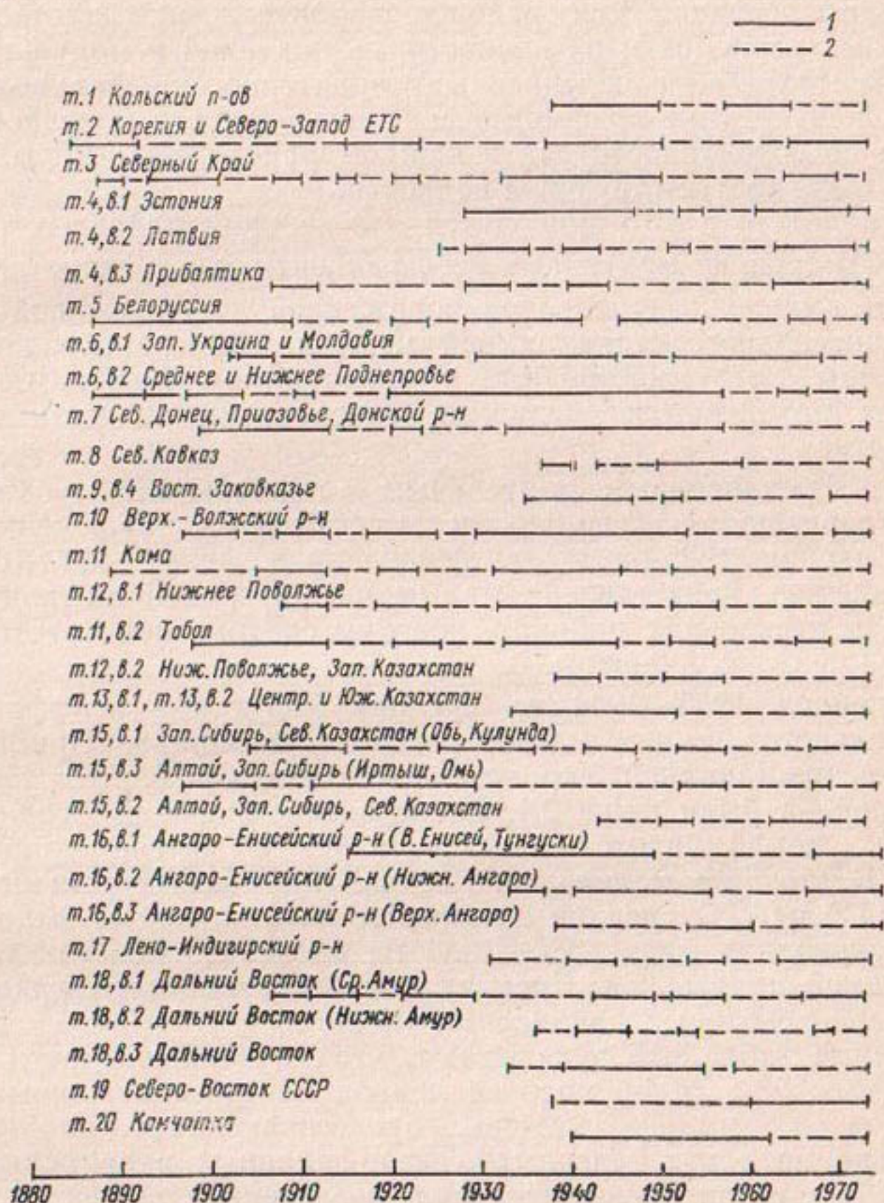
Рис. 3.10. Динамическая средняя. Периоды повышенной (1) и пониженной (2) водности в колебаниях зимних минимумов.
