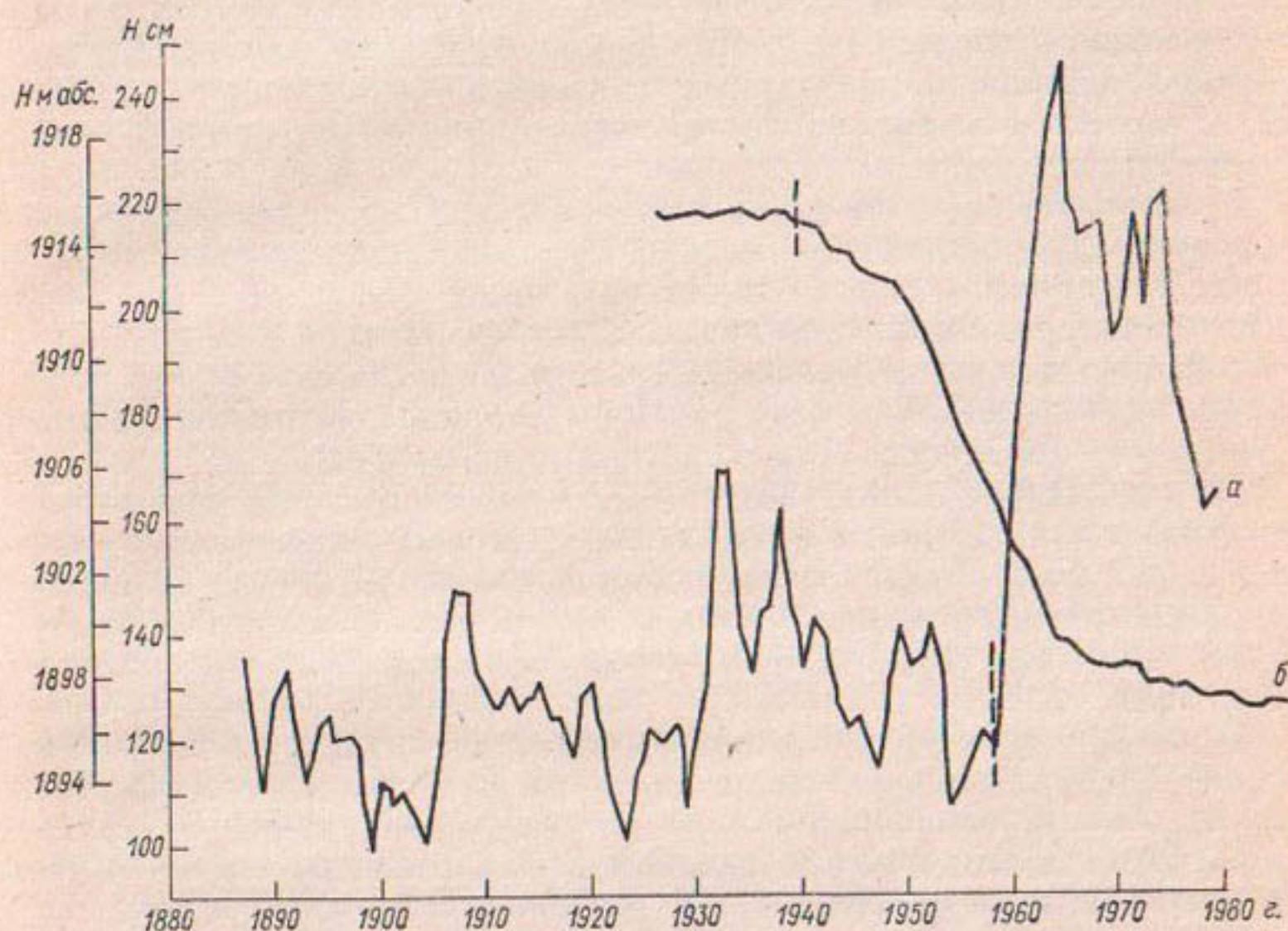
Рис. 6.3. Хронологические графики колебаний уровня озер, подверженных антропогенному влиянию. а — оз. Байкал; б — оз. Севан.
