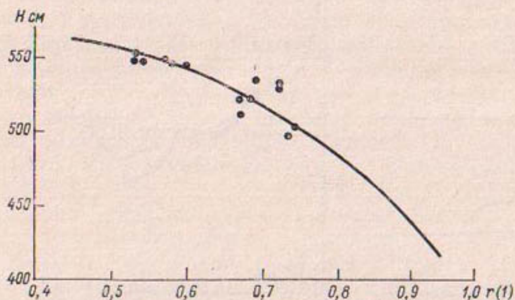
Рис. 6.5. Зависимость коэффициента корреляции смежных значений уровня от наполнения озера. Ладожское озеро, 60-летние выборки.
