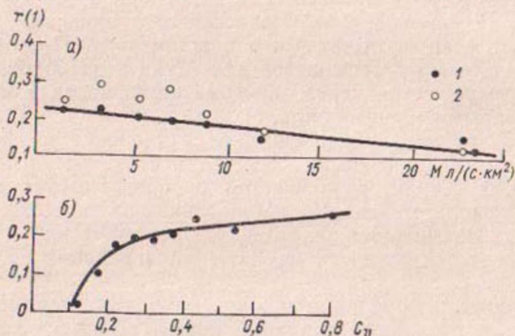
Рис. 2.13. Зависимость коэффициентов автокорреляции от модуля годового стока (а) и от коэффициента вариации годового стока (б).
