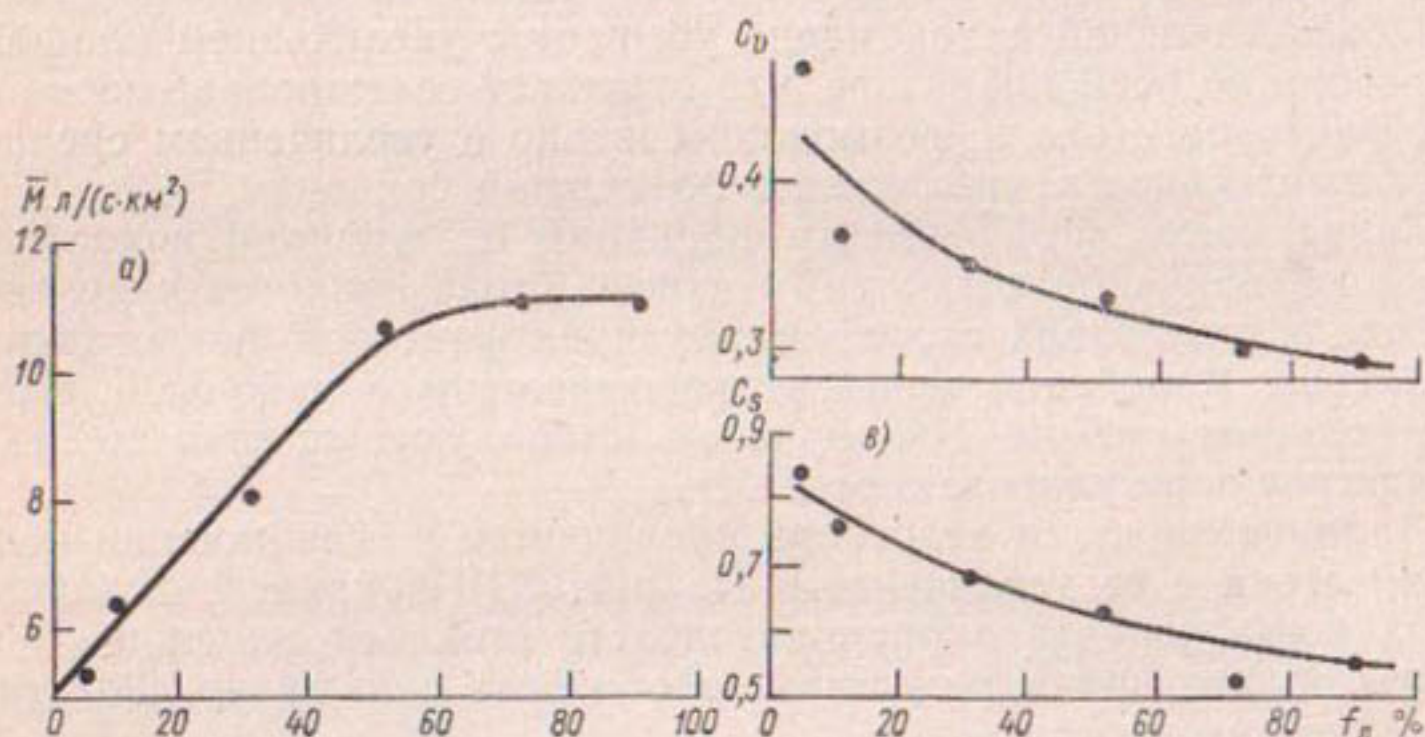
Рис. 2.17. Зависимость среднего многолетнего стока (а), коэффициента вариации (б) и коэффициента асимметрии (в) от залесенности водосбора.
