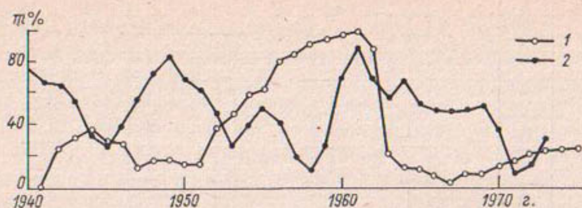
Рис. 4.9. Изменение количества рек (в % от общего числа), для которых наблюдается многоводная фаза.
