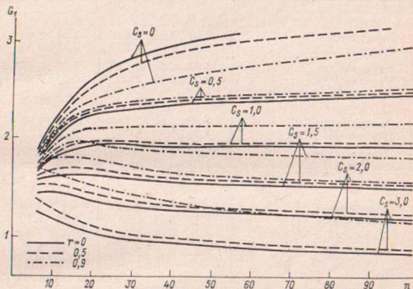
Рис. 1.5. Влияние асимметрии и автокорреляции на статистику G_1 критерия Смирнова — Граббса при \alpha=5\% .
