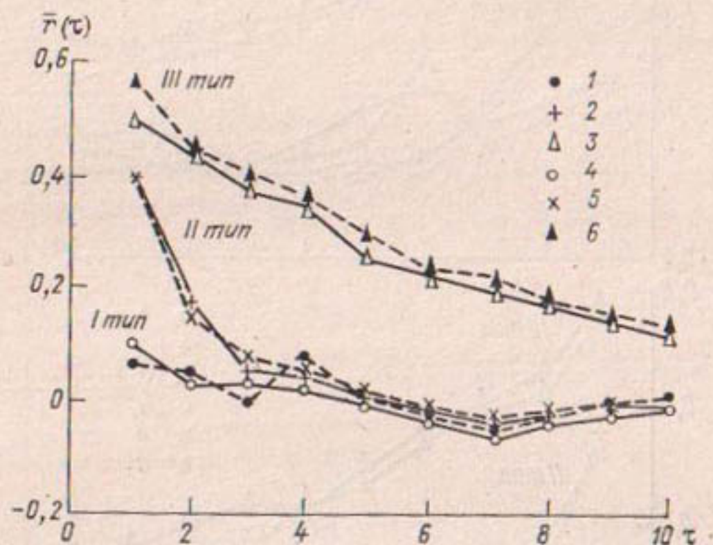
Рис. 3.6. Средние АКФ минимального стока рек СССР.
