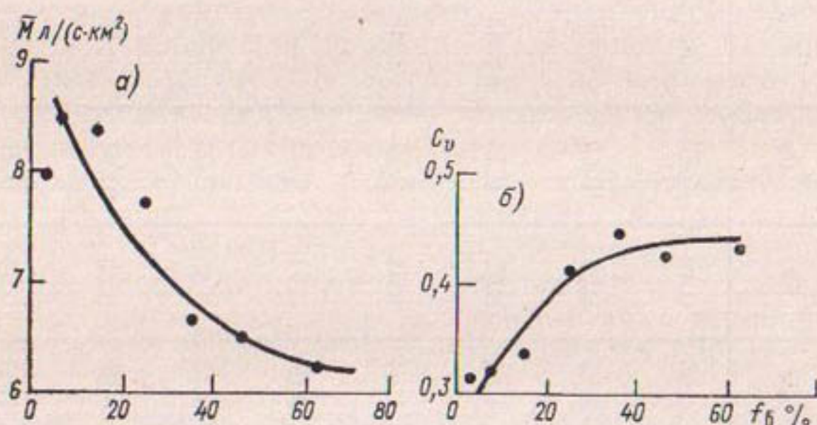
Рис. 2.18. Зависимость среднего многолетнего стока (а) и коэффициента вариации (б) от заболоченности водосбора.
