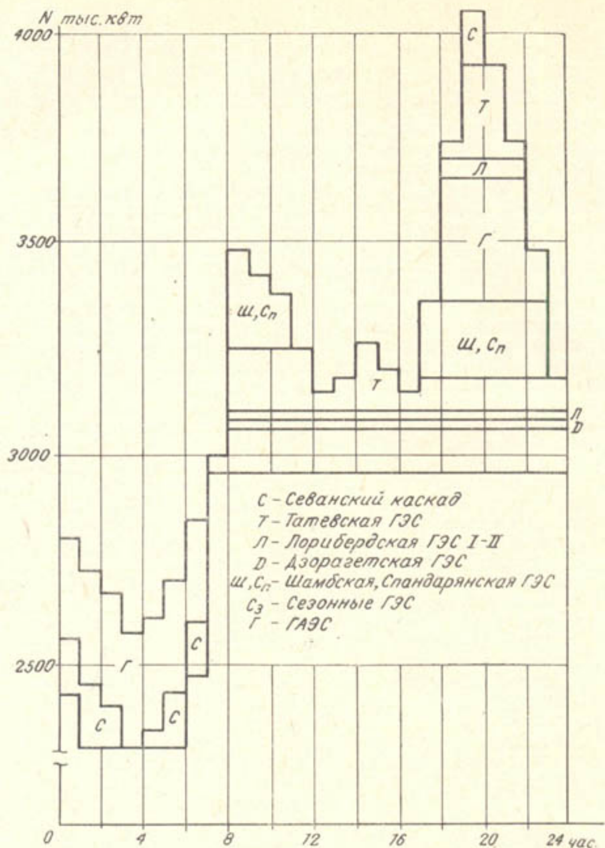
Рис. 1. Покрытие суточного графика нагрузки Армянской энергосистемы в перспективе, зима.
