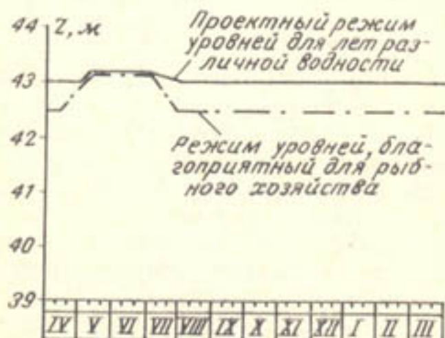
Рис. 3. Уровни Саратовского водохранилища.
