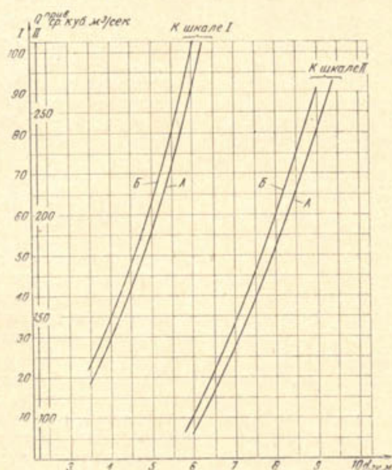
Рис. 4. Зависимость между Q_{крив. ср. куб.} и экономическим диаметром туннеля:
