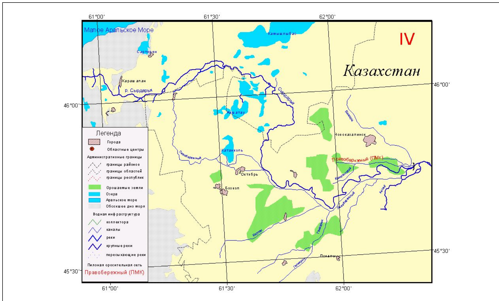
Рис. 4.5. Схема расположения оросительной системы Правобережного Магистрального Канала Казалинского Гидроузла
