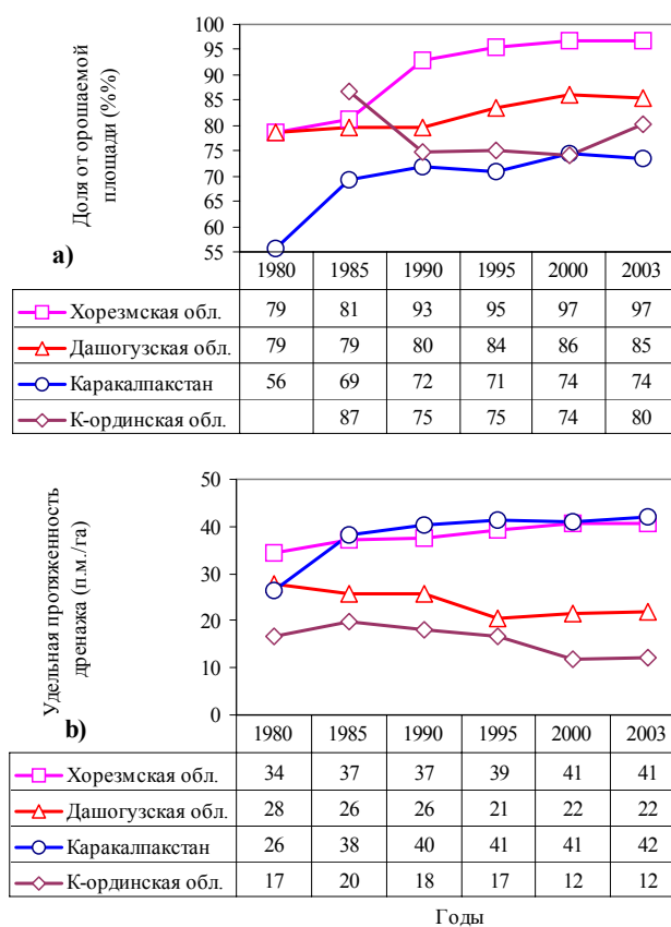
Рис.1.6.4. Обеспеченность дренажем (а) и удельная протяженность дренажа (б)
