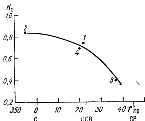
Рис. 6. Связь между коэффициентом ориентации K_0 и преобладающей ориентацией f_{пр} ледников бассейнов левых притоков Сарезского озера и р. Мургаба (1), верховьев рек Сулистьк и Аксу (2), правых притоков р. Мургаба и Сарезского озера (3) и бассейна р. Мургаба в целом (4).
