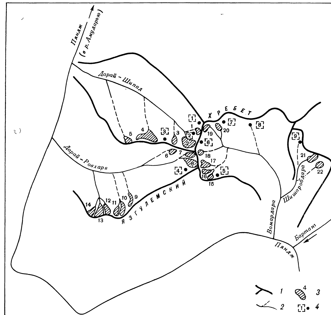
Рис. 20. Схема расположения ледников в бассейнах рек Дарай-Шинд, Дарай-Ровхарв и Вомадара. 1 — хребет, 2 — река, 3 — ледник и его порядковый номер по табл. 1, 4 — ледник размером менее 0,1 км² и его порядковый номер по табл. 39
