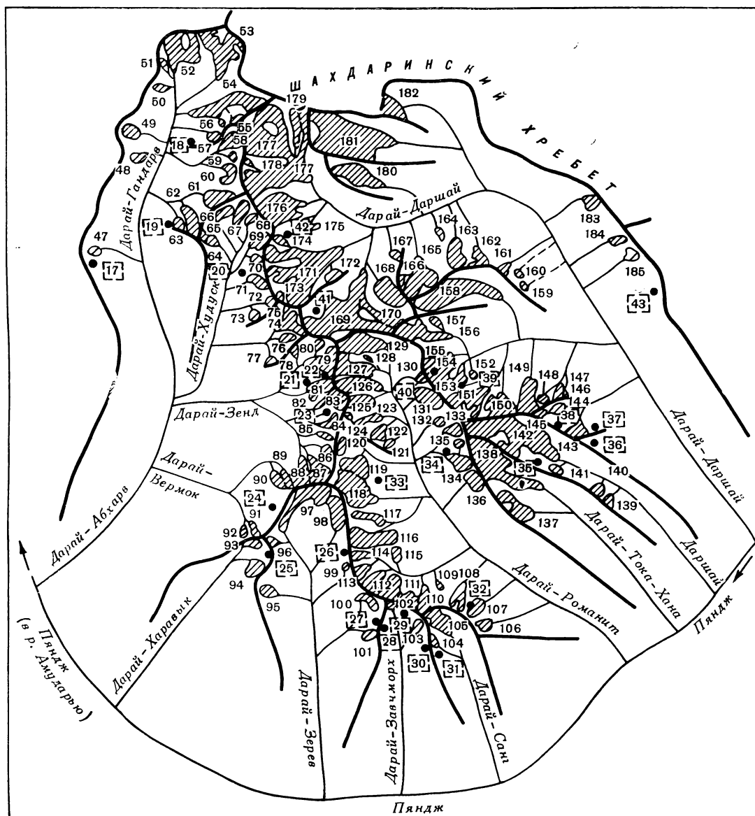
Рис. 11. Схема расположения ледников в бассейнах рек Дарай-Абхарв, Дарай-Харавык, Дарай-Зерев, Дарай-Завчморх, Дарай-Санг, Дарай-Романит, Дарай-Тока-Хана, Даршай и Дарай-Даршай. Усл. обозначения см. на рис. 10.
