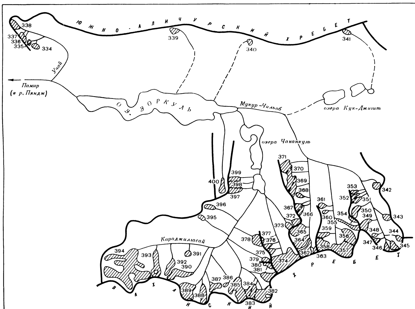
Рис. 15. Схема расположения ледников в бассейнах рек Учай, притоков оз. Зоркуль, рек Мургаб-Чирчик. Караджилгасай. Усл. обозначения см. на рис. 10.
