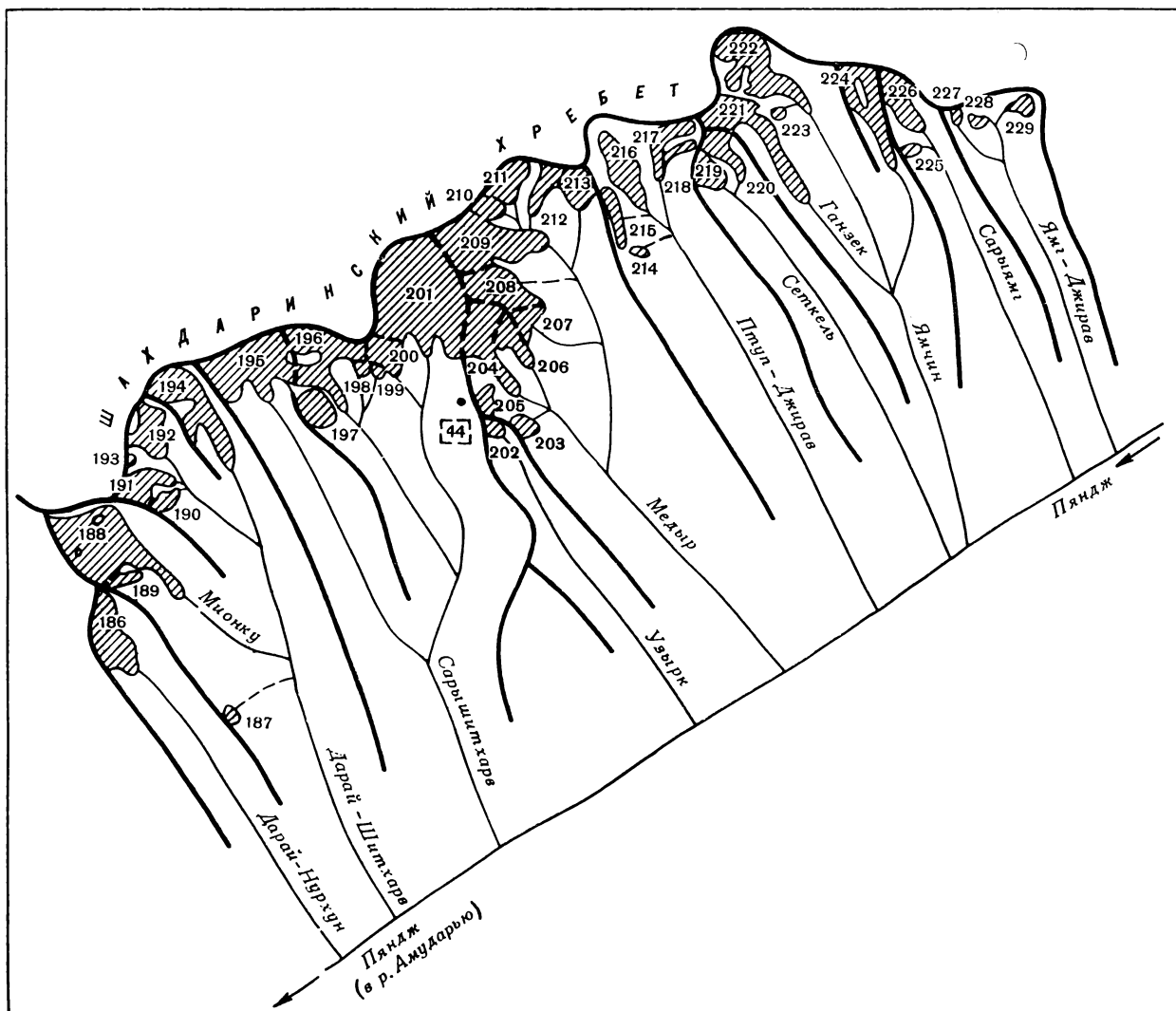
Рис. 12. Схема расположения ледников в бассейнах рек Дарай-Нурхун, Дарай-Шитхарь, Сарышитхарь, Узырк, Медыр, Птуп-Джирав, Сеткель, Ямчин, Сарыямг, Ямг-Джирав. Усл. обозначения см. на рис. 10.
