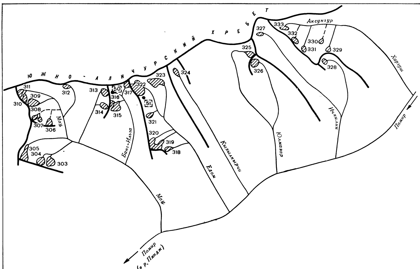
Рис. 14. Схема расположения ледников в бассейнах рек Мац, Едом, Кызылкырчи, Юлмазар, Пчкилик и Харгуш. Усл. обозначения см. на рис. 10.
