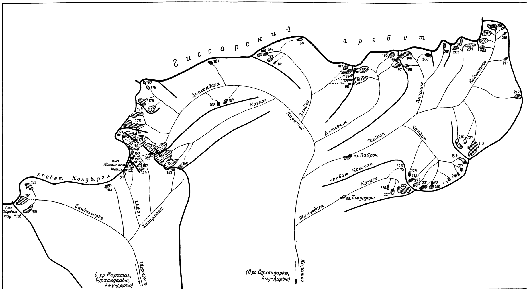
Рис. 14. Схема расположения ледников в бассейнах рек Шеркент и Каратаг.
