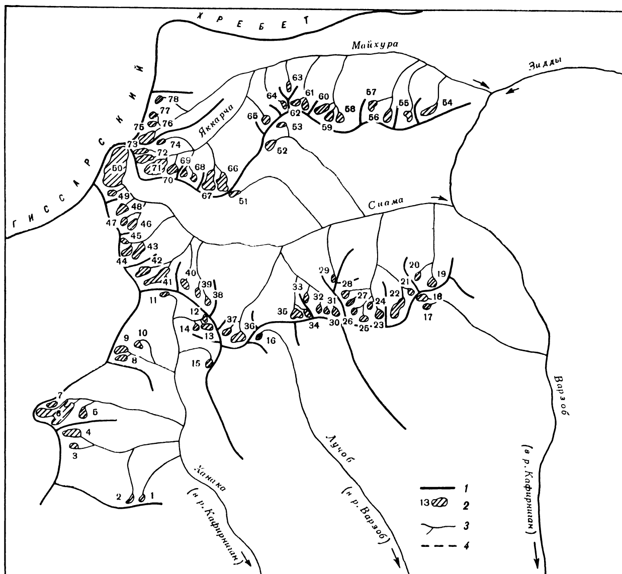
Рис. 8. Схема расположения ледников в бассейнах рек Ханака, Сиамы, Майхуры, Варзоба. 1 — водораздел, 2 — ледник и его номер по табл. 1, 3 — поверхностный сток, 4 — ледораздел
