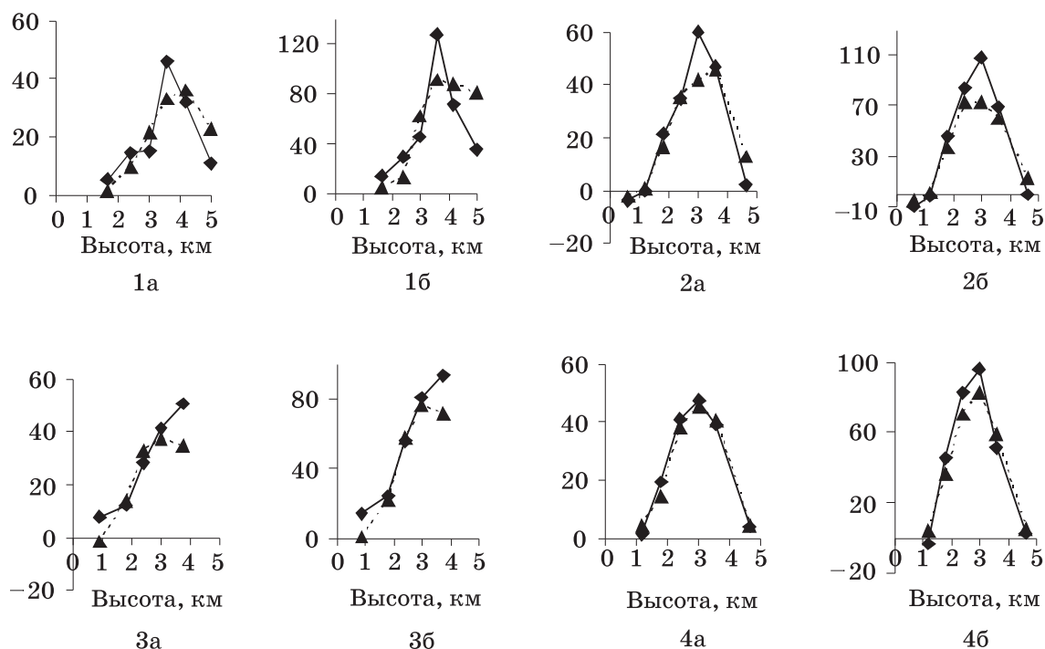
Рис. 2. Величины поясного стока: 1а...4б – районы; ◆ – за период до 1970 года; ▲ – за период после 1970 года; 1а, 2а, 3а, 4а – среднегодовые значения; 1б, 2б, 3б, 4б – средние значения за половодье
