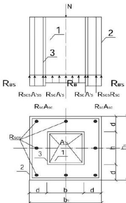
Рис.3.1. Схема центрально сжатого железобетонного элемента, усиленного железобетонной обоймой 1 – усиливаемый железобетонный элемент; 2 – железобетонная обойма; 3 – поверхность сцепления нового бетона со старым (зачистка, насечка, адгезионная обмазка);
