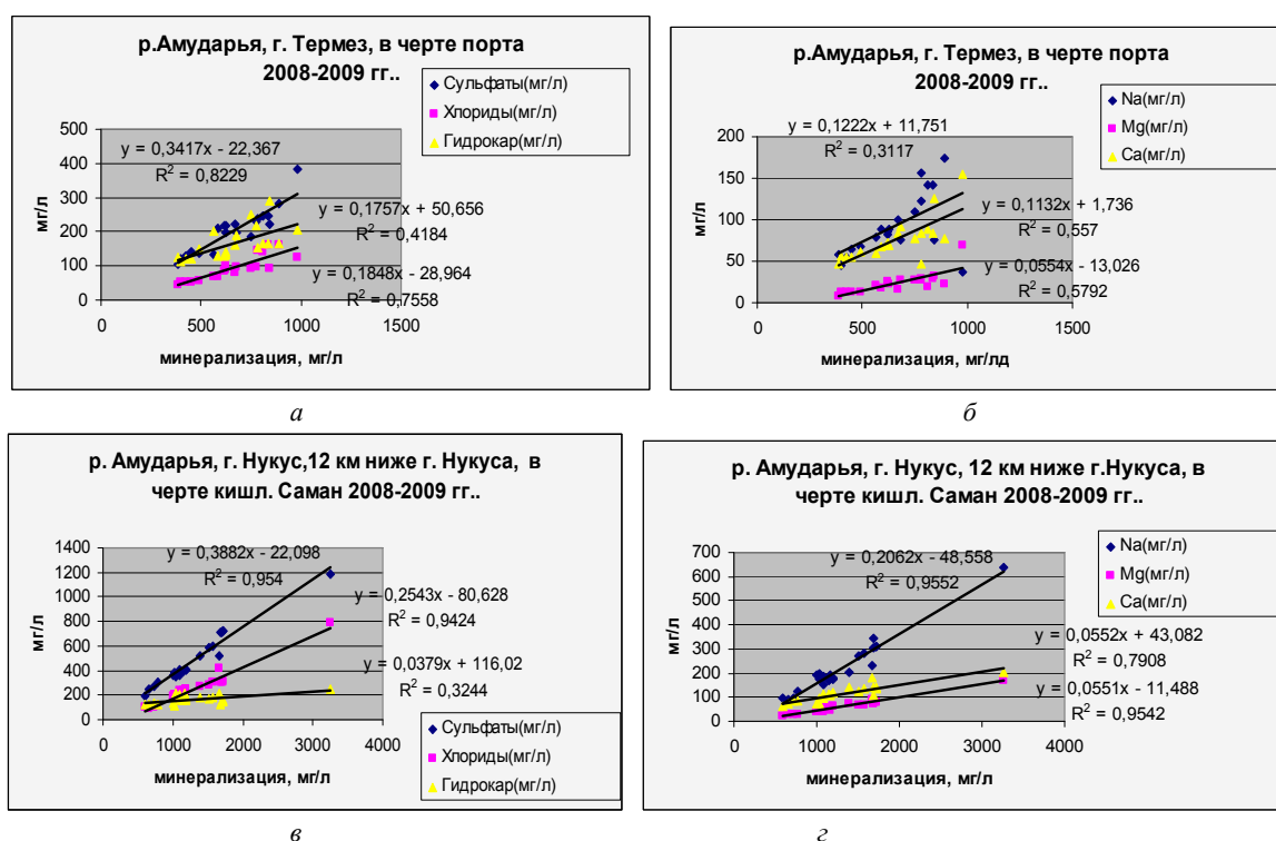
Рисунок 3 – Графики зависимости содержания главных ионов ( \text{Ca}^{2+} , \text{Mg}^{2+} , \text{Na}^{+} , \text{HCO}_3^{-} , \text{Cl}^{-} , \text{SO}_4^{2-} ) от величины минерализации на различных створах р. Амударья
