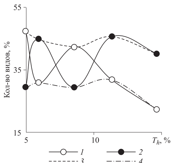
Рис. 3. Зависимость видового богатства обобщенных групп трав (одно-, двулетних и многолетних) от видового богатства группы полудревесных видов растений ( T_h ) по данным 1944–1981 гг.
