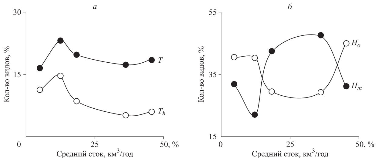
Рис. 1. Зависимость видового богатства обобщенных групп жизненных форм от средних значений речного стока по выделенным временным периодам с 1944 по 1989 г.
