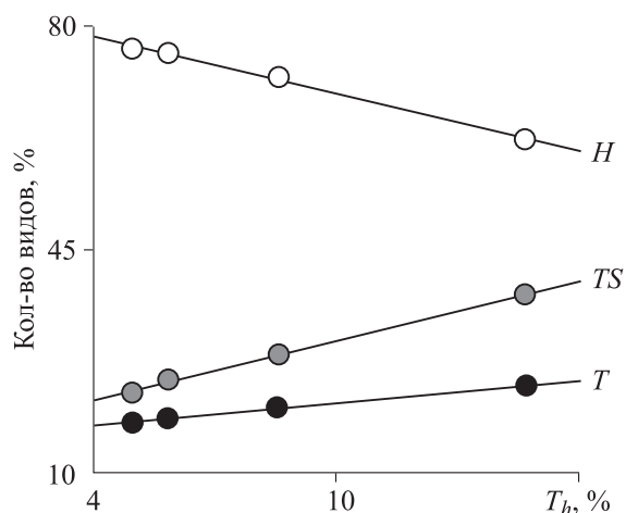
Рис. 2. Зависимость видового богатства обобщенных групп жизненных форм от видового богатства группы полудревесных видов растений ( T_h ) по данным 1944–1989 гг.
