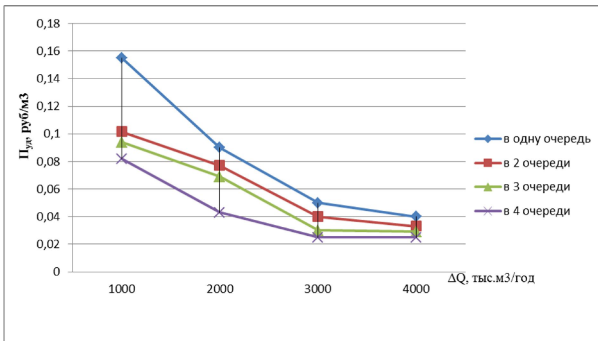
Рис. 4. - Зависимость удельных приведенных затрат на строительство КОС производительностью 64 тыс.м³/сут. от темпов прироста водоотведения при строительстве по очередям
