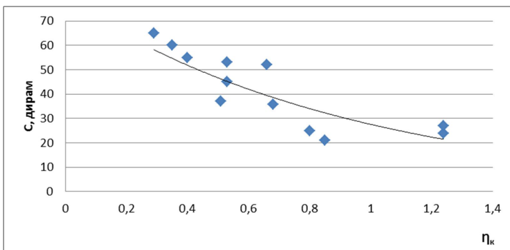
Рис. 2. - Зависимость удельных эксплуатационных затрат в от показателя \eta_k
