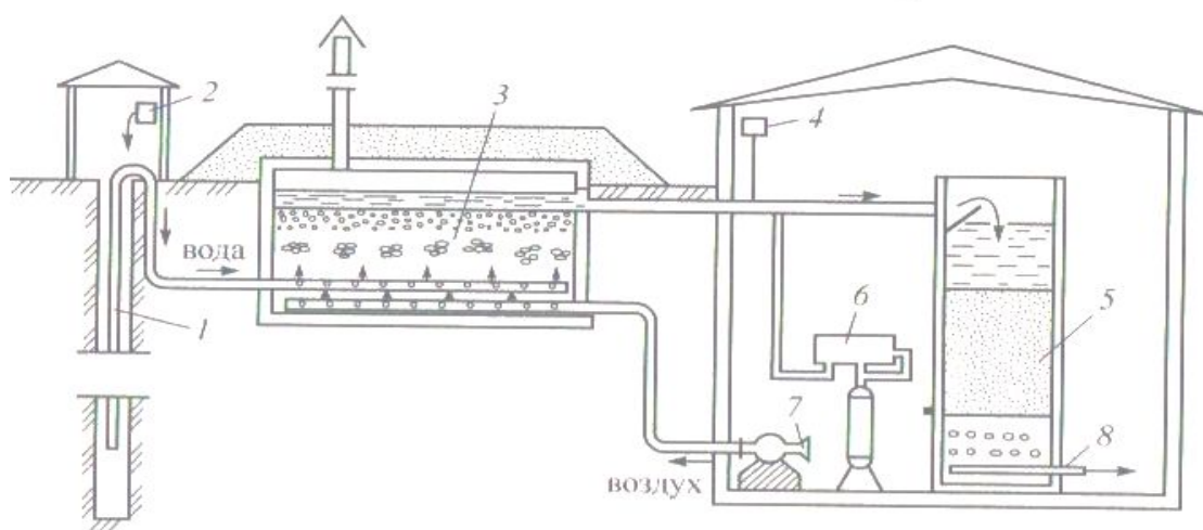
Рис. 5. - Установка биохимического извлечения сероводорода из воды:
