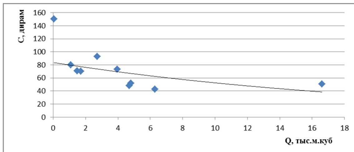
Рис. 3- Зависимость себестоимости от проектной производительности и показателя \Pi_k
