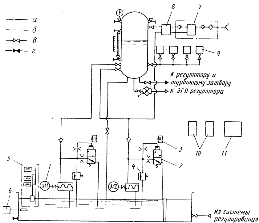
1 – маслоснасос с электроприводом; 2 – клапан пусковой; 3 – бесконтактный датчик положения; 4 – клапан предохранительный; 5 – реле уровня масла; 6 – датчик температуры; 7 – масловоздушный компрессор; 8 – регулятор уровня масла; 9 – реле давления; 10 – станция управления насосами; 11 – масляный трубопровод; 12 – воздушный трубопровод; 13 – клапан нормально открыт; 14 – клапан нормально закрыт
