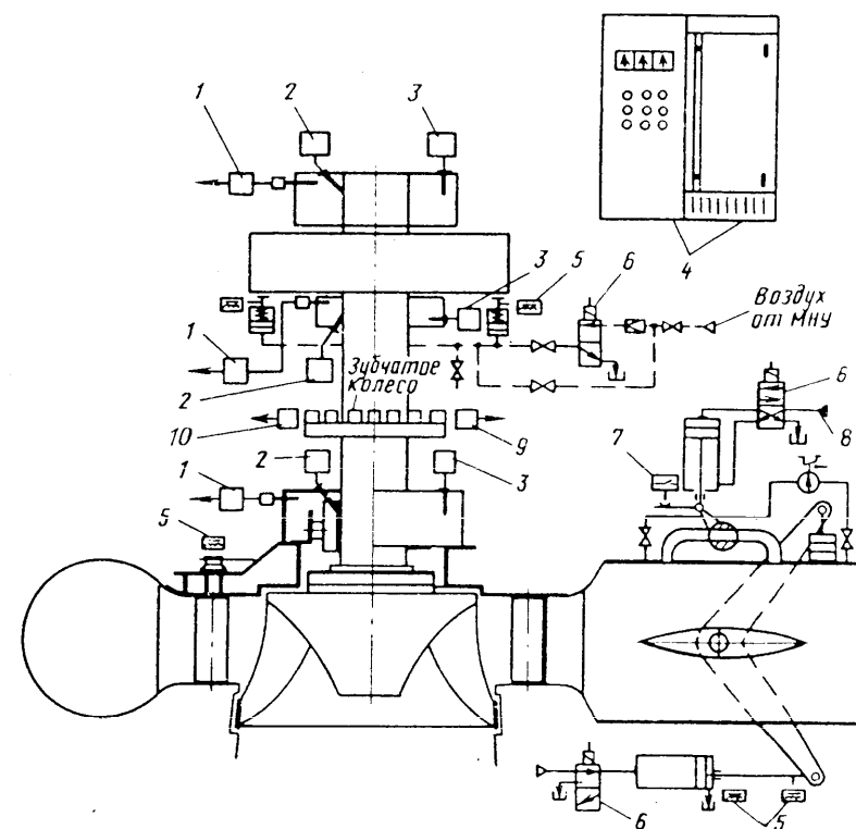
1 – датчик уровня масла; 2 – датчик температуры подшипника; 3 – датчик температуры масла; 4 – панель управления гидроагрегата; 5 – бесконтактные датчики положения; 6 – золотник управления; 7 – контактный датчик положения; 8 – дифманометр; 9 – датчик частоты вращения; 10 – реле частоты вращения
