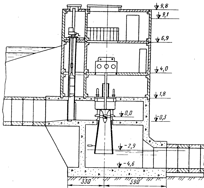
Рис. 3.14. Компоновка здания малой ГЭС с применением сборного железобетона (вариант конструкции)
