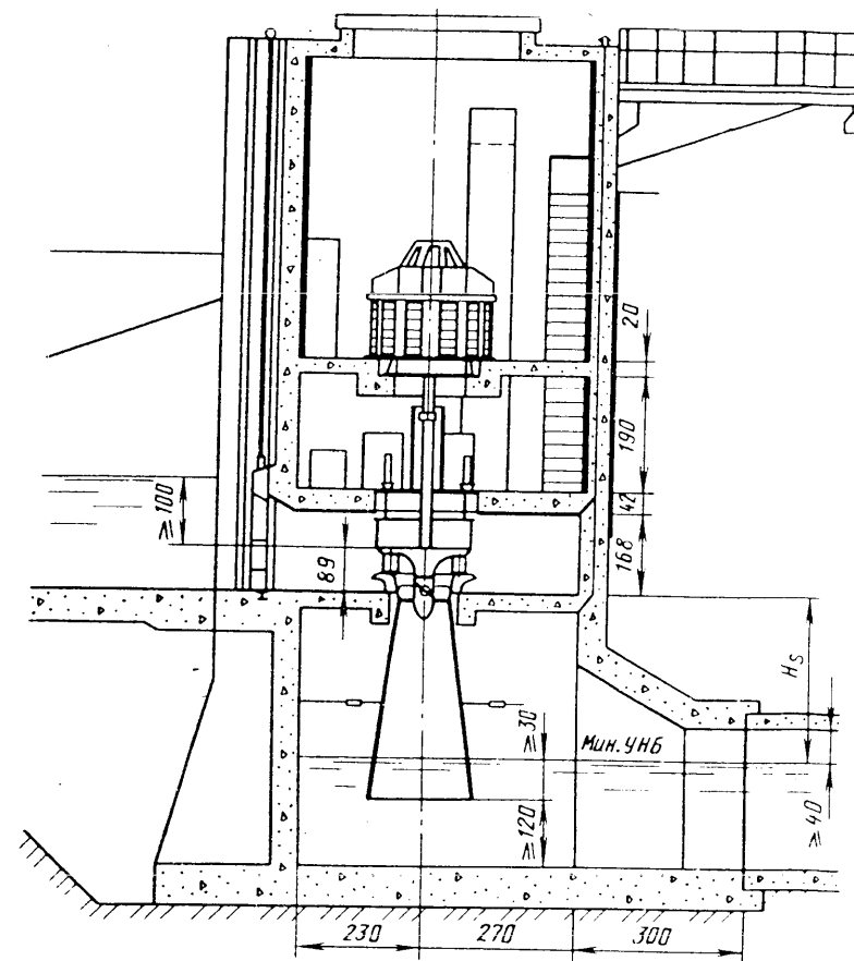
Рис. 3.13. Компонровка здания малой ГЭС с вертикальной осевой гидротурбиной с забором воды непосредственно в турбинную камеру
