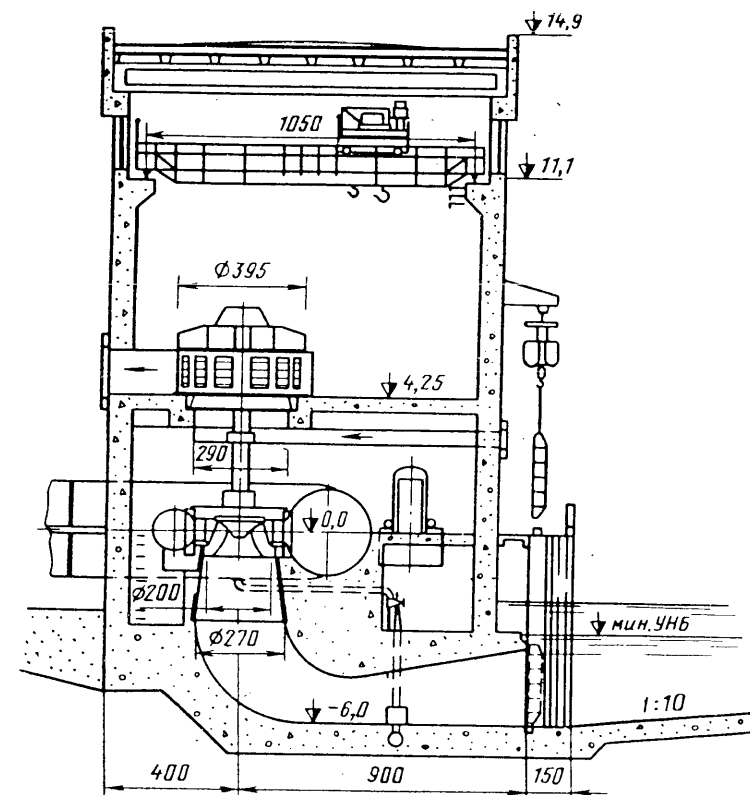
Рис. 3.15. Компоновка здания малой ГЭС с вертикальной радиально-осевой гидротурбиной
