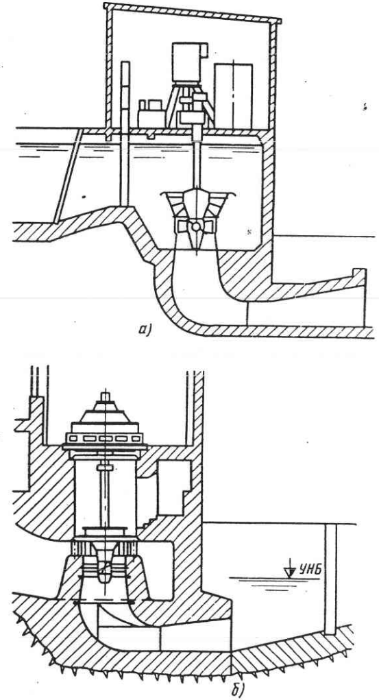
Рис. 7.7. Типовые компоновки агрегатных блоков низковольтных малых ГЭС:
