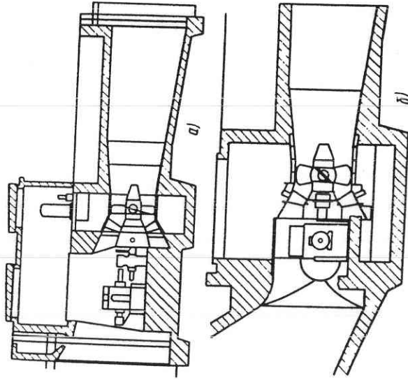
Рис. 7.6. Типовые компоновки агрегатных блоков низковольтных малых ГЭС:
