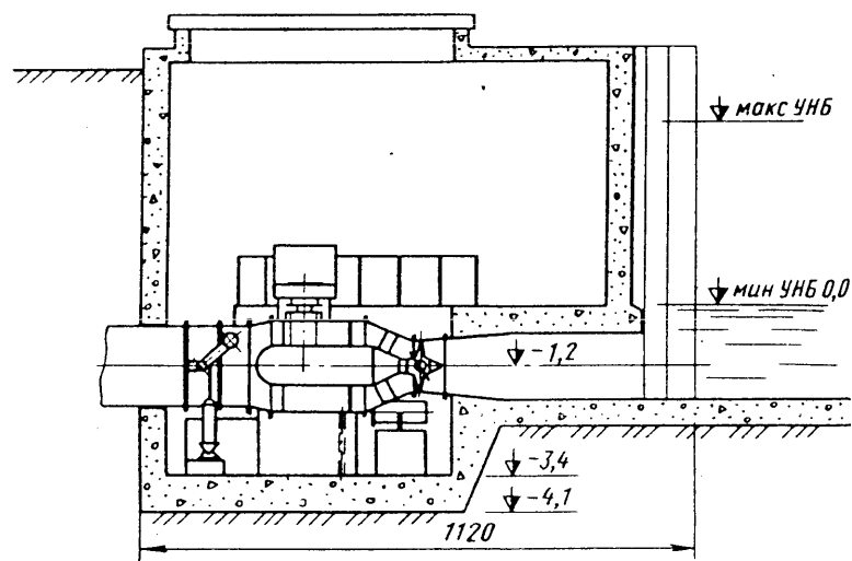
Рис. 3.12. Компонровка здания малой ГЭС с горизонтальной капсульной гидротурбиной и вынесенным в машинный зал вертикальным генератором
