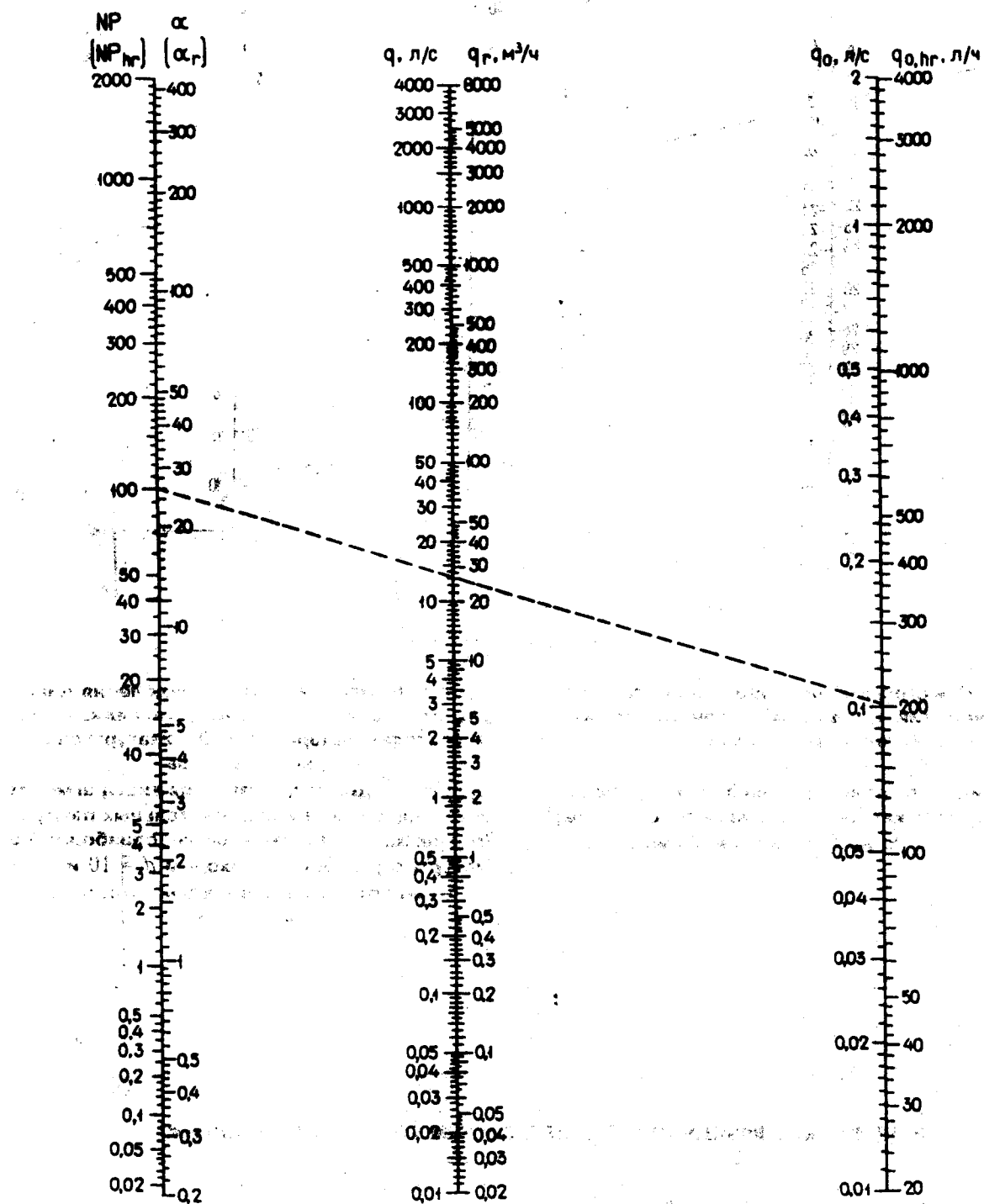
Черт. 4. Номограмма для определения секундных и часовых расходов воды в зависимости от NP ( NP_{hr} ) при различных значениях q_0 , л/с , q_{0,hr} , л/ч
