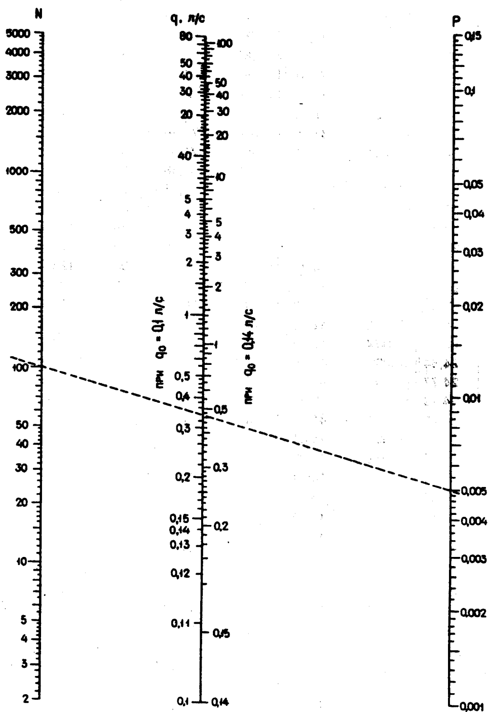
Черт. 1. Номограмма для определения секундных расходов воды q при q_0 = 0,1 и 0,14 л/с и P \leq 0,15
