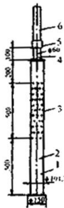
1 - отстойник; 2 - трубка 0-1190; 3 - перфорированная часть, диаметр отверстия 1 мм; 4 - трубка 0-Ц50; 5 - соединительная муфта; 6 - стояк
