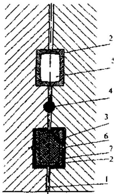
Рисунок К.4 - Восстановление водонепроницаемости уплотнения деформационного шва, выполненного неудаляемыми железобетонными корытами, при наличии обходной фильтрации по контакту железобетонные корыта - бетон сооружения
