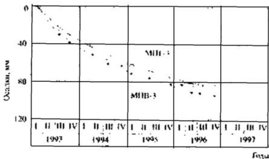
Рисунок Д.4 - График осадки гребня плотины
