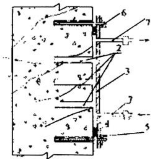
Рисунок Л.3.18 - Принципиальная схема установки для нагнетания цементного раствора
