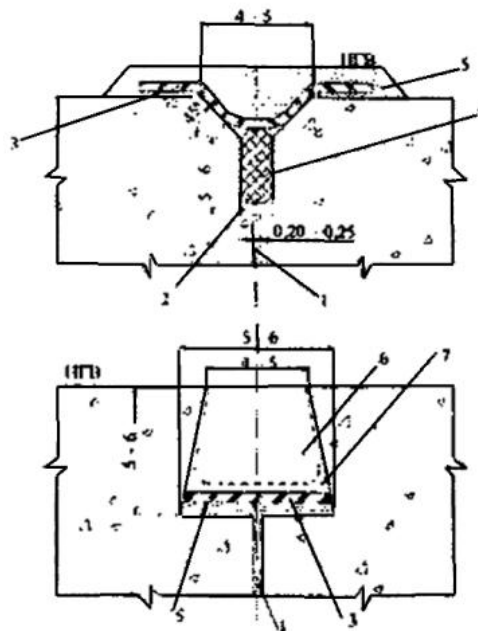
Рисунок Л.3.14 - Уплотнение температурных швов инъекцией
