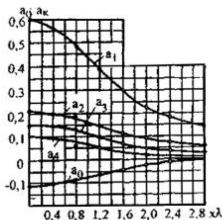
Рисунок E.10 - Графики a_0, a_k для определения скорости
