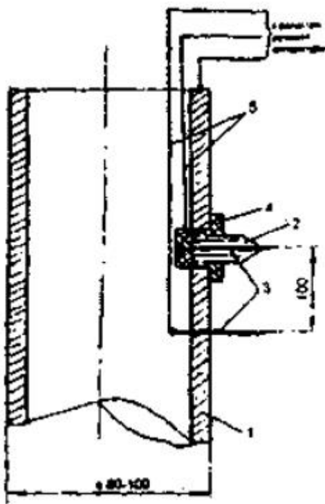
1 - труба стальная; 2 - свеча автомобильная; 3 - центральный электрод; 4 - изолятор; 5 - провода
