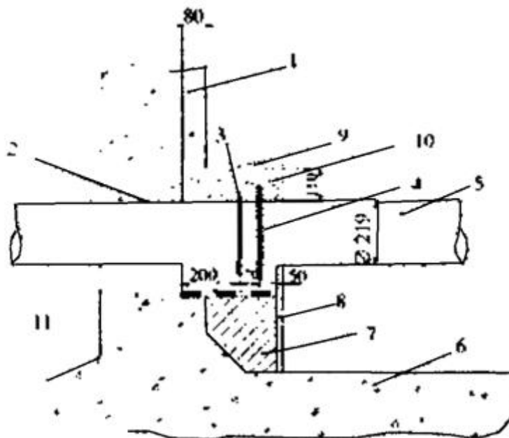
Рисунок Л.3.16 - Ликвидация очага фильтрации в днище
