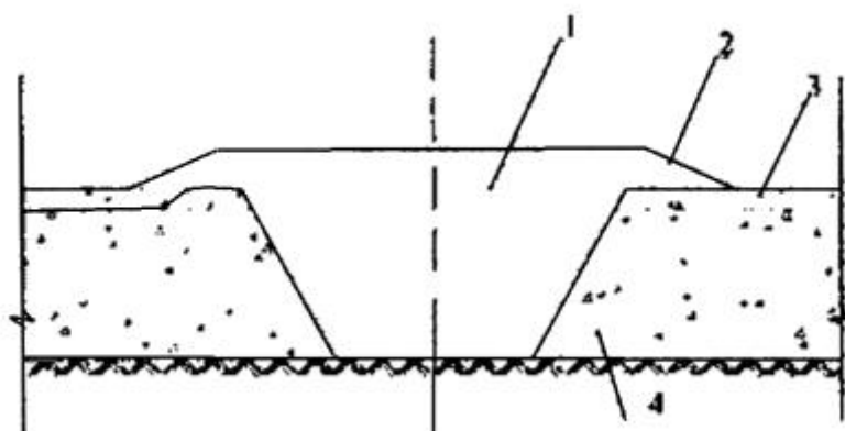
Рисунок Л.3.16 - Ликвидация очага фильтрации в днище
