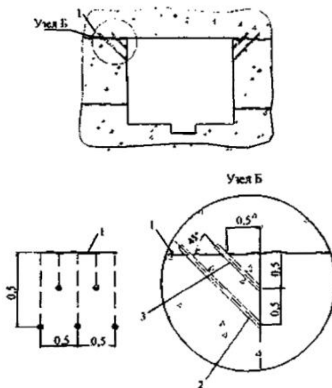
Рисунок Л.3.6 - Уплотнение трещин стен галереи инъекцией
