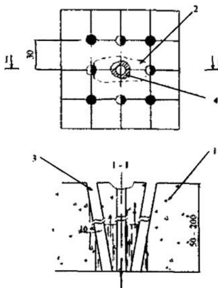
Рисунок Л.3.10 - Тампон-нагнетатель для глубоких скважин
