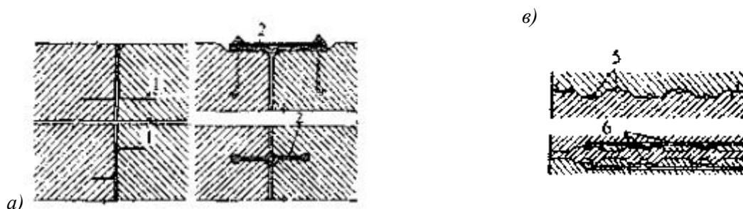
Рисунок К.1 - Схемы расположения уплотнений в постоянных деформационных швах плотин на скальном (а, б) и нескальном (в, г) основаниях
