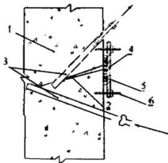
Рисунок Л.3.18 - Принципиальная схема установки для нагнетания цементного раствора
