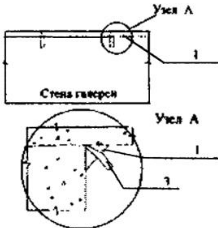
Рисунок Л.3.1 - Схемы расположения скважин при уплотнении фильтрующих трещин и швов
