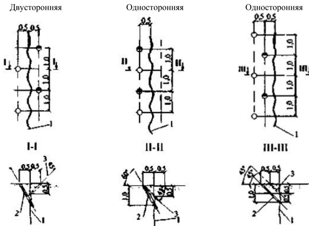
Рисунок Л.3.1 - Схемы расположения скважин при уплотнении фильтрующих трещин и швов
