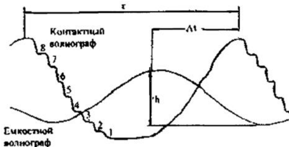
Рисунок Е.7 - Схема волнограммы
