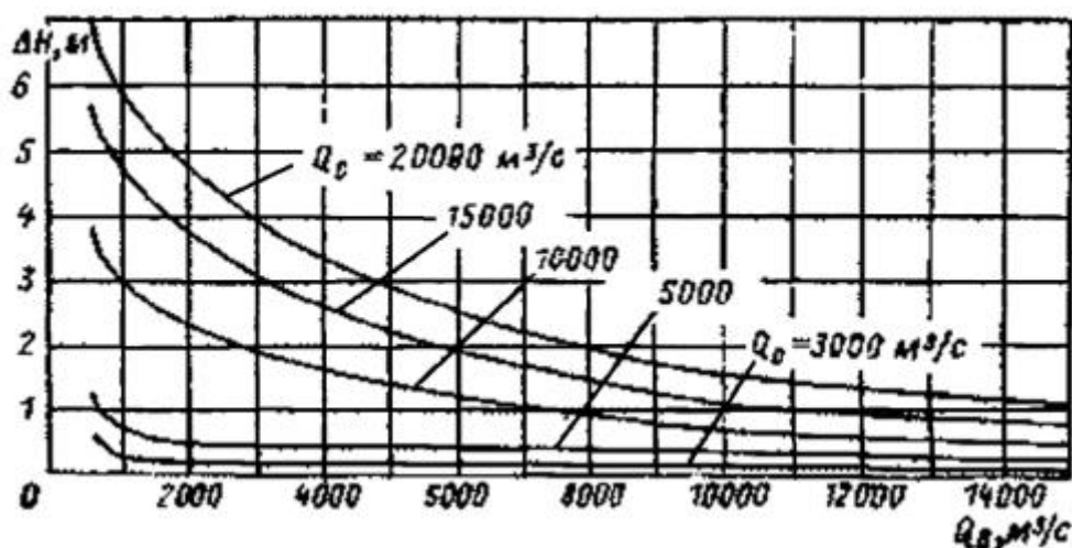
Рисунок И.1.1 - Кривые Q = f(H) в створе Нижегородской ГЭС в зависимости от расхода р. Оки (а) и графики подпора уровня \Delta H при различных расходах Волги Q_o и Оки Q_o (а')
