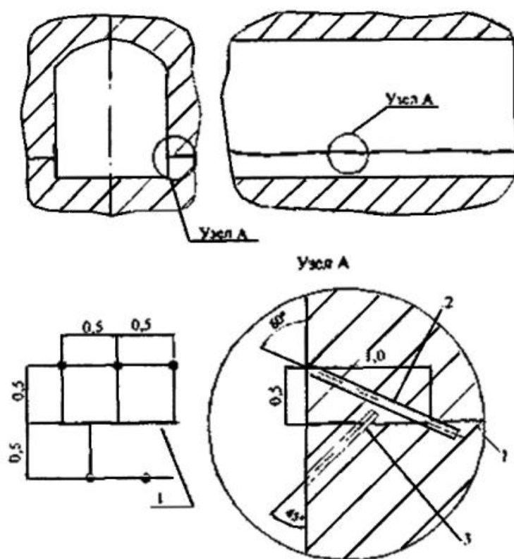
Рисунок Л.3.4 - Уплотнение температурных швов инъекцией
