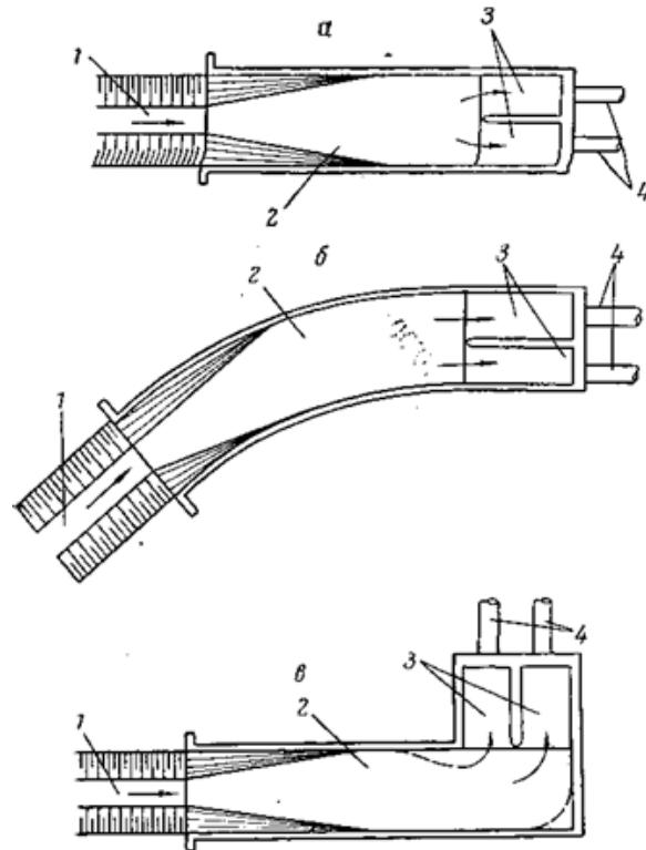
Рисунок 2 – Схемы подвода воды к водопримным камерам напорного бассейна: а – прямолинейный подвод воды; б – криволинейный подвод воды; в – подвод воды под углом 90°. 1 – деривационный канал; 2 – аванкамера; 3 – водопримные камеры; 4 – турбинный трубопровод
