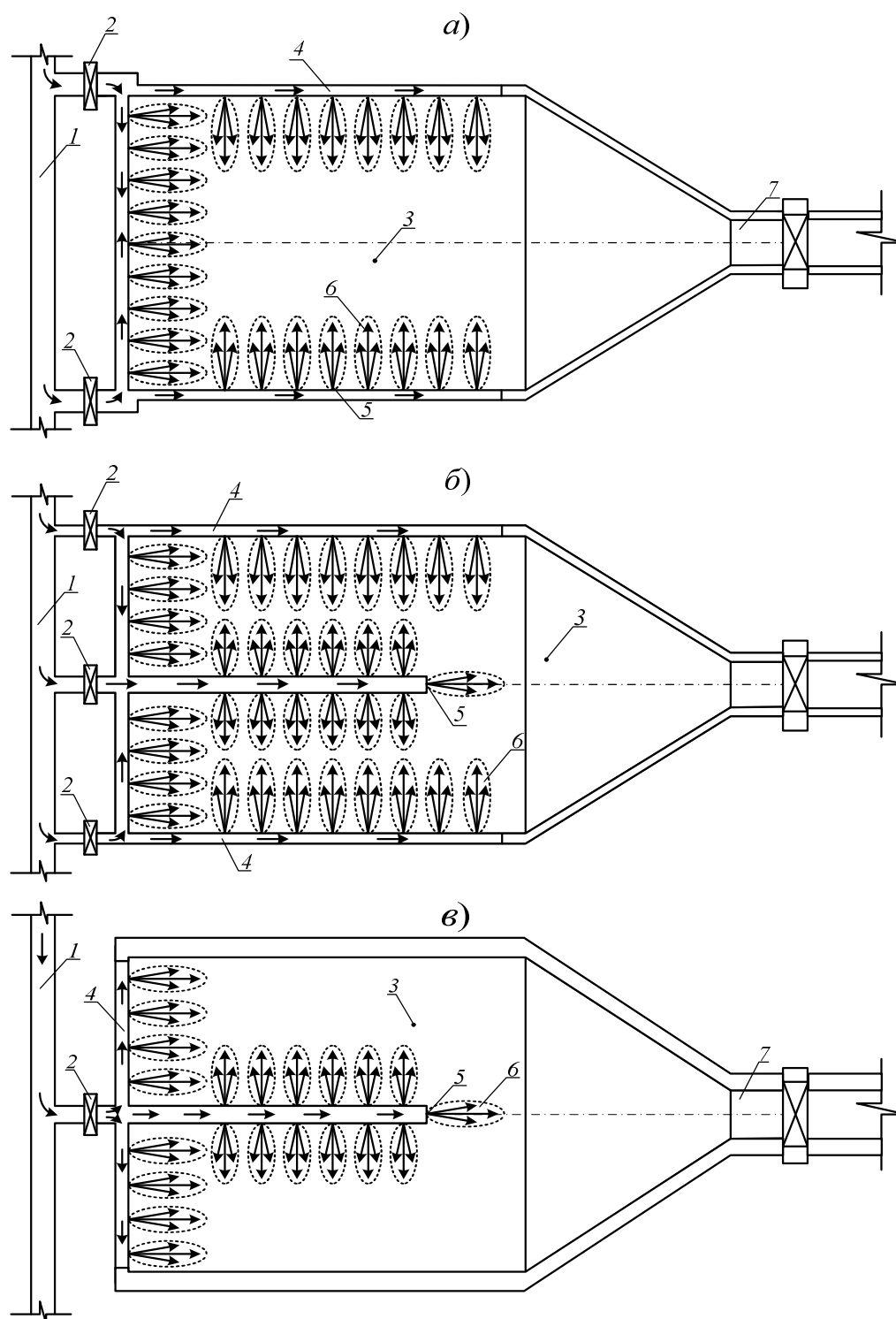
а) схема размещения водоподающих галерей с русловым и береговым их расположением и разделным управлением подачи воды; б) схема размещения водоподающих галерей с центральным управлением подачи воды; в) схема размещения водоподающих галерей с центральным управлением подачи воды; 1 – подводящий водовод; 2 – затвор; 3 – рыбоводный бассейн; 4 – водоподающая галерея; 5 – водовыпускное отверстие; 6 – разноскоростной шлейф; 7 – водорыбоспуск
