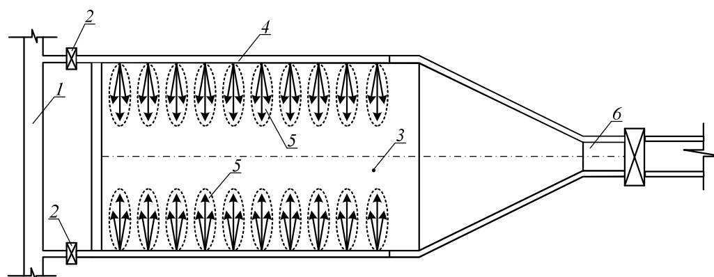
1 – подводящий водовод; 2 – затвор (задвижка); 3 – рыбоводный бассейн; 4 – водоподающая галерея; 5 – водовыпускное отверстие; 6 – водорыбоспуск
