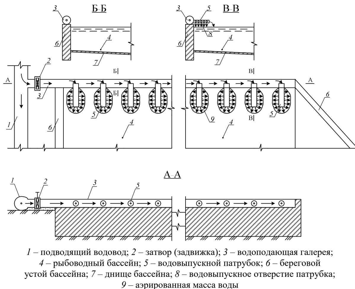
Рисунок 5 – Конструктивно-расчетная схема напорной водоподающей галереи
