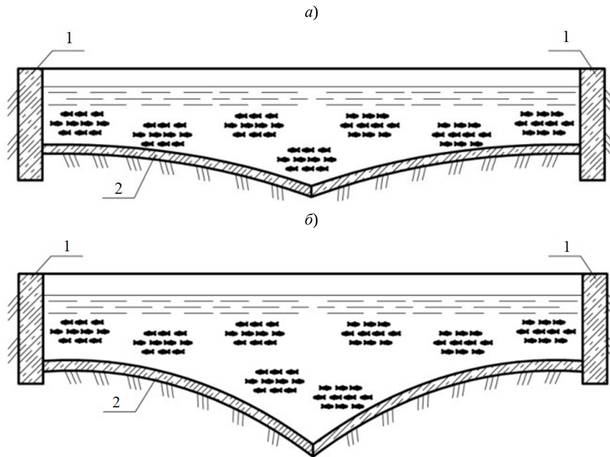
а – поперечный разрез в верховой части бассейна; б – поперечный разрез в низовой части бассейна; 1 – продольный ограждающий устой; 2 – склоновая площадка криволинейного очертания
