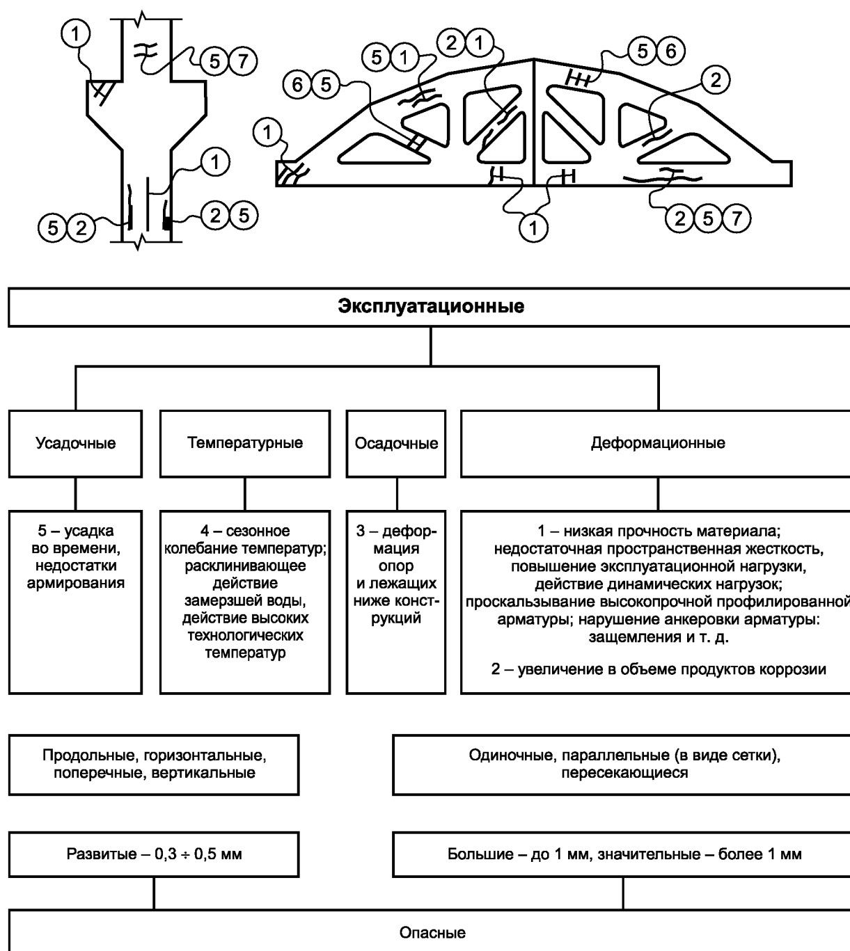
Рисунок К.2 — Эксплуатационные виды трещин
