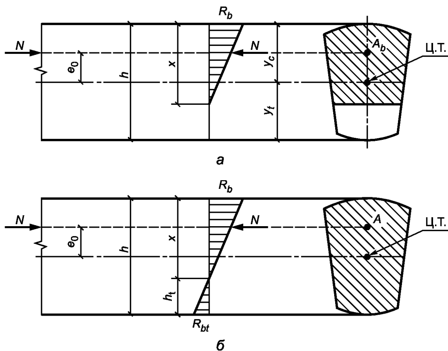
a — без учета сопротивления бетона растянутой зоны сечения; b — с учетом сопротивления бетона растянутой зоны сечения
