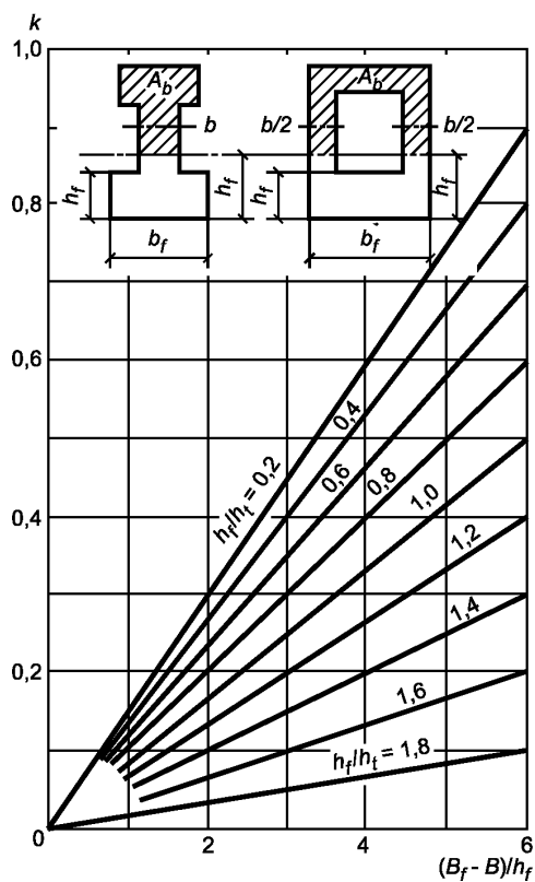
Рисунок Г.1 — Номограмма для определения коэффициента k
