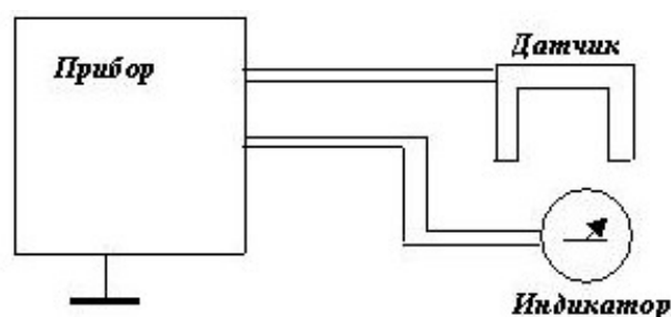
Рис. 1 Блок-схема присоединений к прибору датчика-индуктора и микроамперметра-индикатора.
