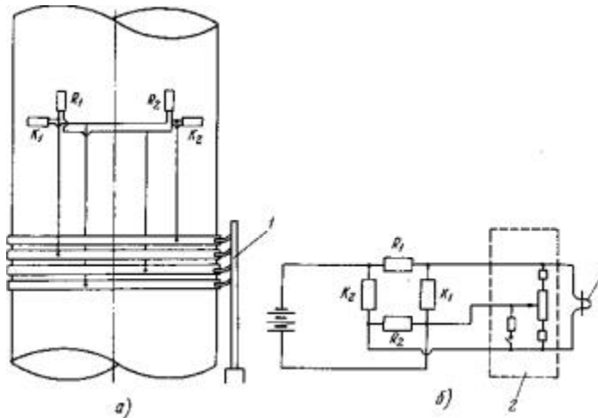
Рис. 1. Схемы измерения осевого усилия на валу:
