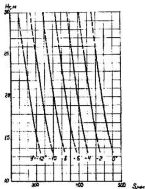
Рис. 26. Графики линий равных углов в координатах H_T - S
