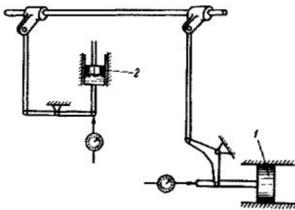
Рис. 7. Схема для определения мертвого хода в рычажной системе обратной связи:
