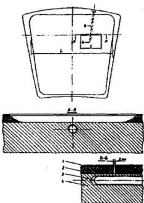
Рис. 6. Выполнение пазов на ЭМП-сегментах для повышения чувствительности термоконтроля:
