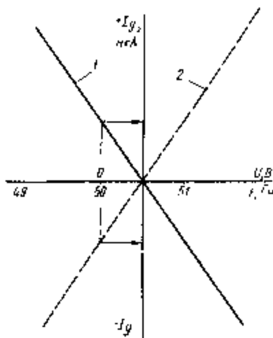
Рис. 9. Характеристика МИЧ (МИО) и ЧЧЭ:
