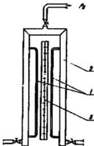
Рис. 7. Схема дифманометра с трубами большого диаметра: 1 - стеклянные трубки; 2 - металлические трубки; 3 - шкала
