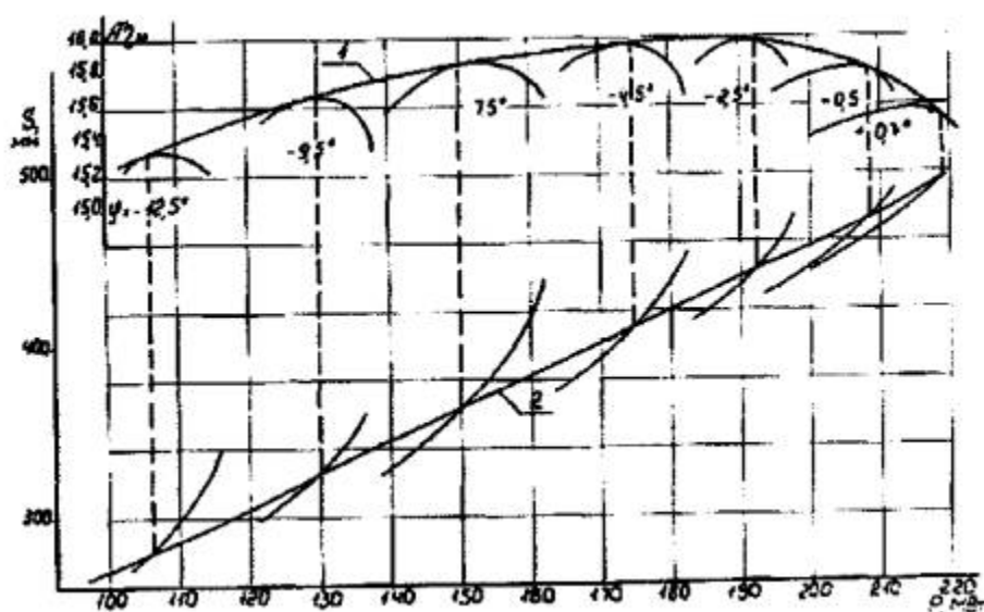
Рис. 25. Графики для определения координат оптимальной комбинаторной зависимости
