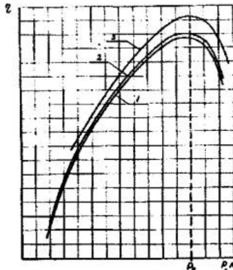
Рис. 19. Рабочие характеристики гидротурбинного блока (1), гидроагрегата (2) и гидротурбины (3)
