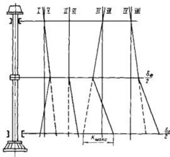
Рис. 4. Пример построения графика состояния линии вала
