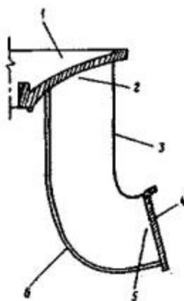
Рис. 1. Схема лопасти рабочего колеса радиально-осевой гидротурбины с указанием основных мест контроля:
