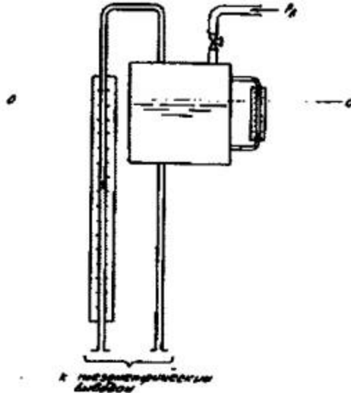
Рис. 6. Чашечный дифманометр
