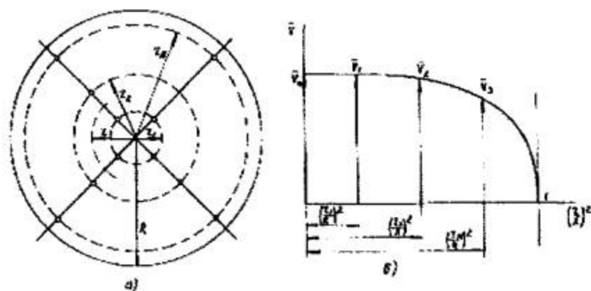
Рис. 14. Графики для определения расхода воды в круглом трубопроводе:
