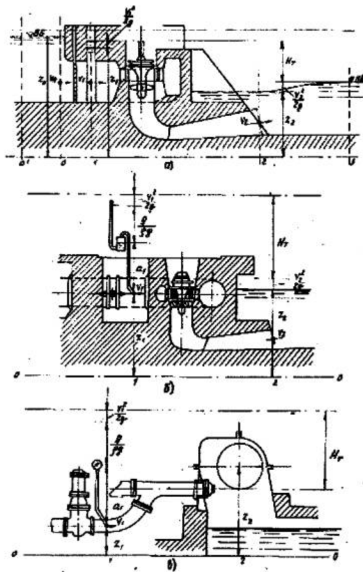
Рис. 2. Схема определения напора:
