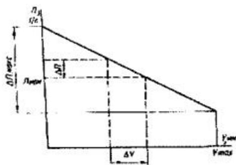
Рис. 5. Статическая характеристика регулятора
