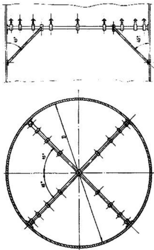
Рис. 11. Стационарная батарея
