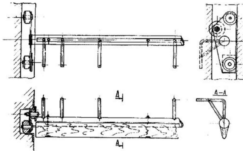
Рис. 9. Однорядная вертушечная рама
