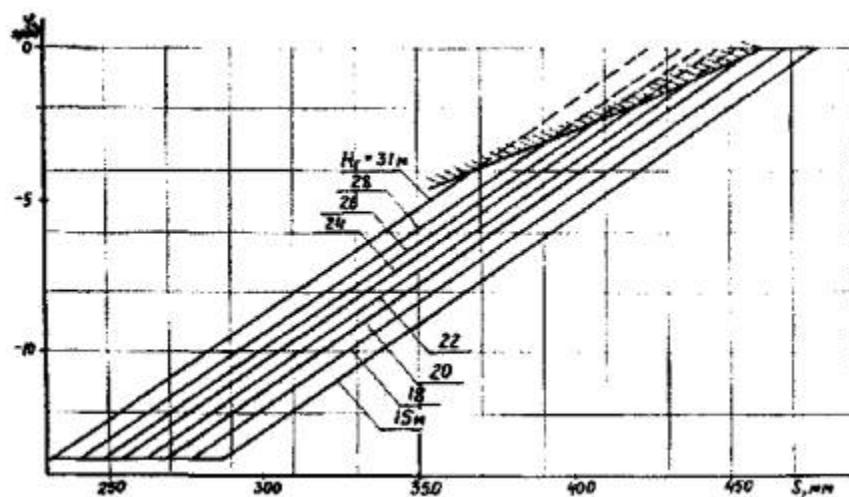
Рис. 27. Оптимальные комбинаторные зависимости для рабочего диапазона напоров
