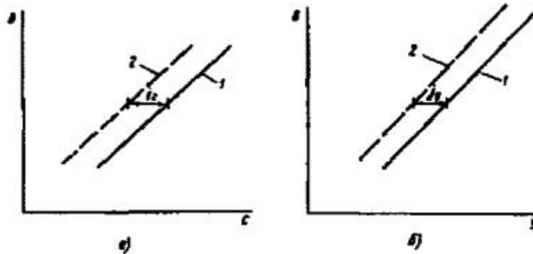
Рис. 15. Статические характеристики системы регулирования для определения мертвой зоны:
