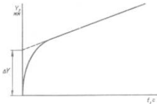
Рис. 2. Переходная характеристика открытия направляющего аппарата
