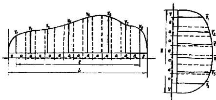
Рис. 13. Эпюры скоростей в мерном створе прямоугольного сечения
