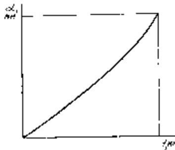
Рис. 12. Кривая зависимости открытия НА от хода штока сервомотора
