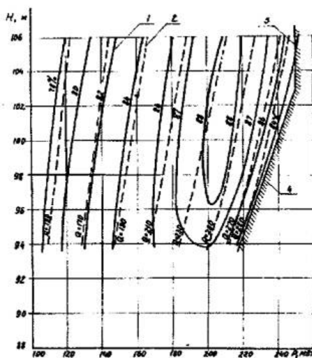
Рис. 21. Эксплуатационная характеристика гидротурбинного блока:
