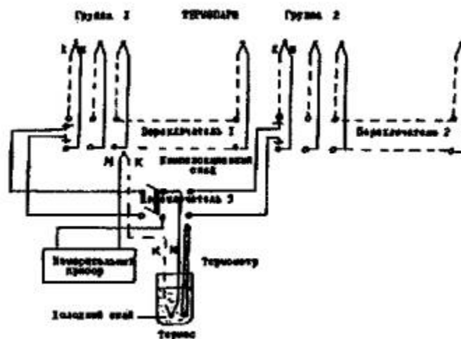
Рис. 1. Схема измерений температуры паяк обмотки статора гидрогенератора при помощи термопар
