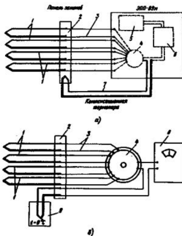
Рис. 6. Схемы подсоединения термопар к потенциометрам:
