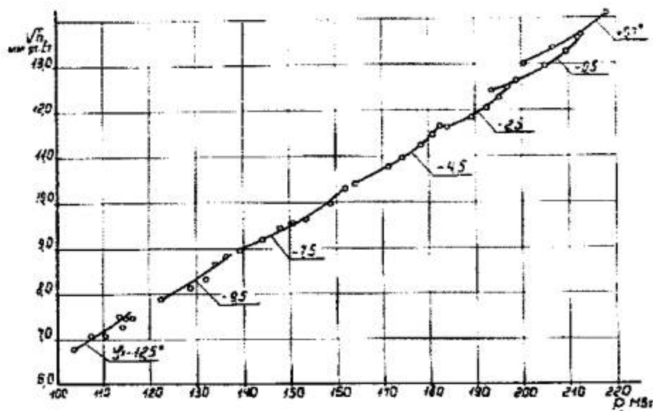
Рис. 24. Пропеллерные расходные характеристики
