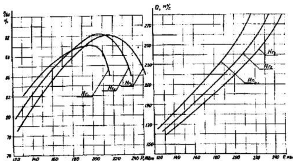
Рис. 20. Рабочие и расходные характеристики гидротурбинного блока для трех напоров
