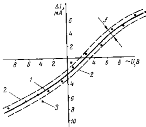
Рис. 10. Характеристика усилителя по входу на Т4:
