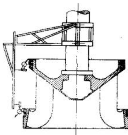
Рис. 2. Приспособление для проверки concentricity
