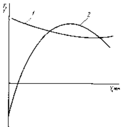
Рис. 13. Примерный вид характеристики перестановочных усилий сервомотора НА:
