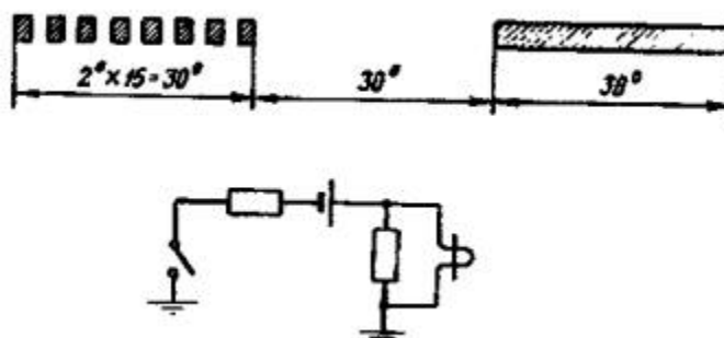
Рис. 8. Схема наклейки меток на валу и электрическая схема измерений угла поворота ротора при пуске
