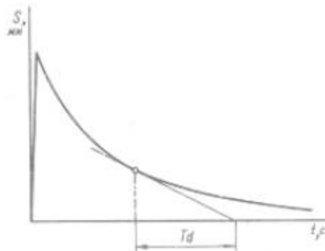
Рис. 3. Переходная характеристика изодрома
