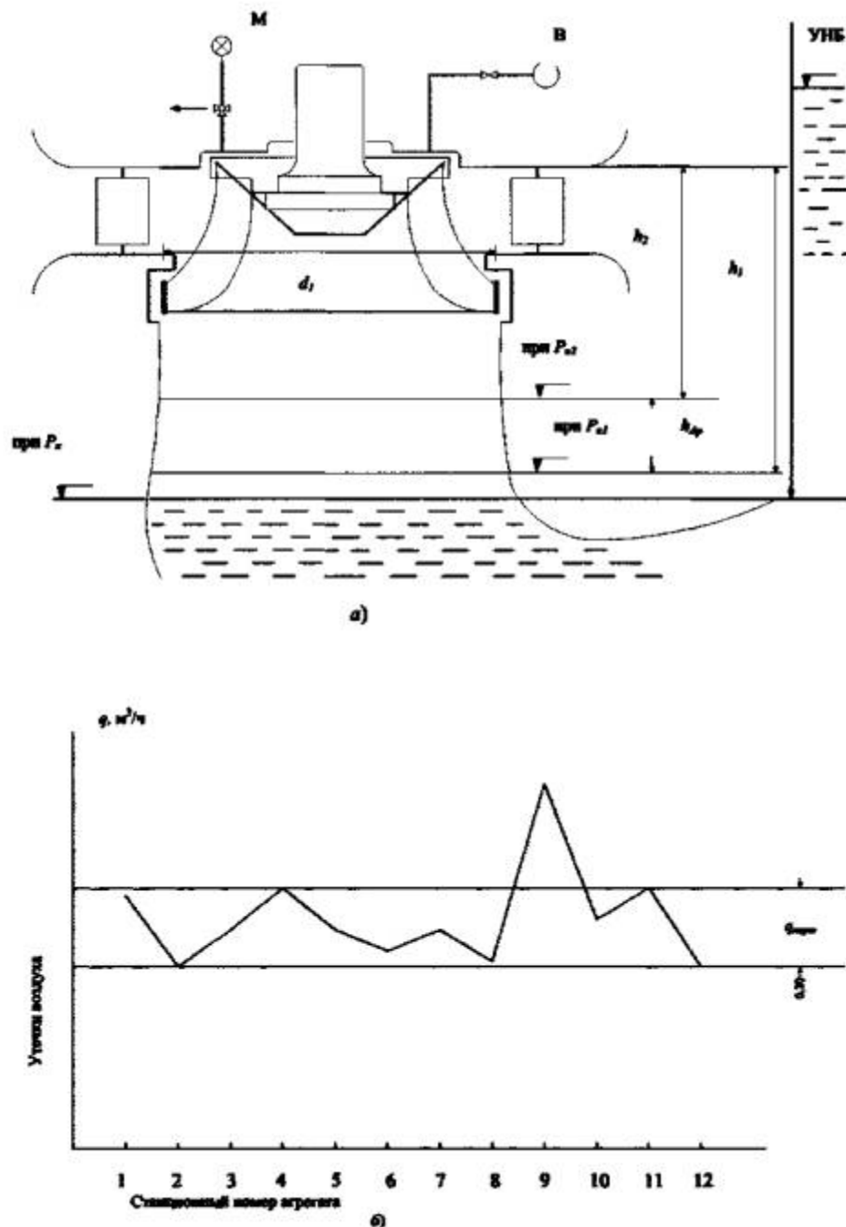
Рис. 1. Контроль утечки воздуха из камеры рабочего колеса турбины при работе в режиме СК:
