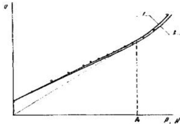
Рис. 18. Расходная характеристика гидроагрегата (1) и турбины (2)
