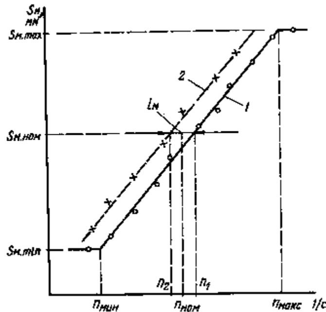
Рис. 1. Статическая характеристика маятника с зоной нечувствительности
