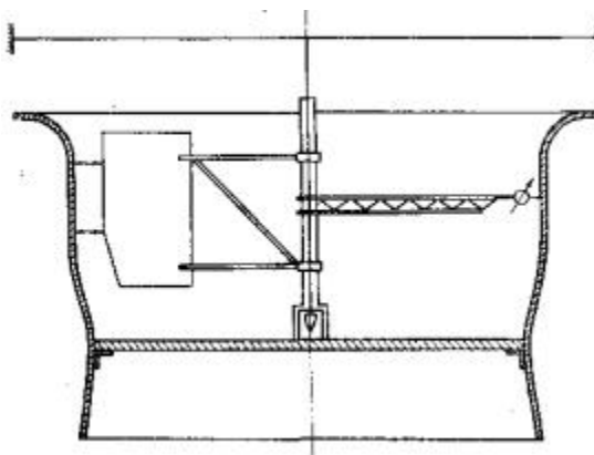
Рис. 1. Проверка размеров камеры рабочего колеса с помощью струны
