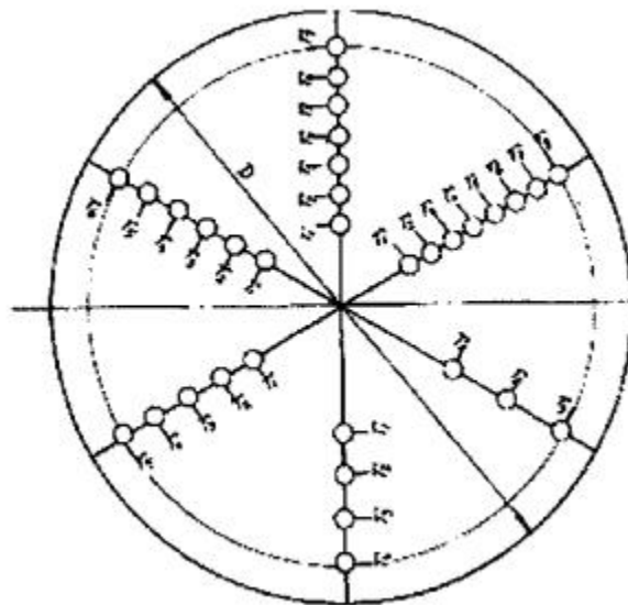
Рис. 10. Схема расположения вертушек в круглом трубопроводе
