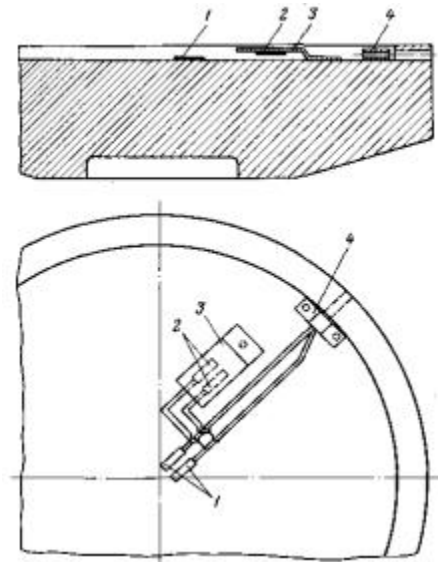
Рис. 2. Расположение тензометров на опорной тарелке:
