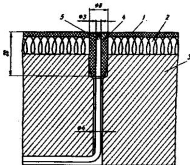
Рис. 5. Установка термопары на поверхности ЭМП-сегмента:
