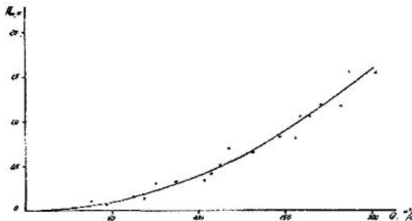
Рис. 16. График зависимости потерь напора в турбинном водоводе от расхода воды
