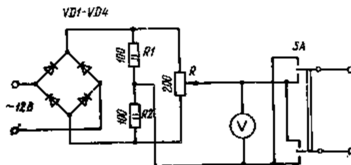
Рис. 16. Электрическая схема сигналов задания
