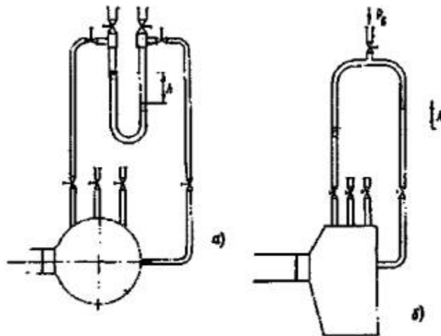
Рис. 5. Схема измерения перепада давления в спиральных камерах турбин с помощью дифманометров:
