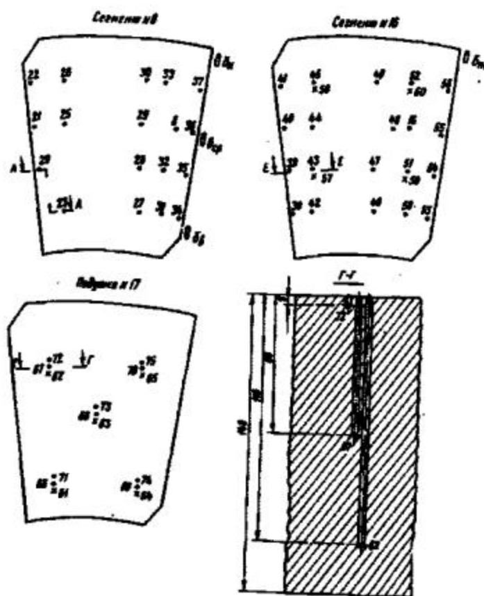
Рис. 4. Расположение точек измерения температуры подпятника агрегата № 6 ДДГЭС:
