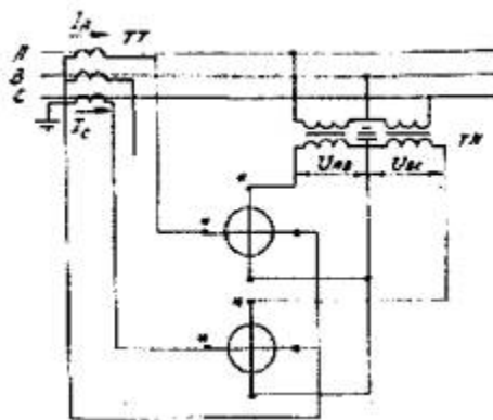
Рис. 4. Схема измерения активной мощности в трехфазных цепях двумя однофазными ваттметрами
