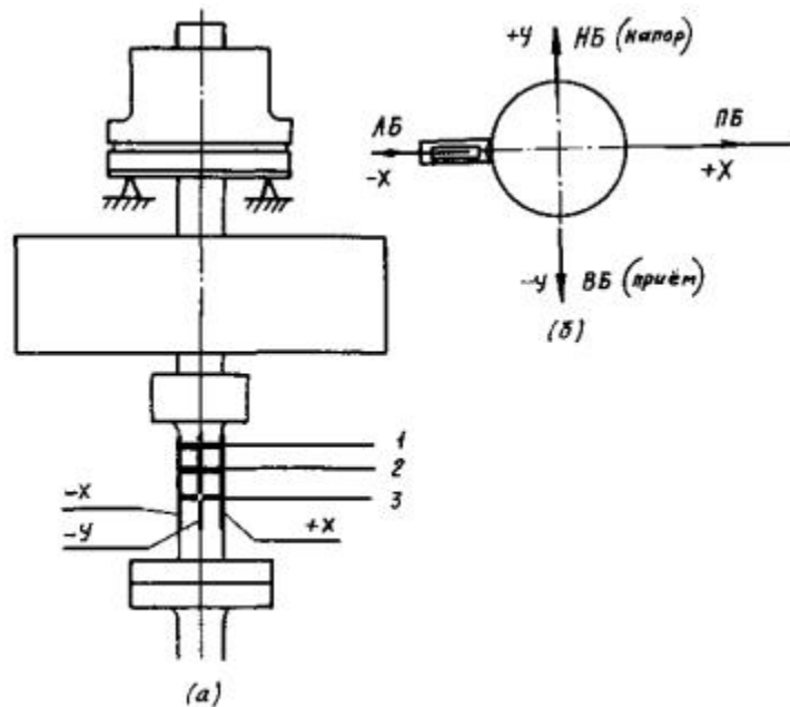
Рис. 5. Разметка вала агрегата для проверки центровки уровнем «Геологоразведка»:
