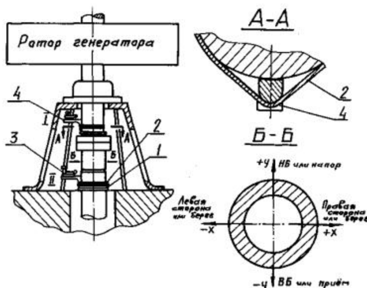
Рис. 7. Ротор генератора:
