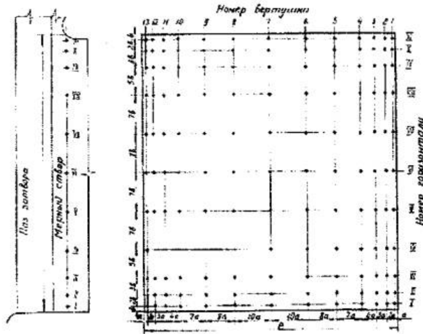
Рис. 8. Пример расположения мерных точек в сечении водовода турбины
