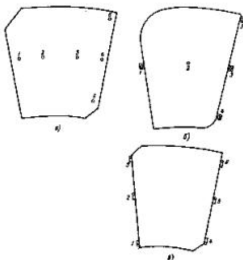
Рис. 3. Различные схемы расположения датчиков толщины масляной пленки в сегментах
