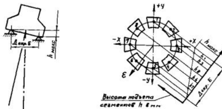
Рис. 8. Схема регулировки высоты элементов подпятника для устранения уклона линии валов
