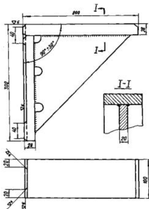
Рис. 6. Уголок для проверки линии валов с помощью уровня
