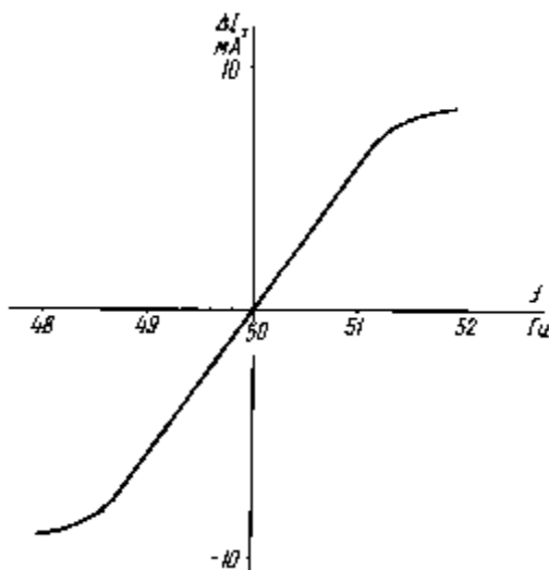
Рис. 8. Характеристика усилителя по входу частоты
