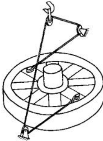
Рис. 3. Симметричный способ поворота ротора гидроагрегата
