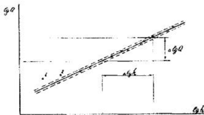
Рис. 15. Тарировочная характеристика расходомерного створа спиральной камеры в логарифмических координатах
