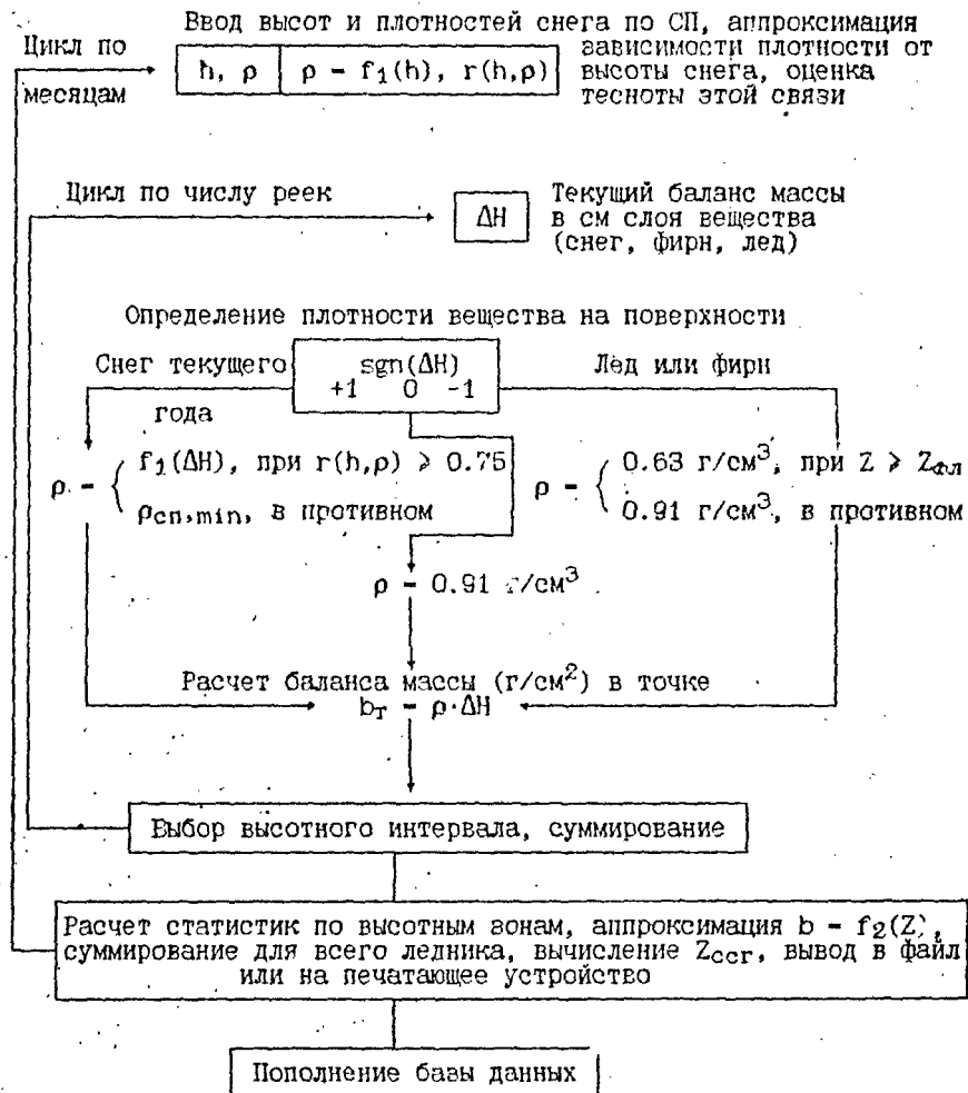
Рис. 2. Блок-схема расчета удельного баланса массы горного ледника
