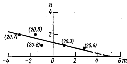
Рис. 92. Связь между показателями степени n при v_*/w_0 и m при C/\sqrt{g} в ряду формул (20.3)—(20.7).
