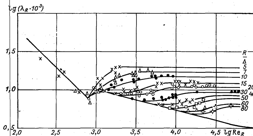
Рис. 13. График сопротивления открытых русел по опытам Зегжды.
