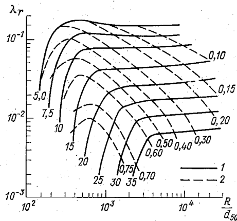
Рис. 36. Функция \lambda_r = \text{fct} \left( \frac{U}{\sqrt{gd_{50}}}, \frac{R}{d_{50}} \right) (по Абу Аламу и Кеннеди).
