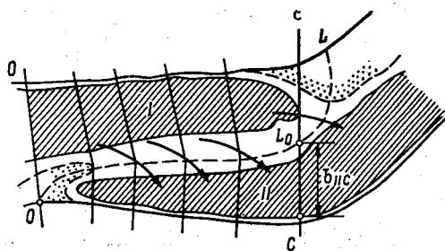
Рис. 47. Фрагменты плана течения на перекате с затонской частью.
