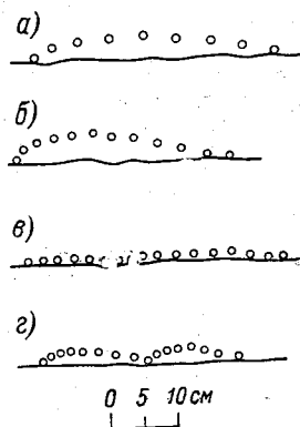
Рис. 77. Траектории подскакивающих частиц (по Россинскому и Любомировой).
