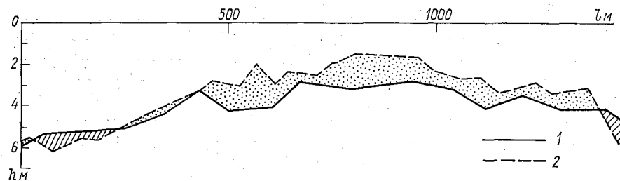
Рис. 101. Продольные профили дна по линии наибольших глубин на В. Желнинском перекате р. Оки.
