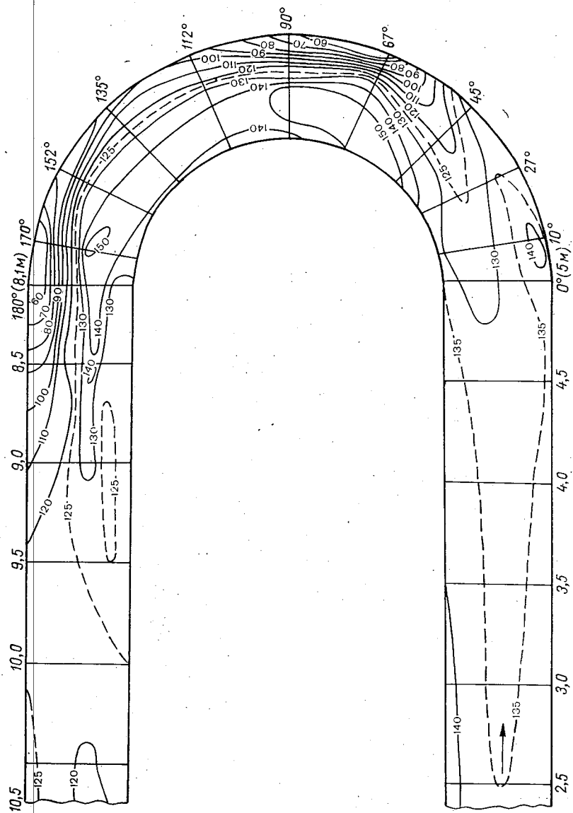
Рис. 64. Рельеф дна, сформированного стационарным потоком ( Q=4 л/с) в лотке с поворотом на 180^\circ (по Власенко).
