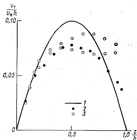
Рис. 12. Распределение коэффициента турбулентной вязкости в плоском напорном потоке.
