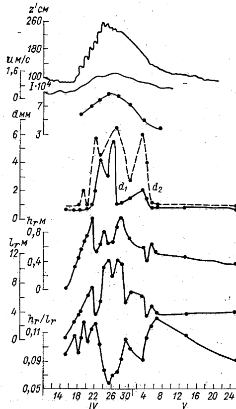
Рис. 89. Изменение параметров потока и размеров гряд во время паводка на р. Полометь (по Снитченко).
