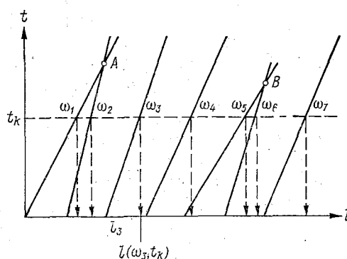
Рис. 93. К интегрированию уравнения деформации способом характеристик.
