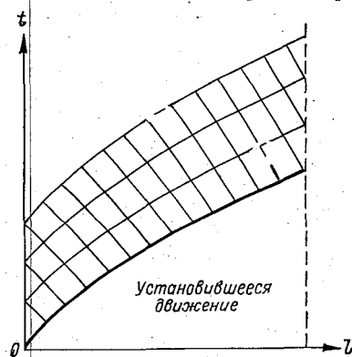
Рис. 39. Сетка характеристик.
