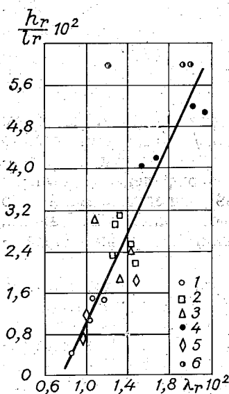
Рис. 34. Сопротивление грядового дна на речных порогах (по Смирнову).
