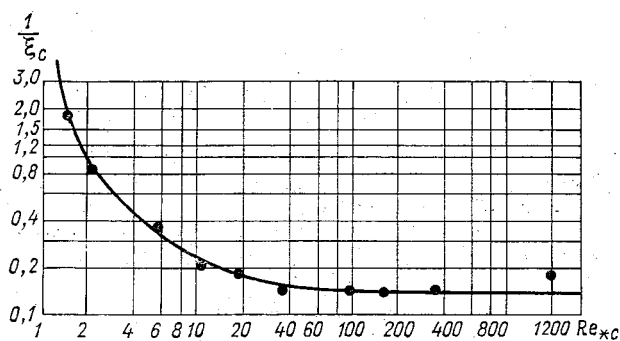
Рис. 76. Функция 1/\xi_c = fct(Re_{*c}) , по Кнорозу.
