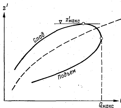
Рис. 40. Неоднозначная связь между расходом и уровнем при резком колебании расхода.
