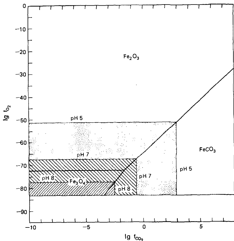
Р и с. 11.14. Зависимость соотношений устойчивости в системе Fe - O - H_2O - CO_2 при 25°C от \lg f_{O_2} и \lg f_{CO_2} . Затененные области — поля устойчивости Fe^{2+} (с активностями, превышающими 10^{-6} ) при различных значениях pH.
