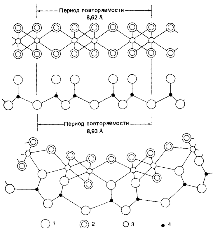
Р и с. 4.4. Схема, показывающая, как несогласованность между октаэдрическим и тетраэдрическими слоями вызывает изгиб решетки, приводящий к трубочатой структуре гаптуазита. 1 — кислород; 2 — гидроксип; 3 — апюминий; 4 — кремний.
