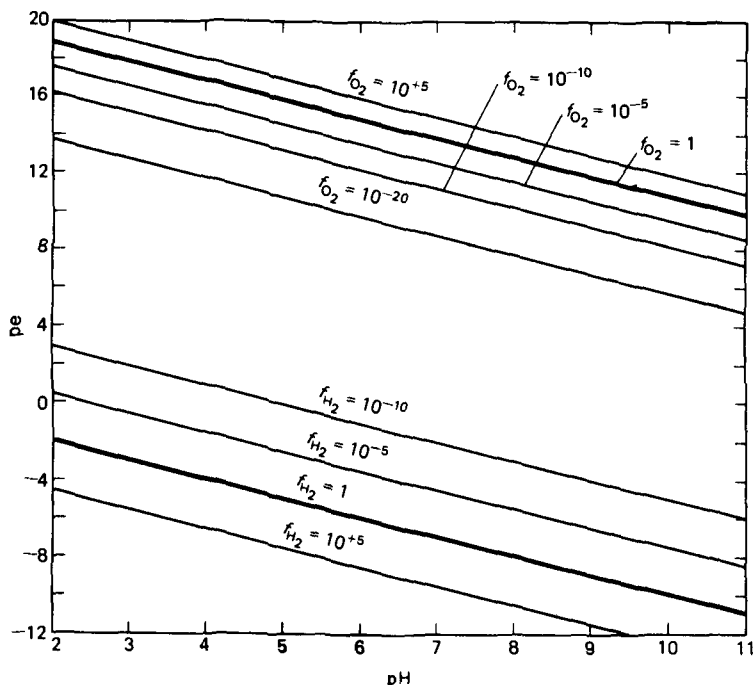
Р и с. 11.3. Линии равных петучестей кислорода и водорода в зависимости от p_e и pH при 25^\circ\text{C} .
