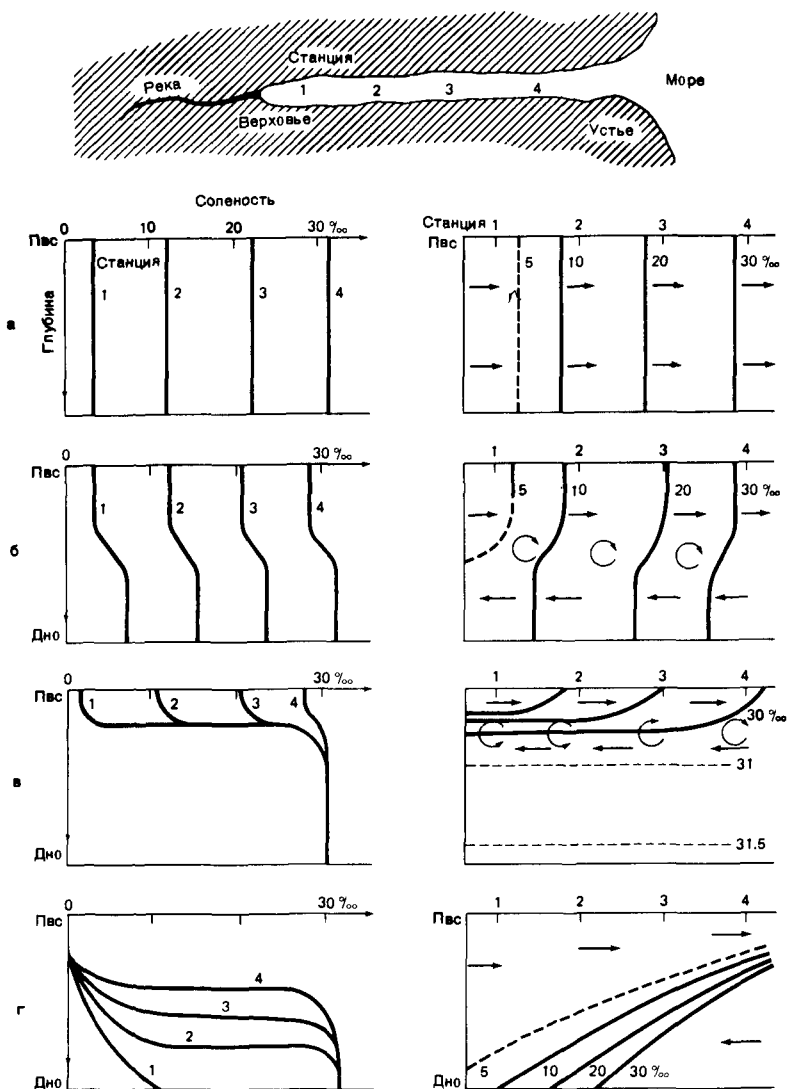
Р и с. 10.3. Типичные профили соленость — глубина в эстуарии вертикального смешения (а), слабостратифицированном (б), высокостратифицированном (в), с солевым клином (г). Контурные справа — соленость (в г/кг); Пвс — поверхность (по Пикарду [270]).
