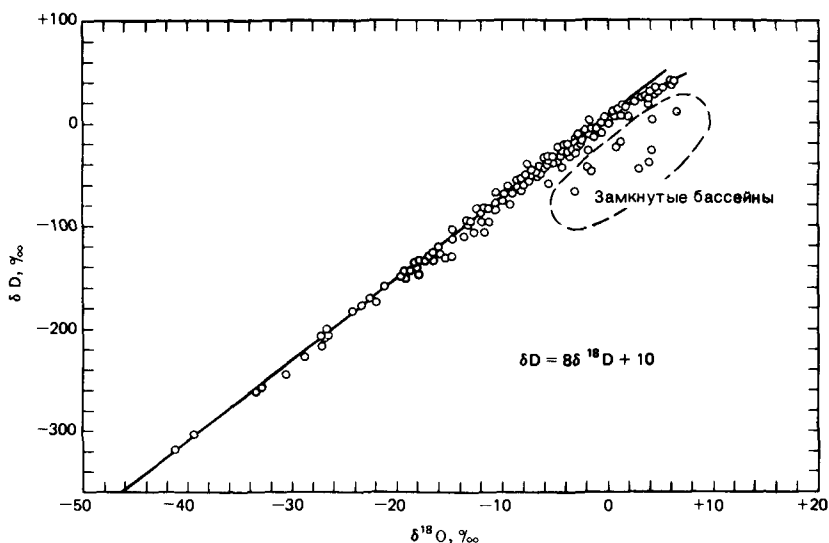
Р и с. 15.1. Изменения концентраций дейтерия и ^{18}O в реках, озерах, дождевых водах и в снегу (по Крейгу [74]).
