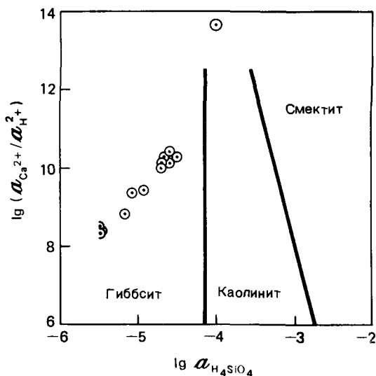
Р и в. 8.4. Пробы вод из ледникового района Южных Каскадных гор (по Рейнольдсу и Джонсону [286]), нанесенные на диаграмму устойчивости \lg(a_{Ca^{2+}}/a_{H^+}^2) - \lg a_{H_4SiO_4} . Половины кружков — содержания кремнезема ниже предела чувствительности аналитического метода (0,2 мг/л).
