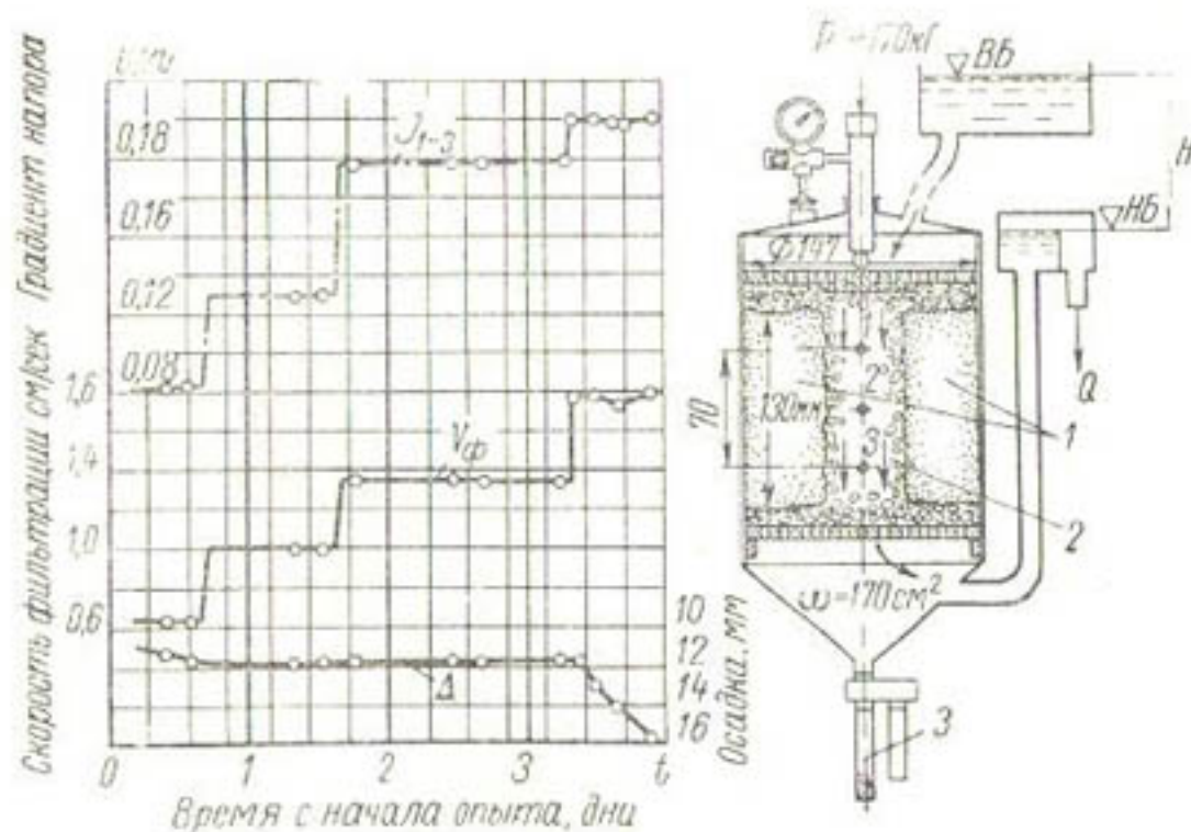
Рис. 22. Схема и результаты опыта по определению сопротивляемости суглинка размыву продольным вертикальным фильтрационным потоком в слое гравия 1—суглинок \gamma_{c,n} = 1,31 \text{ г/см}^3 ; W_n = 18,7\% ; 2—гравий; 3—песколовка.
