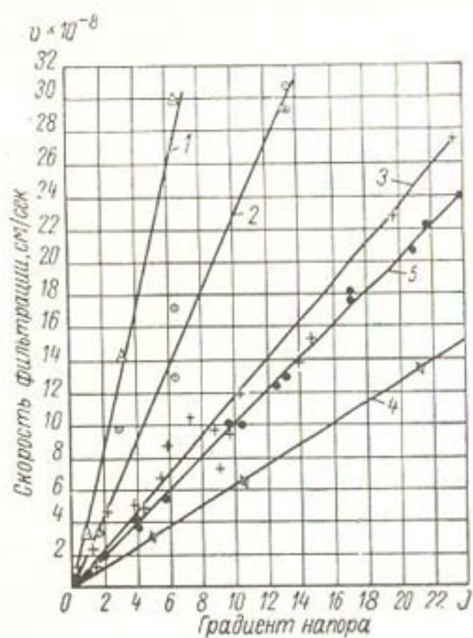
Рис. 13. Графики зависимостей между градиентом напора и скоростью фильтрации для различных связных грунтов: 1—лессовый суглинок, k=4,23 \cdot 10^{-8} см/сек (опыт № 13, продолжительностью 76 суток); 2—лессовый суглинок, k=2,25 \cdot 10^{-8} см/сек (опыт № 12, продолжительностью 84 суток); 3—кембрийская глина, k=1,16 \cdot 10^{-8} см/сек (опыт № 16, продолжительностью 132 суток); 4—ил Азовского моря, k=6,29 \cdot 10^{-9} см/сек (опыт № 15, продолжительностью 39 суток); 5—тектоническая «глина трения», заполняющая отдельные трещины в скальном массиве основания Нурекской плотины, k=1,0 \cdot 10^{-8} см/сек (опыт № 17, продолжительностью 270 суток).
