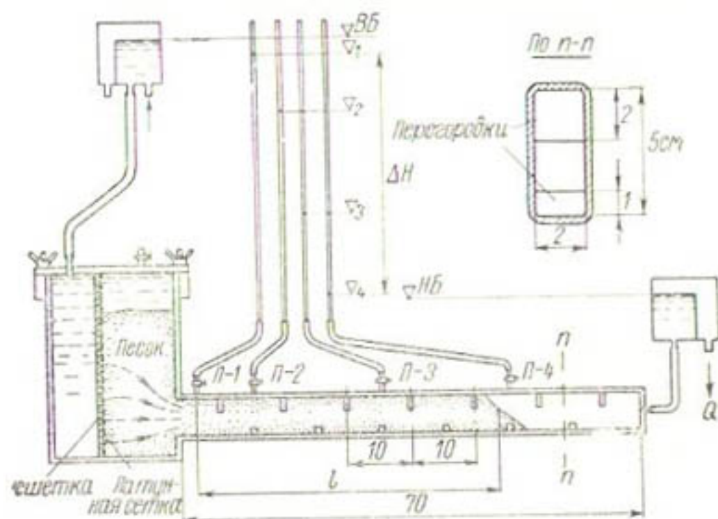
Рис. 28. Схема установки для экспериментального изучения кольматажа сквозных трещин песком.
