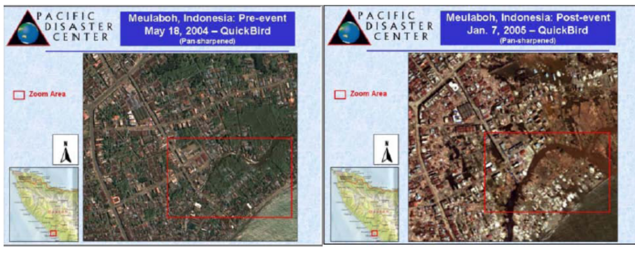
Рис. 5.9.3 Пример полученного со спутника изображения, показывающего ущерб, нанесенный цунами (фотография предоставлена Тихоокеанским центром катастроф)
