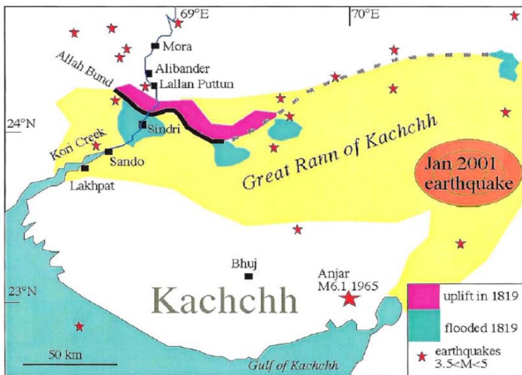
Рисунок 10.4.2 Измененная геоморфология области Кutch после землетрясения 1819 года
