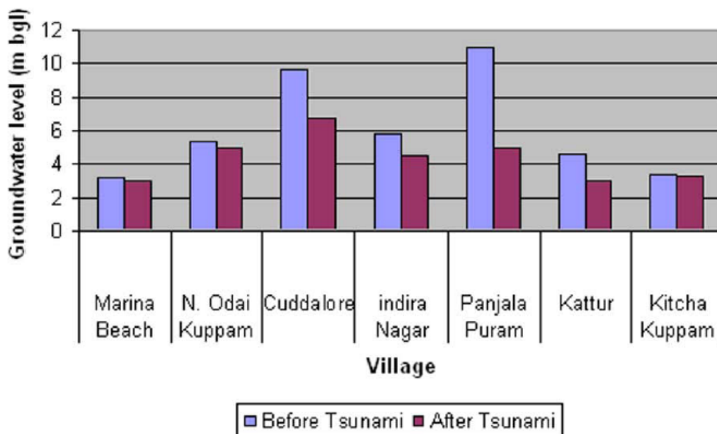
Рисунок 10.5.3 Уровни подземных вод до и после цунами
