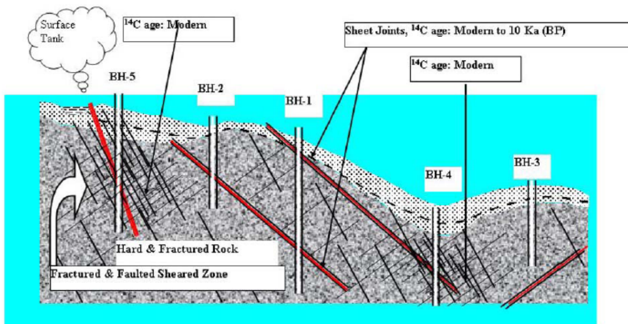
Рис. 4.2.3 Концептуальная гидрогеологическая модель, основанная на данных радиоуглеродного анализа. Модель предназначена для обнаружения глубоких водоносных пластов с большим временем удержания воды, пригодных для использования в чрезвычайных ситуациях, например, в случае засухи (Сикхия и др., 2005)
