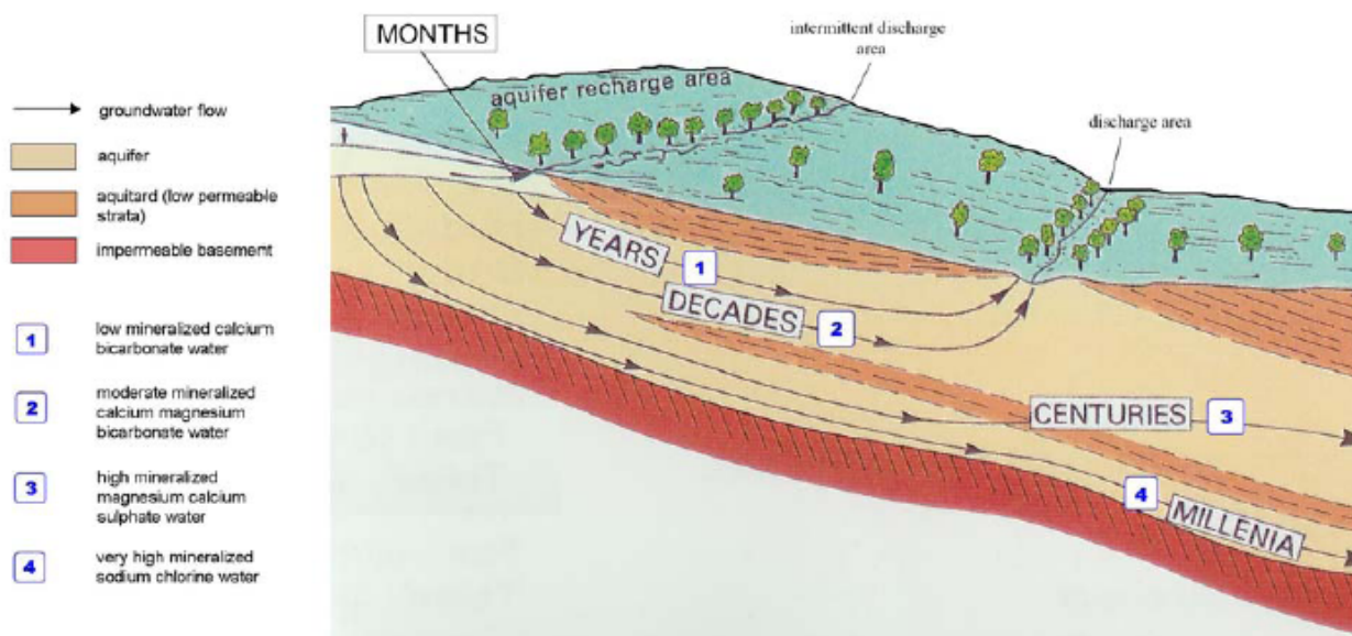
Рисунок 5.3.1 Пример структуры движения, возраста и гидрохимического состава подземных вод (не изменять масштаб, адаптировано из материалов геологических исследований Британии)
