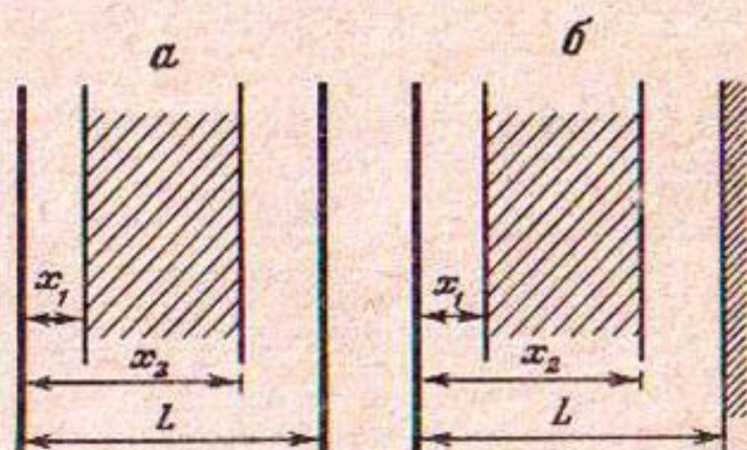
Р и с. 3.5. Схемы площадного водоотбора в условиях пластов-полос с двумя границами питания (а) и с разнородными границами (б)
