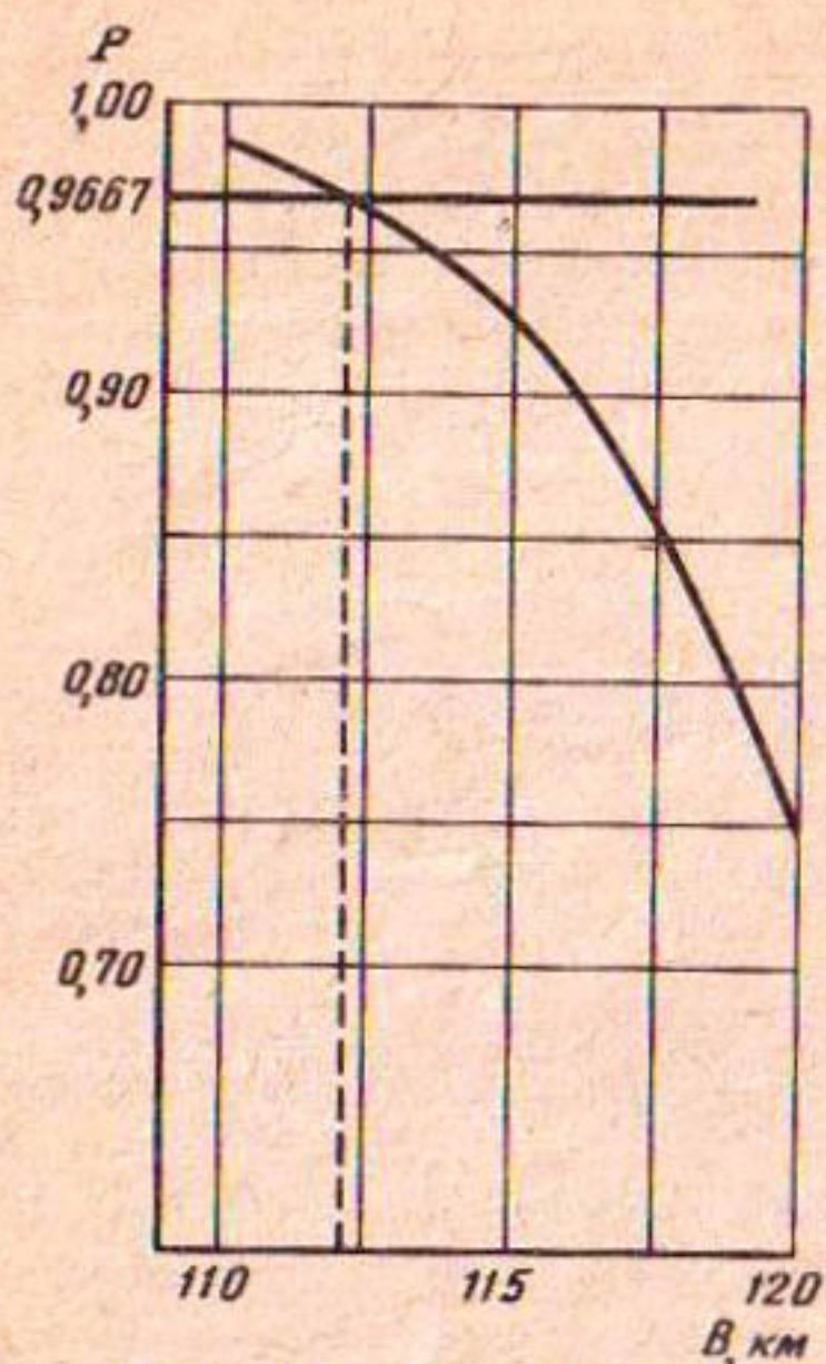
Рис. 6.7. График зависимости надежности от протяженности линейного водозабора в условиях примера
