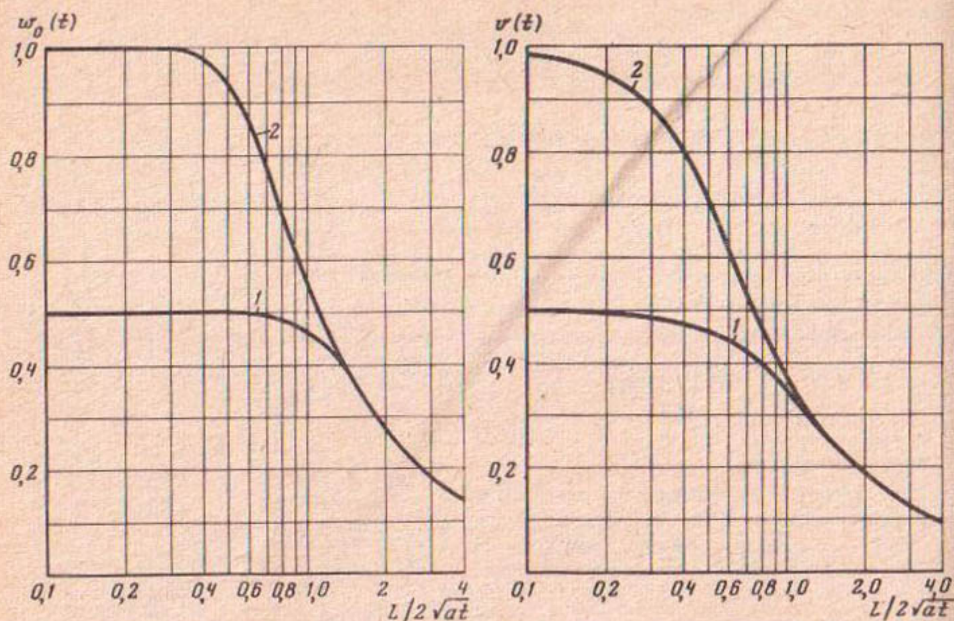
Р и с. 3.6. Графики временных зависимостей функции относительной редукции в условиях, когда площадной водозабор занимает всю полосу
