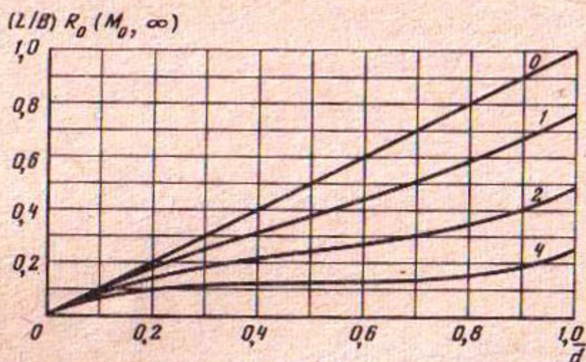
Р и с. 2.13. Зависимости предельного значения гидравлического сопротивления по линии водозабора подземных вод линейным рядом скважин в пласте-полосе с разнородными границами от относительного расстояния водозабора до границы питания Цифры у кривых — значения \chi = gL
