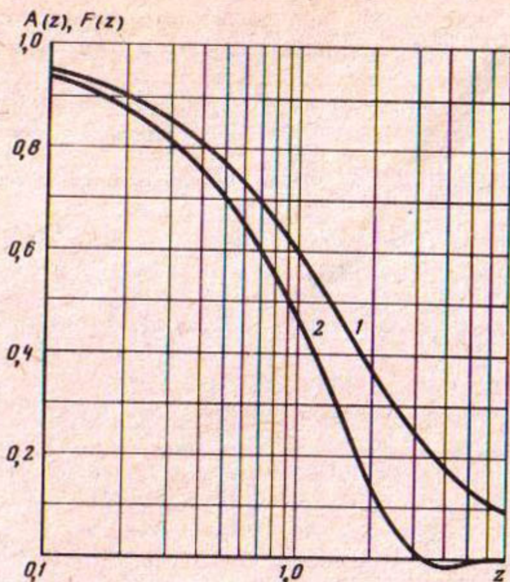
Р и с. 4.4. Графики функций A(z) (кривая 1), F(z) (кривая 2)
