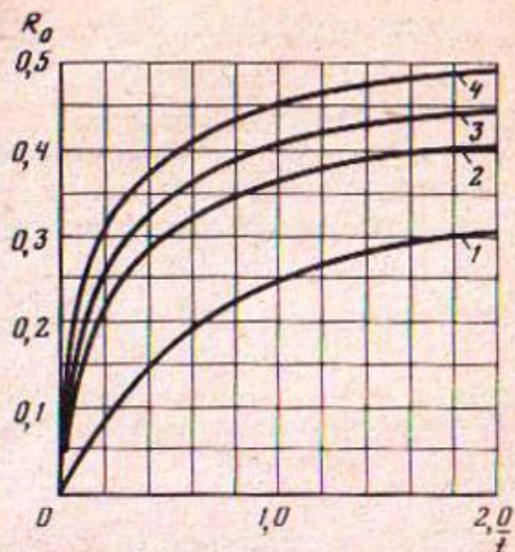
Р и с. 1.2. Графики первых трех собственных функций в условиях примера 1 и их приближений по методу Рунца
