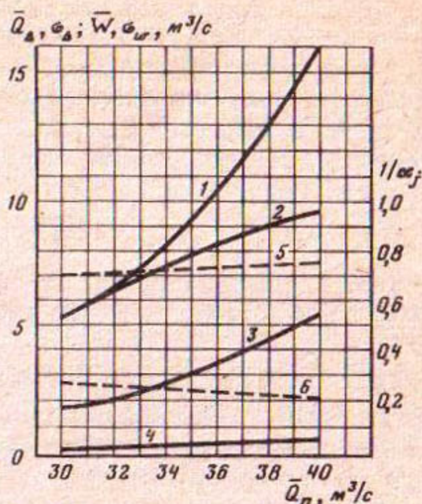
Р и с. 6.9. График надежности функционирования системы в условиях примера в зависимости от величины \bar{Q}_П
