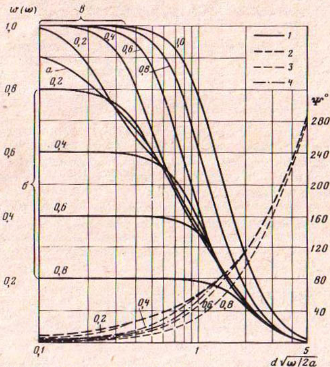
Р и с. 5.6. Частотные характеристики редукции в условиях пласта-полуполосы (а) и пластов-полос с двумя границами питания (б) и с разнородными границами (в)
