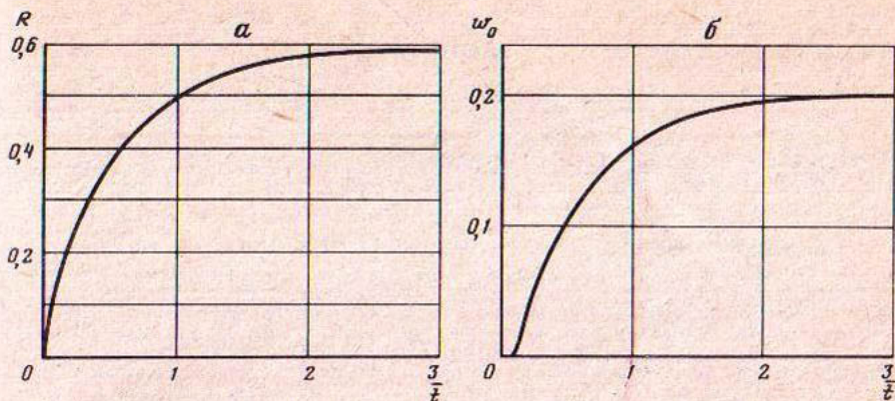
Р и с. 1.8. Графики временных зависимостей к примеру 2 а – гидравлического сопротивления; б – функции редукции
