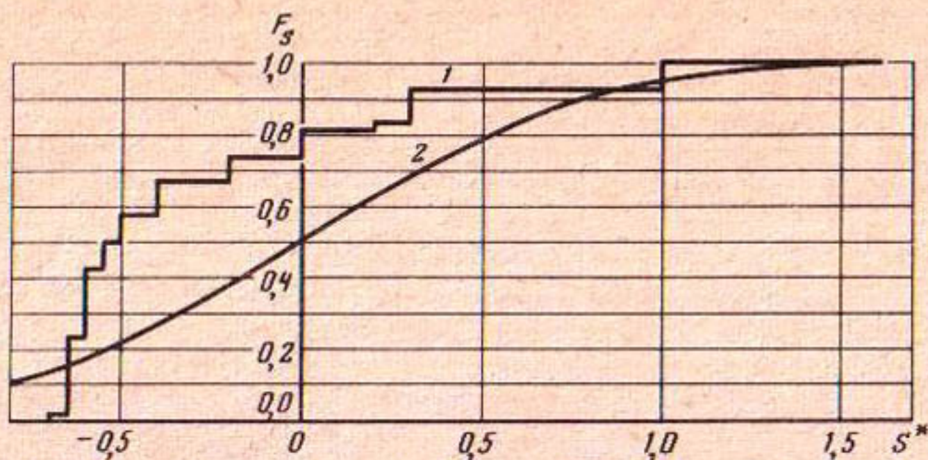
Р и с. 6.5. График эмпирического распределения величины относительного понижения S^* (кривая 1) и график функции нормального распределения с параметрами (0, \sigma_S) (кривая 2)
