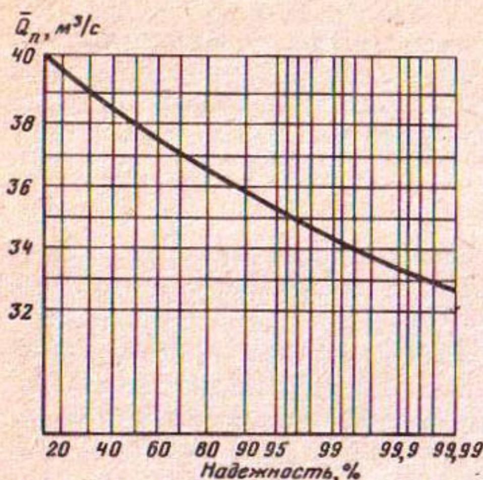
Р и с. 6.9. График надежности функционирования системы в условиях примера в зависимости от величины \bar{Q}_П
