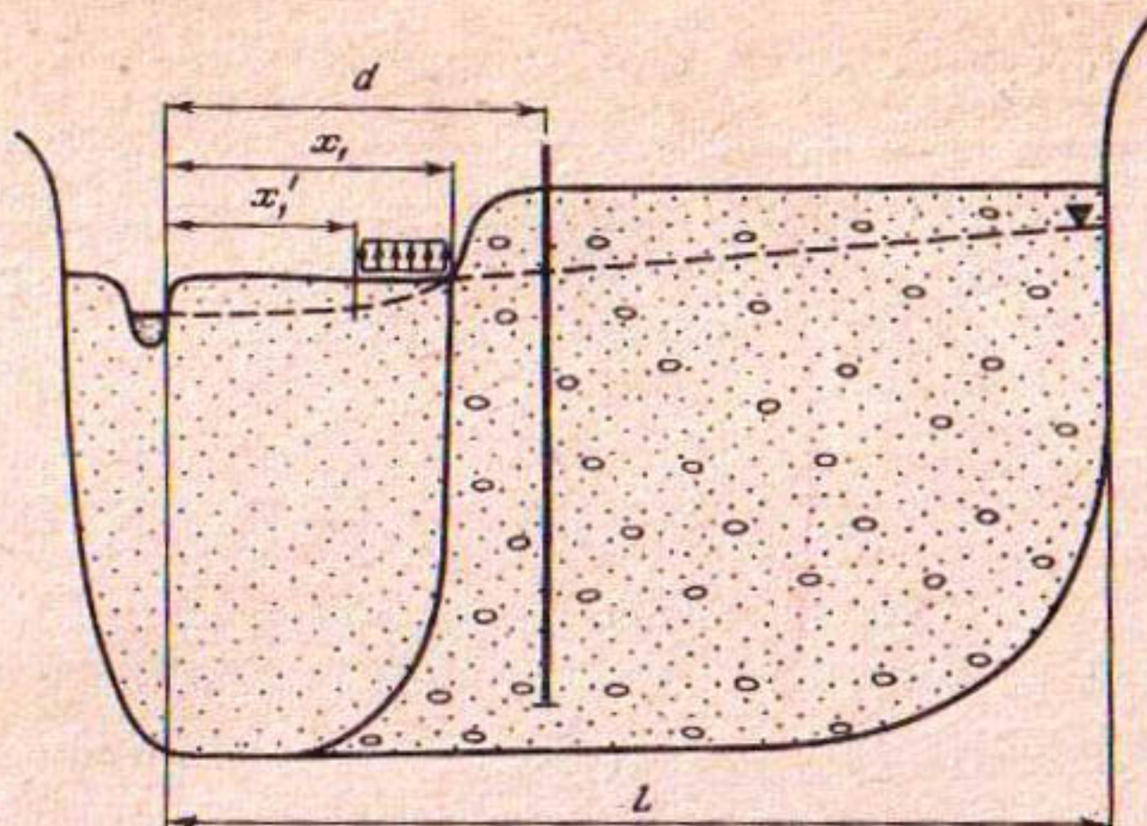
Р и с. 1.7. Схематизированный гидрогеологический разрез к примеру 2
