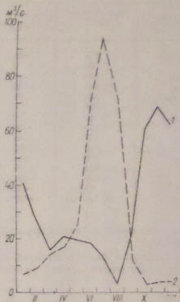
Рис. 11.4. Внутригодичное перераспределение стока. Каттакурганское водохранилище.
