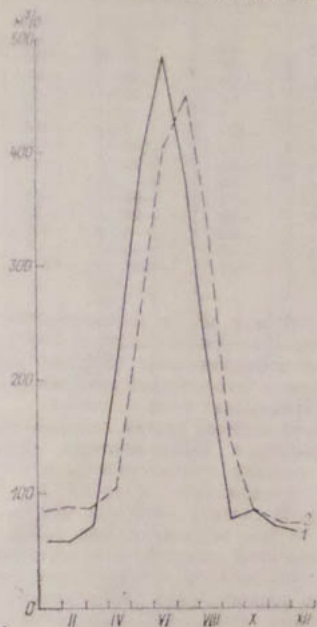
Рис. 11.3. Внутригодичное перераспределение стока. Чарвакское водохранилище.
