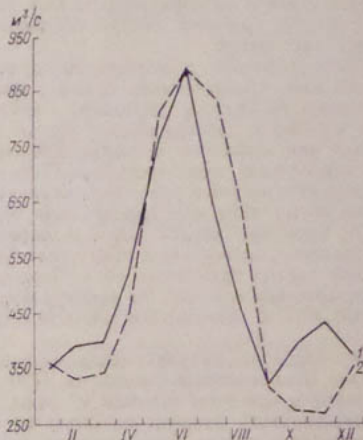
Рис. 11.1. Внутригодовое перераспределение стока Кайраккумского водохранилища. 1 — приток, 2 — отток.
