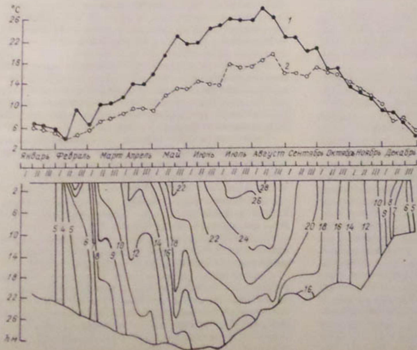
Рис. 5.12. Термоизоплеты на рейдовой вертикали Туябугузского водохранилища. 1 — поверхность, 2 — дно.
