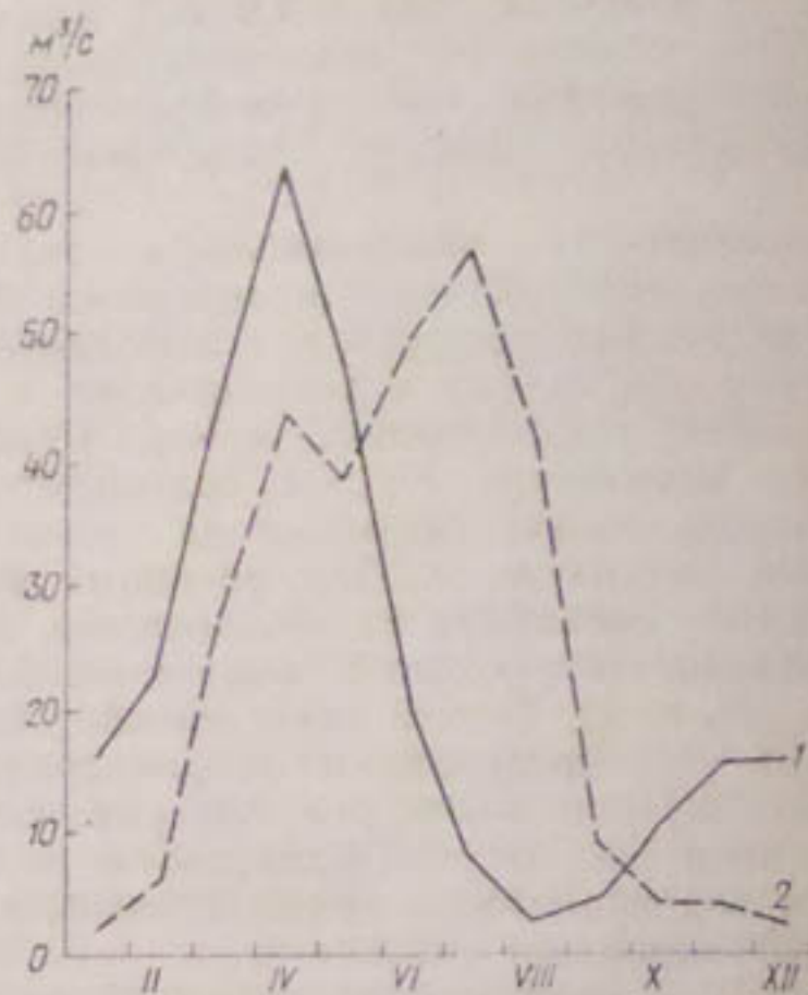
Рис. 11.2. Внутригодовое перераспределение стока. Чимкуртанское водохранилище. 1 — приток, 2 — отток.
