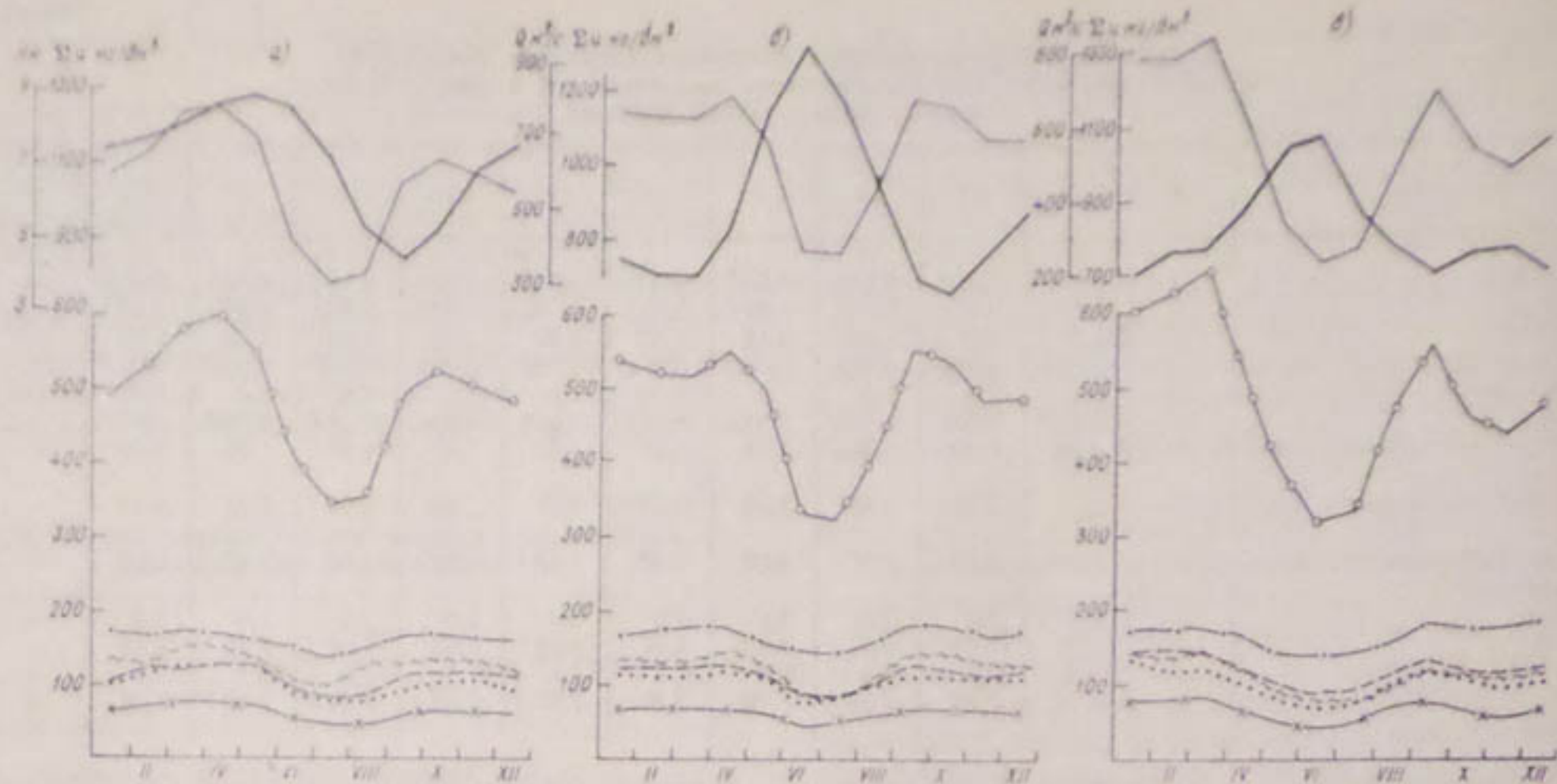
Рис. 10.8. Средневзвешенное содержание ионов и минерализация воды Кайраккумского водохранилища (а), р. Сырдарьи у поста Кызылжар (б), р. Сырдарьи у поста Чильмахрам (в). Усл. обозначения см. на рис. 10.3.
