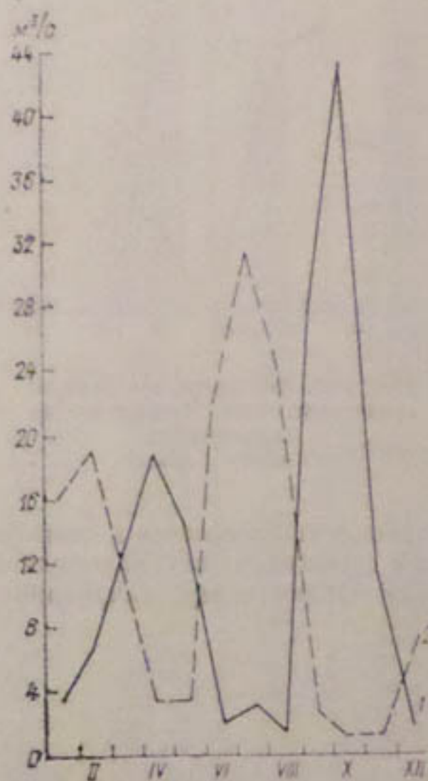
Рис. 11.5. Внутригодичное перераспределение стока. Куюмазарское водохранилище.
