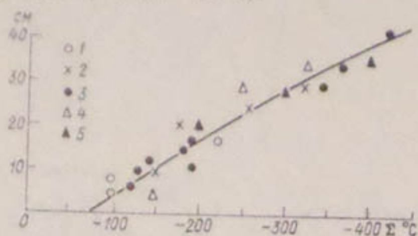
Рис. 6.7. Зависимости толщины льда (см) от сумм отрицательных температур воздуха для водохранилищ Средней Азии. Водохранилища: 1—Каттакурганское, 2—Чардаринское, 3—Тугумукское, 4—Бугуньское, 5—оз. Бийлюколь.
