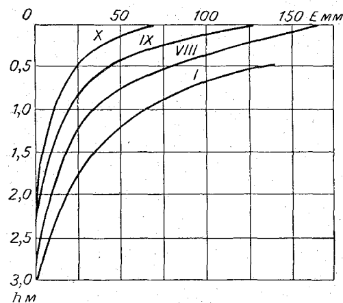
Рис. 3. Расход грунтовых вод на суммарное испарение E и влагонасыщение в зоне аэрации в зависимости от глубины грунтовых вод h (Армения, Араздайнская степь, по А. С. Акопяну).
