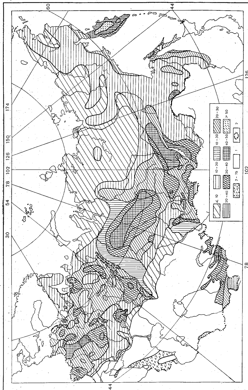
Рис. 57. Распределение величин подземного стока в реки в процентах от общего речного стока. 1 — нерассчитанная величина подземного стока, 2 — участок сложной условий формирования подземного стока.
