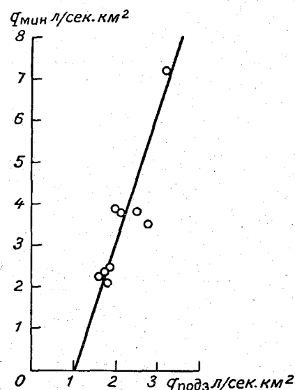
Рис. 33. График связи минимальных месячных модулей q_{мин} речного стока и среднегодовых модулей подземного питания рек q_{подз} в условиях многолетнего озерного регулирования.
