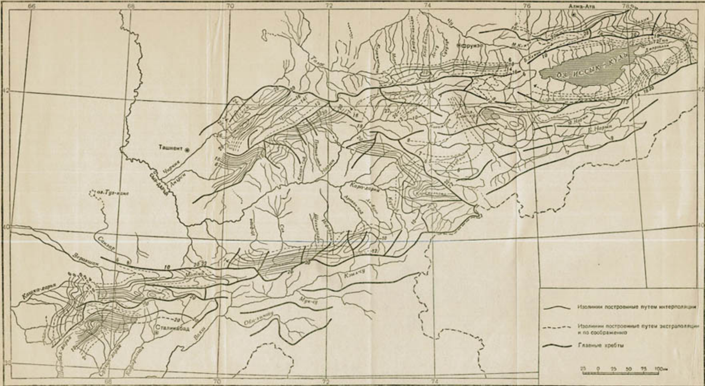
Рис. 62. Схема изолиний коэффициента A_{1\%} в формуле M_{max} = \frac{A_{1\%}}{r_{0,20}} для горной области Средней Азии.
