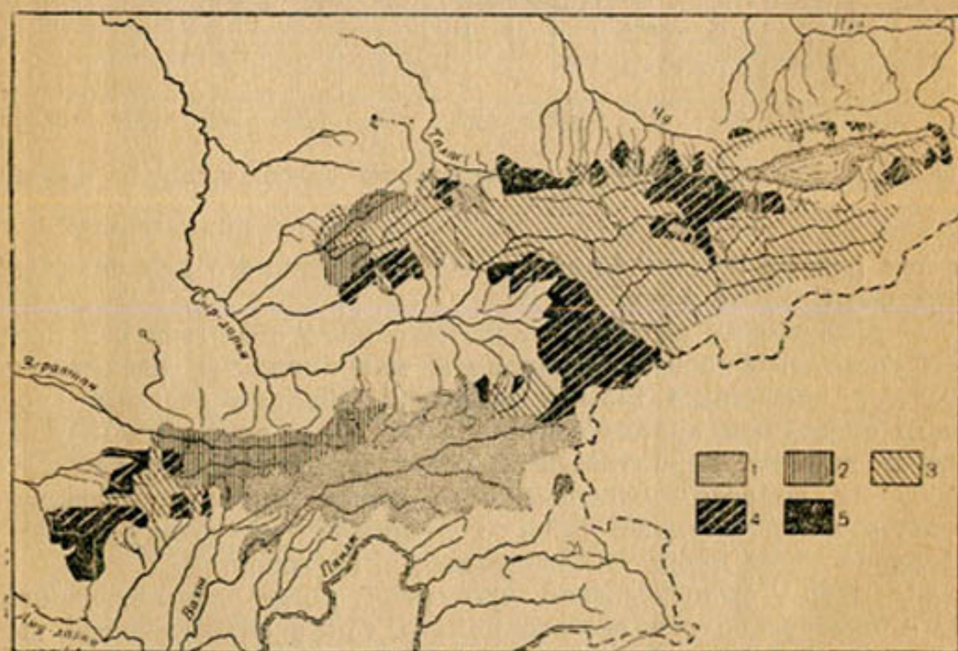
Рис. 61. Распределение коэффициентов вариации максимальных расходов воды по территории Средней Азии.
