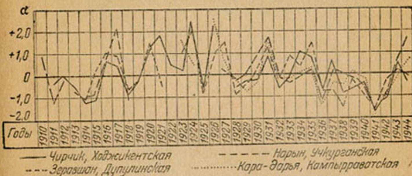
Рис. 56. Хронологическая последовательность лет с различной концентрацией стока на протяжении паводочного периода.
