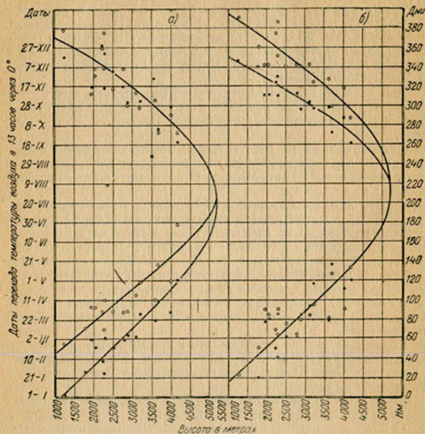
Рис. 46. Зависимость времени перехода температур воздуха в 13 часов через 0° (положение фронта снеготаяния) от высоты местности для крайних лет.
