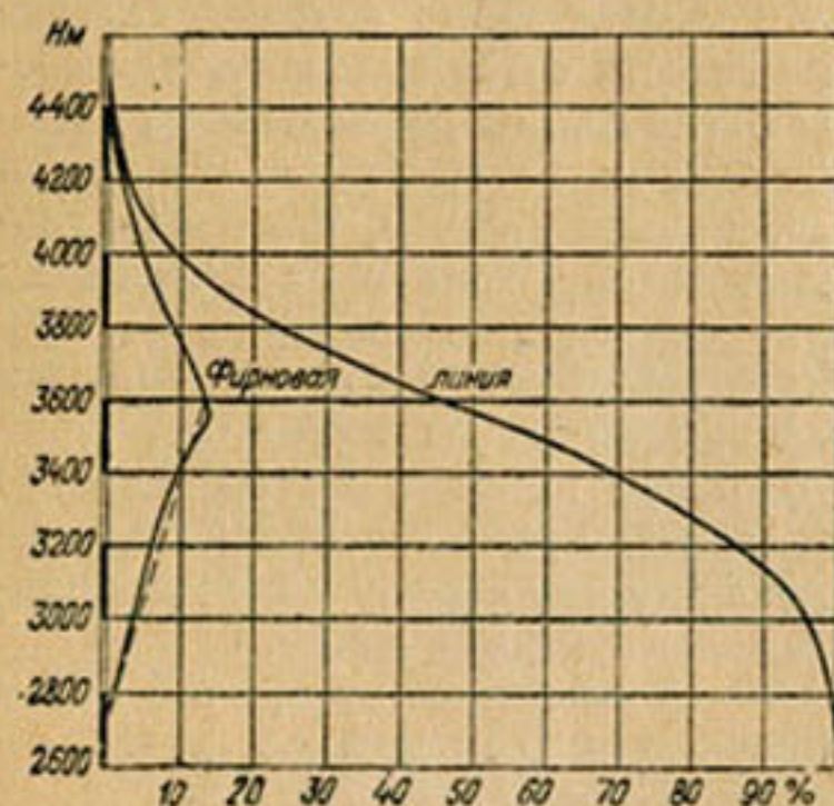
Рис. 6. Кривая распределения и гипсометрическая кривая площади оледенения в водосборе р. Сох.
