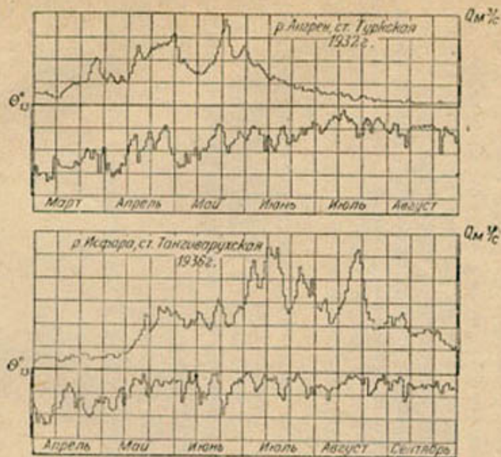
Рис. 21. Ход расходов воды и температур воздуха за период интенсивного снеготаяния в водосборах р. Ангрен (ст. Туркская) за 1932 г. и р. Исфара (ст. Тангварухская) за 1936 г.
