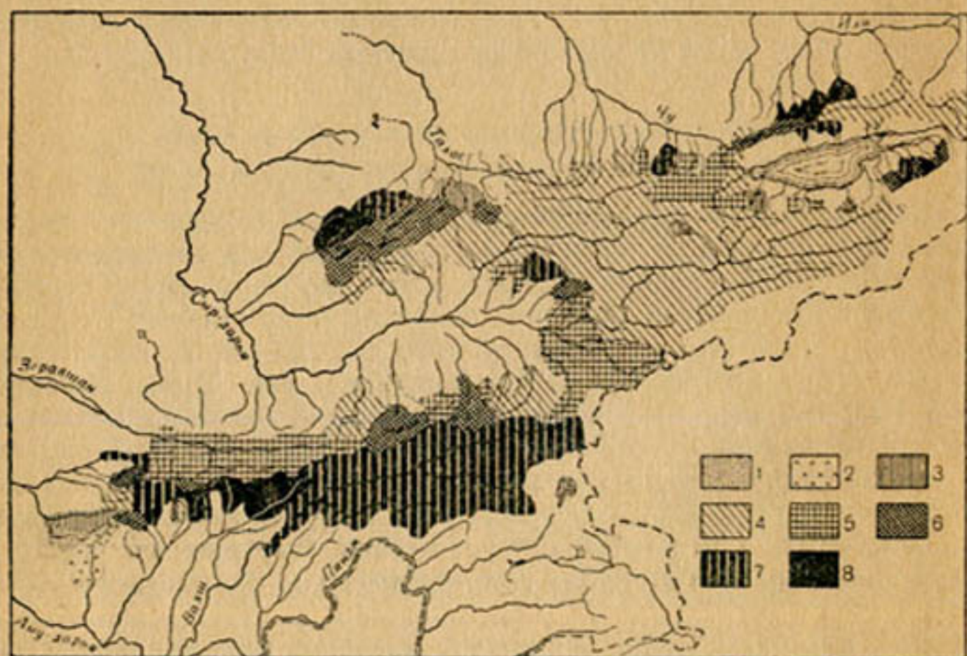
Рис. 64. Распределение средних месячных минимальных модулей стока по территории Средней Азии.
