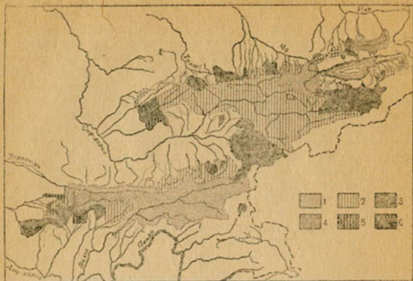
Рис. 55. Коэффициенты вариации за период октябрь–февраль: 1 — 0,00–0,10; 2 — 0,10–0,15; 3 — 0,15–0,20; 4 — 0,20–0,25; 5 — 0,25–0,30; 6 — свыше 0,30.
