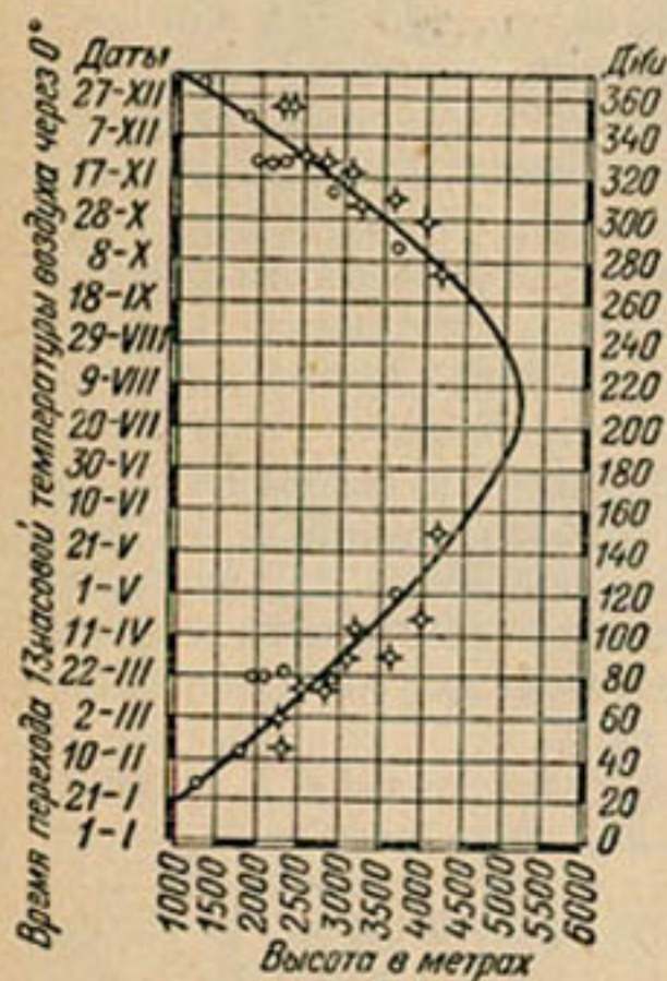
Рис. 27. Зависимость среднего времени перехода температур воздуха в 13 часов через 0^{\circ} (положения фронта снеготаяния) от высоты местности.
