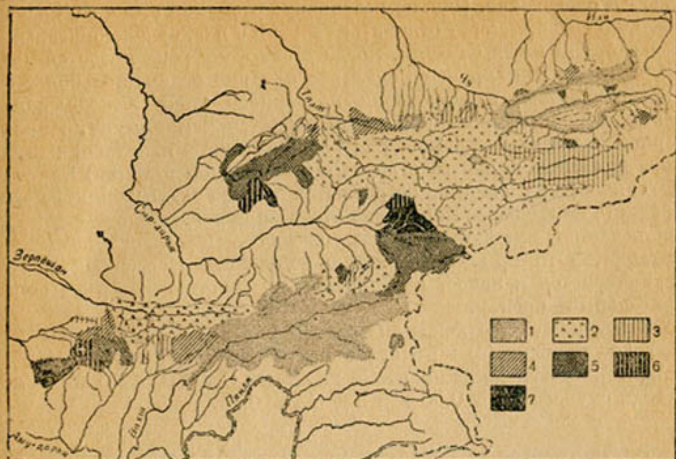
Рис. 55 2 . Коэффициенты вариации за период июль—сентябрь: 1 — 0,10—0,15; 2 — 0,15—0,20; 3 — 0,20—0,25; 4 — 0,25—0,30; 5 — 0,30—0,40; 6 — 0,40—0,50; 7 — свыше 0,50.
