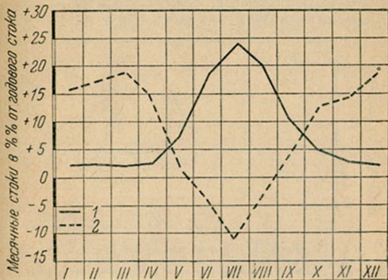
Рис. 25. Ход величин месячного стока р. Зеравшан (при выходе из гор) и возвратных вод.
