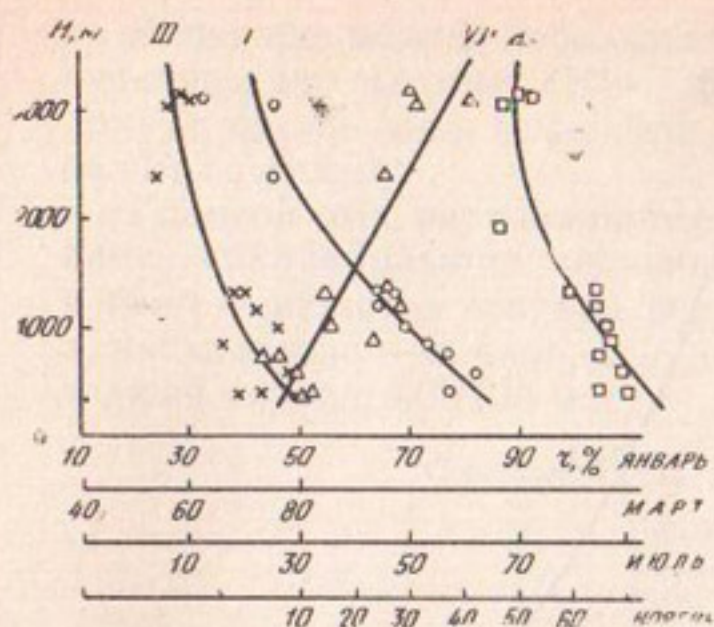
Рис. 5. Зависимость среднемесячной относительной влажности воздуха от высоты для северного склона Туркестанского хребта: I — январь, III — март, VII — июль, XI — ноябрь.
