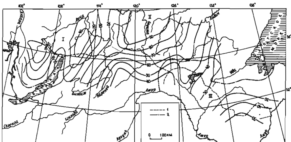
Рис.8.6. Средняя многолетняя толщина речных наледей, приведенная к площади водосбора 5000 км 2 и высоте местности 500 м абс., в зоне БАМ, см. 1 - трасса БАМ, 2 - граница и номера районов по характеру связи на рис.8.5
