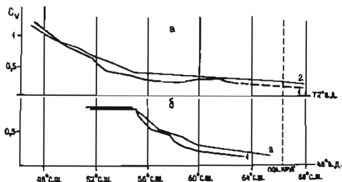
Рис. 9.5. Меридиональные профили изменений коэффициентов вариации C_v полного речного стока (1) и стока половодья (2); а - Европейская территория бывшего СССР, б - Западно-Сибирская низменность
