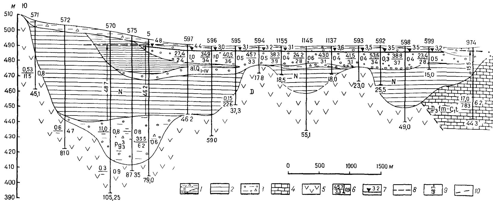
Рис 27 Гидрогеологический разрез Жартас Котурского участка долины р Джон по линии А—Б (составила Э Д Кузьмина по материалам В А Курдюкова)
