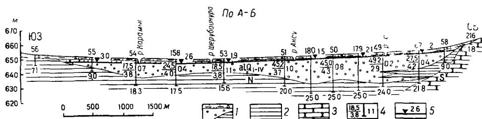
Рис 36 Гидрогеологический разрез долины р Шерубайнуры (см рис. 35) по линии А—Б (составил И. И. Ротарь)
