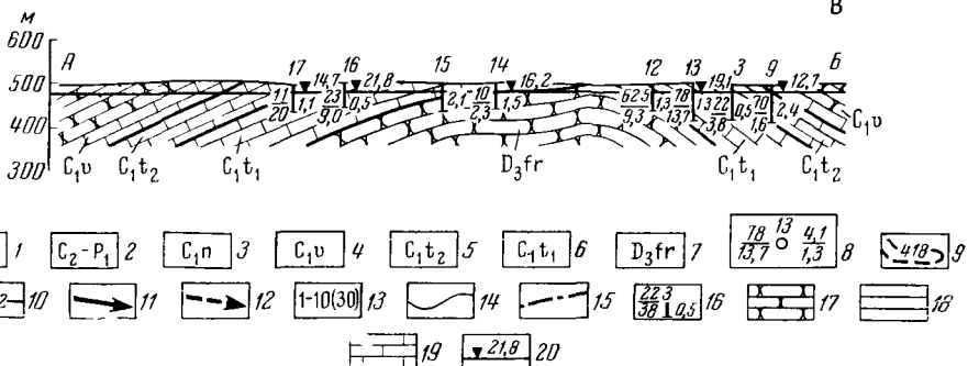
Рис 22 Гидрогеологическая карта Жанайской антиклинали (составил М. А Хорди-кайнен по материалам С К Калугнна)
