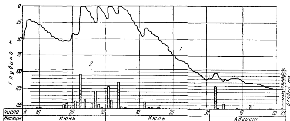
Рис. 57. График режима уровня подземных вод гранитоидов в районе Балхаш-Нуринского водораздела 1 — уровень воды в скважине, 2 — внутригодичное распределение атмосферных осадков
