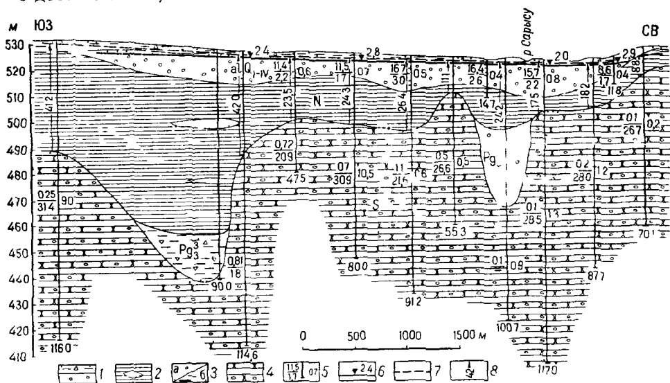
Рис 44 Гидрогеологический разрез верховья долины р. Сарысу (составил А. Насырханов)
