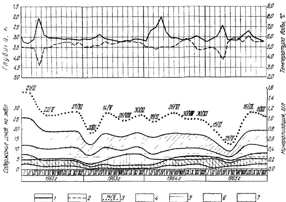
Рис. 61. Графики режима уровня и химического состава грунтовых вод аллювиальных четвертичных отложений Сергиопольского участка долины р. Нуры (составил К. И. Сычев) 1 — уровень воды в скважине; 2 — температура воды на гидрохимическом графике; 3 — линия общей минерализации воды (г/л); содержание ионов (мг. экв/л): 4 — \text{HCO}_3^- ; 5 — \text{SO}_4^{2-} ; 6 — \text{Cl}^- ; 7 — \text{Mg}^{2+} . Содержание \text{Ca}^{2+} откладывается от нуля графика
