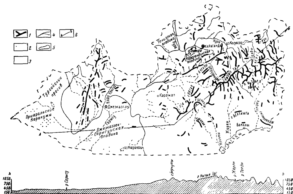
Рис. 9. Орографическая схема территории Карагандинской области (составил М. А. Авербух)
