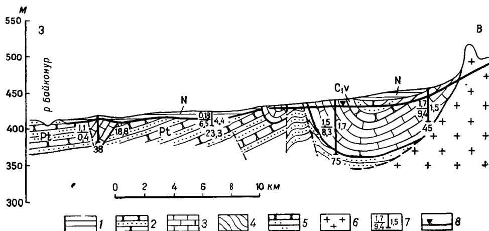
Рис. 20. Гидрогеологический разрез по приразломной Сарысайской мульде (составил М. А. Хордикийен по материалам В. Н. Островского)
