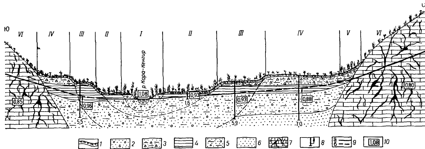
Рис. 21. Характер распределения растительности в поперечном сечении долины р. Кара-Кенгир на участке Кожамсит (составил В. Н. Островский)
