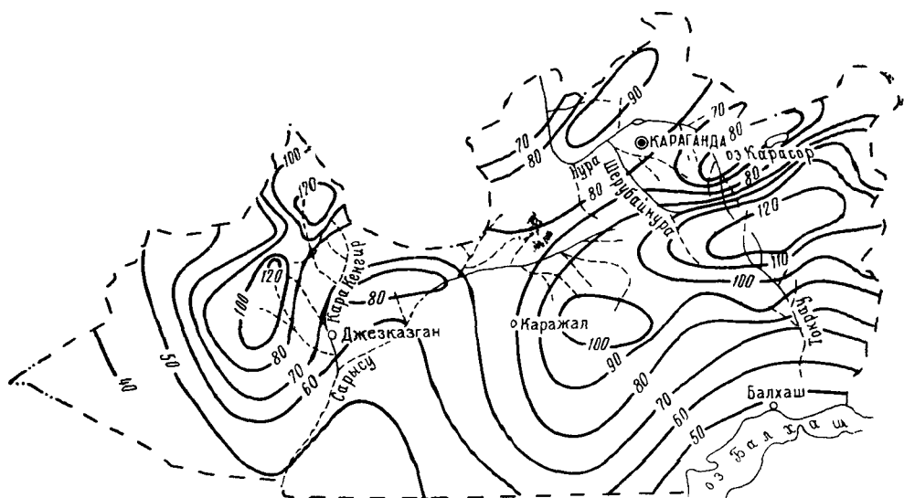
Рис 5 Карта запасов воды в снежном покрове (в мм) по Карагандинской области
