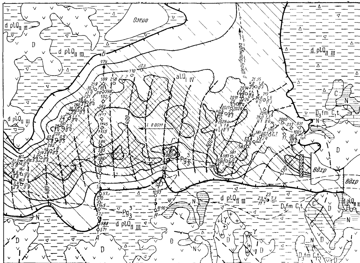
Рис 26 Гидрогеологическая карта Жар- тас Котурского участка долин рек Ше- рубайнуры и Джон (составил Л А Де- нисова по материалам С Мырзахано- ва, Т В Зыковой)
