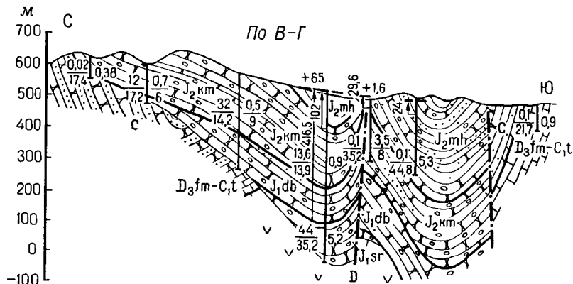
Рис. 33. Гидрогеологические разрезы Карагандинского артезианского бассейна по линиям А—Б и В—Г (составили И. М. Детцель, Н. С. Евтюхина)
