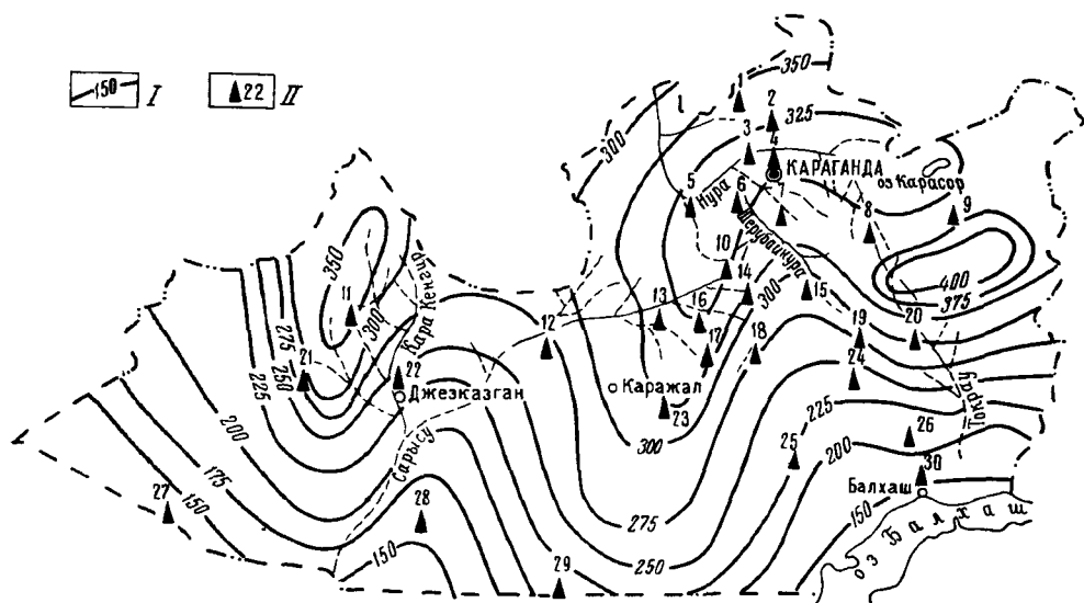
Рис 3 Карта годовых осадков по Карагандинской области
