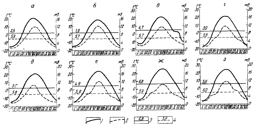
Рис. 2. Графики колебаний температуры и абсолютной влажности воздуха за многолетний период по метеорологическим станциям Карагандинской области а — Караганда; б — Каркаралинск; в — Улутау; г — Жанаарка; д — Жарык; е — Джезказган, ж — Бетпакдала; з — Балхаш 1 — кривая колебаний средней годовой температуры; 2 — кривая колебаний средней годовой абсолютной влажности; 3 — средняя годовая температура; 4 — средняя годовая абсолютная влажность
