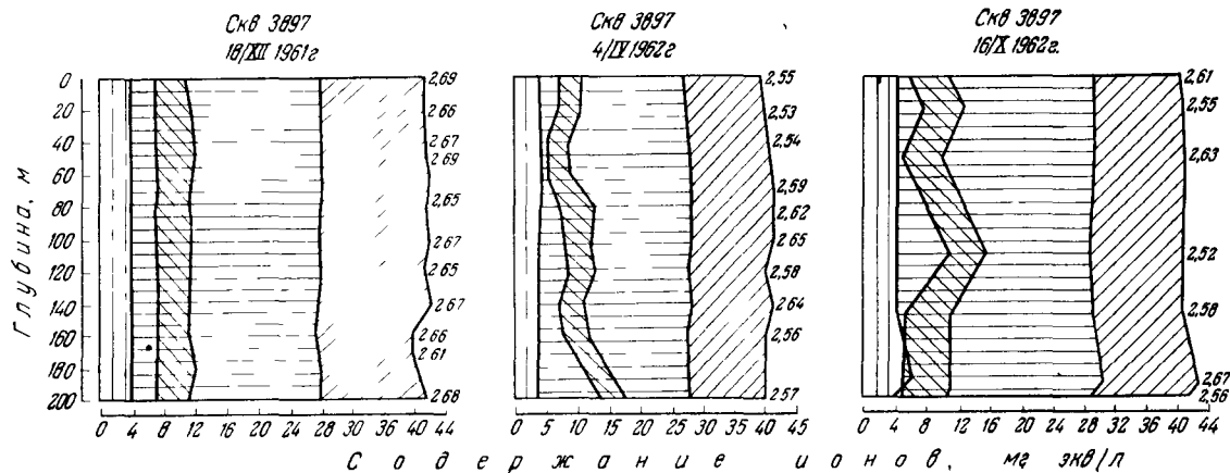
Рис. 39. Графики вертикальной гидрохимической зональности подземных вод Джезказганского месторождения
