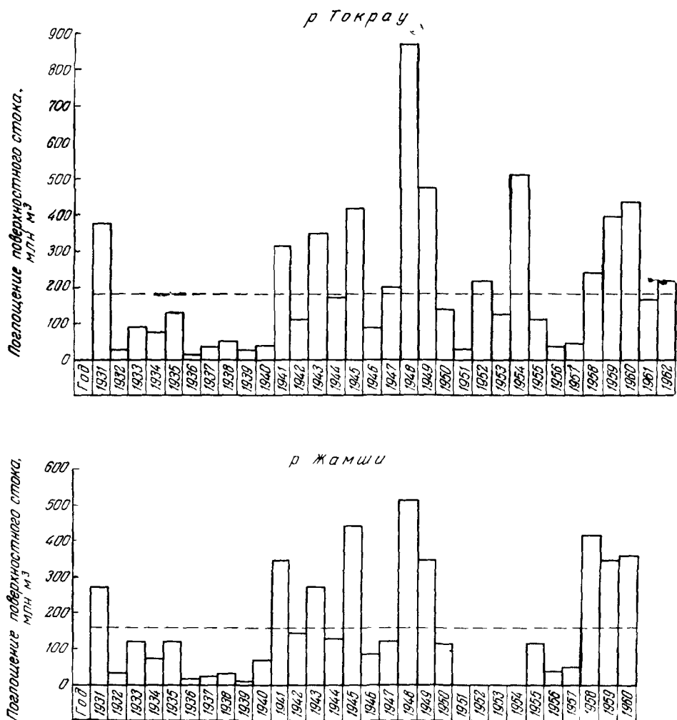
Рис. 58. Диаграмма поглощения поверхностного стока за многолетний период водоносным горизонтом аллювиальных четвертичных отложений (составил К. И. Сычев). Пунктир — норма поглощения поверхностного стока (млн. м³)
