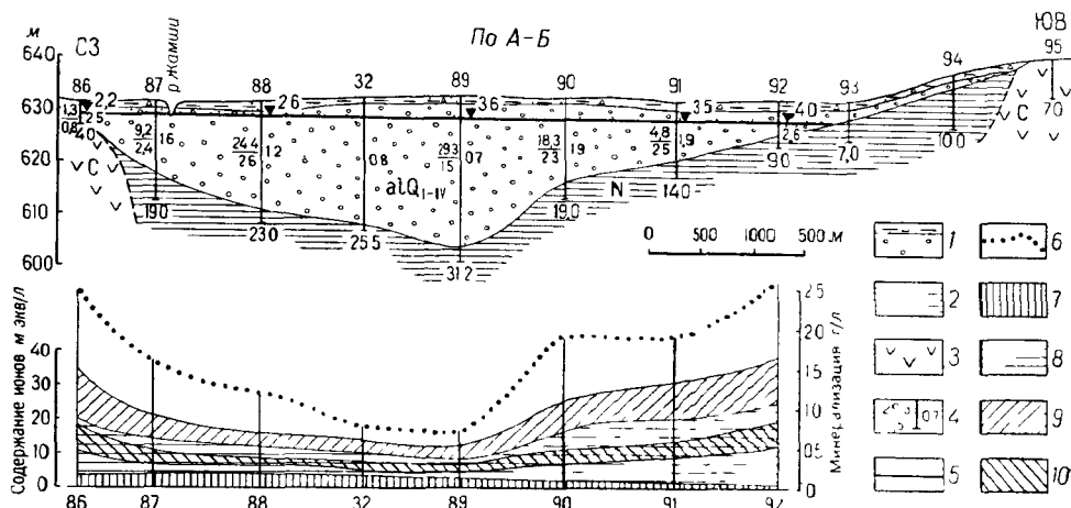
Рис. 46. Гидрогеологический разрез (см. рис. 45) и гидрохимический профиль долины р. Жамши по линии А—В (составила Л. А. Денисова по материалам Е. А. Кожевниковой)
