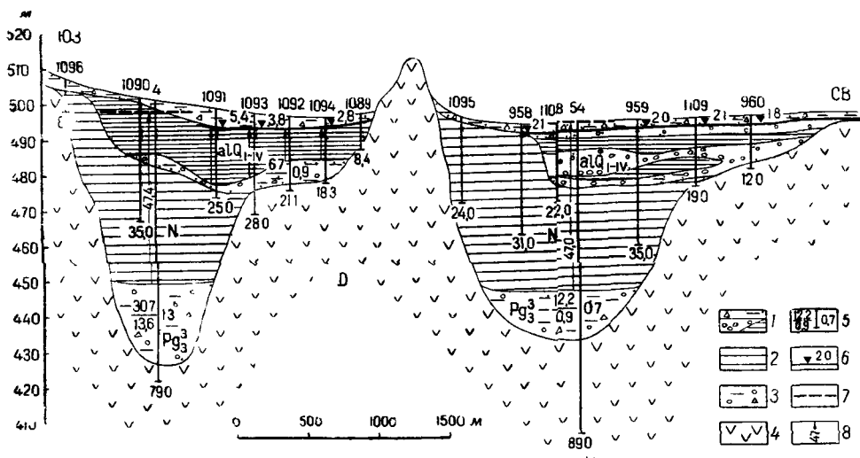
Рис 28 Гидрогеологический разрез Жартас-Котурского участка долины р. Джон по линии В—Г (составила Э. Д. Кузьмина по материалам В. А. Курдюкова)
