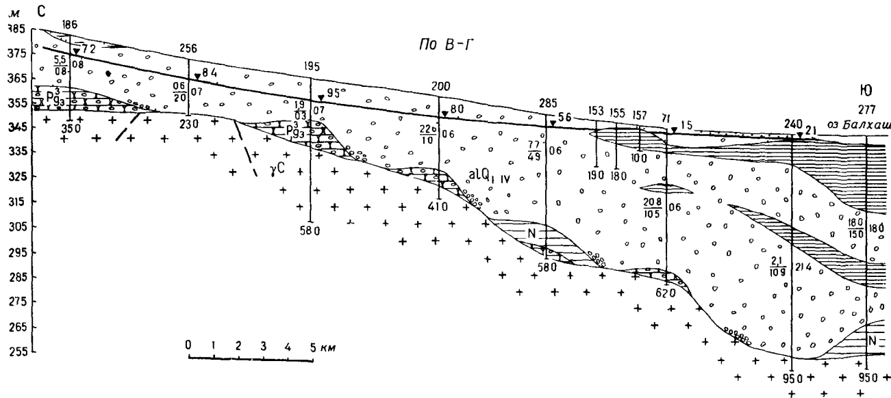
Рис 48 Гидрогеологические разрезы низовья р Токрау (составил В А Андрусевич по материалам К И Сычева, К И Ишмакова) 1 — водоносный горизонт аллювиальных нижнечетвертичных — современных отложений ( alQ_{I-IV} ) Песчано гравийно галечниковые отложения с прослоями су- глинок супесей и глин 2 — водоупорные пестроцветные глины (N) 3 — практически водонепроницаемые верхнеолигоценовые сливные конгломераты ( Pg_3^3 ) 4 — подземные воды зоны открытой трещиноватости вулканических пород (C) Порфириды и их туфы 5 — подземные воды зоны открытой трещи- новатости каменноугольных интрузивных пород ( \gamma C ) Граниты 6 — тектонические нарушения 7 — скважины слева в числителе — дебит ( л/сек ) в знаменате- ле — минерализация воды ( г/л ), 8 — уровни грунтовых вод
