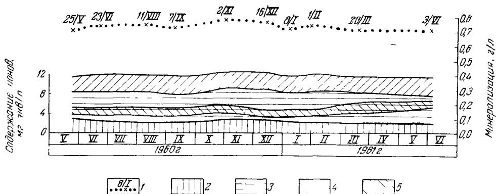
Рис. 51. График изменения минерализации и химического состава грунтовых вод аллювиальных четвертичных отложений низовья долины р. Токрау (составил К И Сычев)
