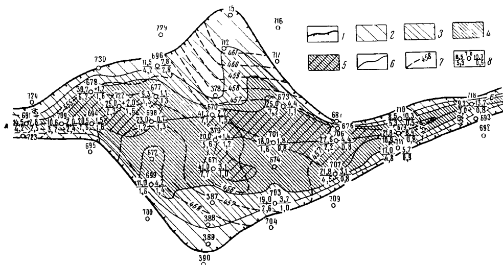
Рис. 29 Гидрогеологическая карта водоносного горизонта верхнеолигоценовых отложений Молодецкого участка долины р. Нуры (составила Э. Д. Кузьмина по материалам П. И. Савчука, Ж. Букетова)
