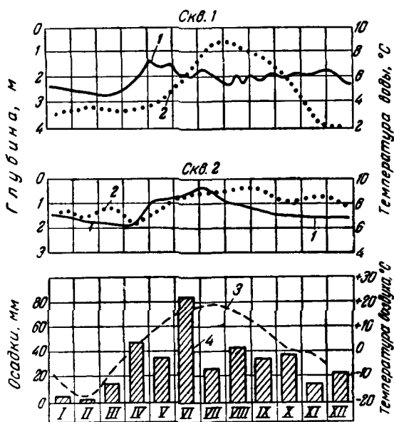
Рис. 56. График режима уровня подземных вод Каркаралинского гранитного массива 1 — уровень воды в скважинах; 2 — температура воды, 3 — температура воздуха; 4 — внутригодичное распределение атмосферных осадков
