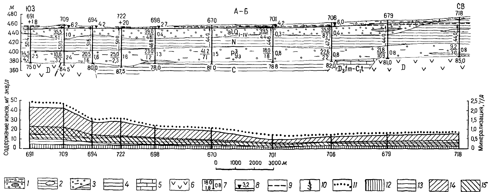
Рис 31 Продольный гидрогеологический разрез и гидрохимический профиль (см рис 30) Молодецкого участка долины р Нуры по линии А—Б (составила Л И Савицкая)
