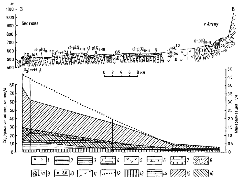
Рис 43 Гидрогеологический разрез и гидрохимический профиль восточного крыла Джайльминской синклинали по линии Бестюбе-Актау (составил Л. Я. Тененбаум). 1 — воды спорадического распространения делювиально-пролювиальных средне-верхнечетвертичных отложений ( dplQ_{II-III} ). Супеси и суглинки с линзами песков; 2 — водоупорные пестроцветные неогеновые глины (N), 3 — водоносный комплекс осадочных каменноугольных отложений (C) Аргиллиты, пересланяющиеся с алевролитами и песчанками, 4 — водоносный комплекс карбонатных фаменских и турнейских отложений ( D_3fm-Ct ) Известняки, 5 — подземные воды зоны открытой трещиноватости эффузивных девонских пород (D) Порфириды, альбитофиры, туфы, 6 — водоносный комплекс осадочных силурийских отложений (S) Песчаники и алевролиты 7 — водоносный комплекс осадочных ордовикских отложений (O) Песчаники с прослоями конгломератов и алевролитов, 8 — подземные воды зоны открытой трещиноватости метаморфических протерозойских пород (Pt) Кварциты и метаморфические сланцы, 9 — скважины слева в числителе — дебит (л/сек), в знаменателе — понижение (м), справа — минерализация воды (г/л), 10 — уровень подземных вод; 11 — тектонические нарушения, на гидрохимическом профиле 12 — линия общей минерализации воды (г/л); содержание ионов (мг.экв/л) 13 — HCO_3^- , 14 — SO_4^{2-} , 15 — Cl^- , 16 — Mg^{2+} Содержание Ca^{2+} откладывается от нуля графика
