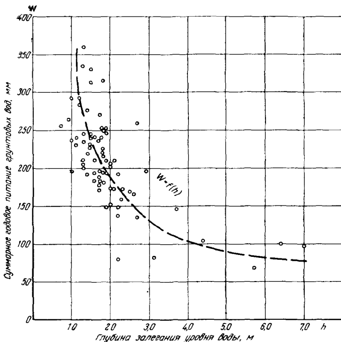
Рис. 59. График зависимости суммарного годового питания грунтовых вод от глубины залегания уровня воды (составил К. И. Сычев)
