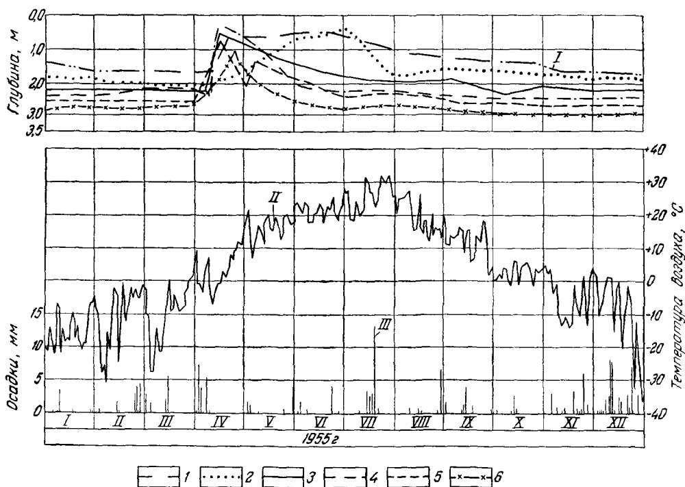
Рис. 53. График режима уровня грунтовых вод аллювиальных четвертичных отложений Жартасского участка долины р. Шерубайнуры
