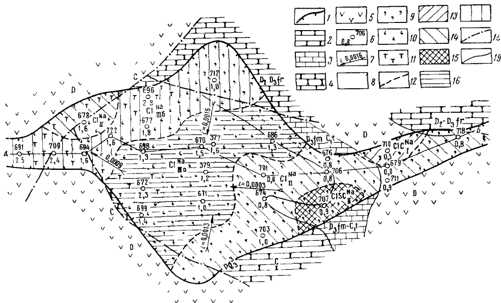
Рис. 30. Гидрохимическая карта водоносного горизонта верхнеолигоценовых отложений Молодецкого участка долины р. Нуры (составила Э. Д. Кузьмина по материалам П. И. Савчука, Ж. Букетова)
