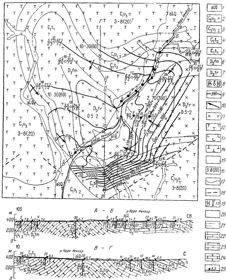
Рис 23 Гидрогеологическая карта Айдооской антиклинали (составили М. А. Хор и А. А. Емельянов)
