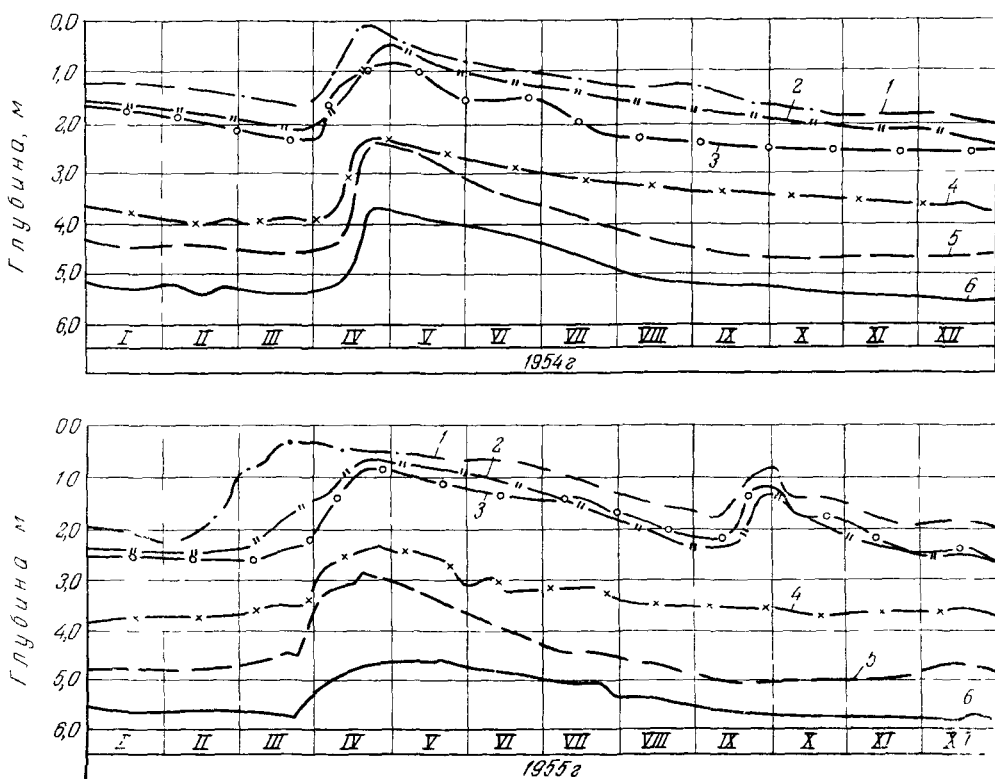
Рис. 54. График колебания уровня подземных вод Куинского гранитного массива скважины: 1 — 23; 2 — 14; 3 — 19; 4 — 39; 5 — 18; 6 — 22
