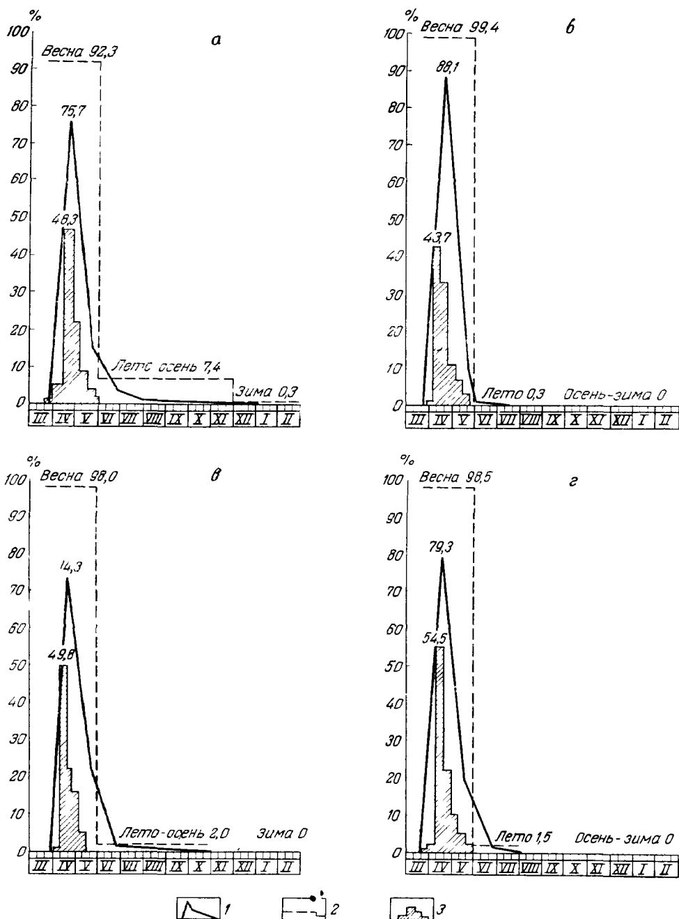
Рис. 10 Среднее распределение стока по рекам Нуре, Моинты, Сарысу и Кара-Кенгиру в характерные по водности годы (по данным Е. Г. Юриной) а — р. Нура у с. Сергиопольское; б — р. Моинты у ст. Кник; в — р. Сарысу у разъезда № 57; г — р. Кенгир в 5 км выше устья р. Жиланды 1 — средний многолетний сток по месяцам, 2 — средний многолетний сток по сезонам года, 3 — средний многолетний подекадный сток в период паводка
