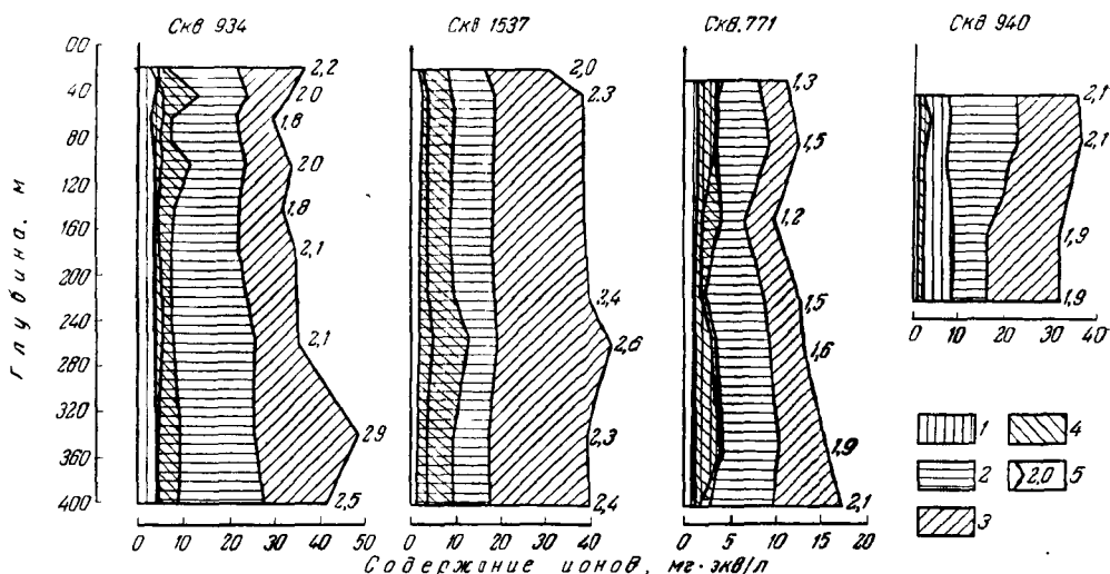
Рис. 38. Графики вертикальной гидрохимической зональности подземных вод Жиландинского месторождения
