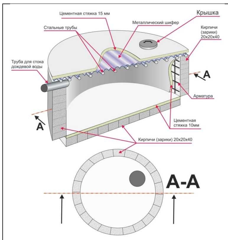
Рисунок 7 – Схема сардобы
