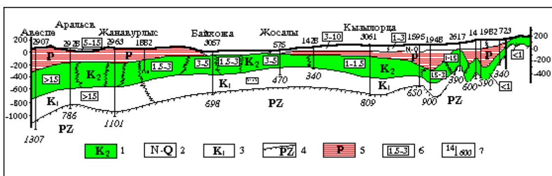
Рис. 2. Схематический гидрогеологический разрез по линии I-I
