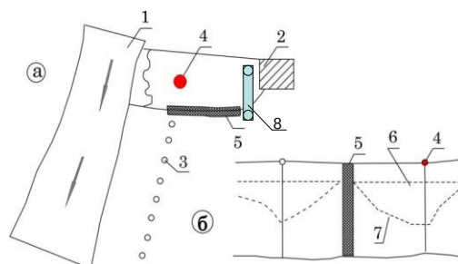
Рис. 5. Комплексный барьер в долине реки: 1 – потоки загрязненных вод, 2 – элювий, 3 – илисто-глинистые отложения, 4 – глины и суглинки, 5 – аллювиальный водоносный горизонт, 6 – УГВ, 7 – река с чистой водой, 8 – водоупор, 9 – геохимический барьер, 10 – гидродинамический барьер, 11 – водозаборные скважины, 12 – дренаж, 13 – источник загрязнения.
