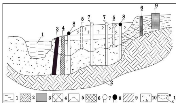
Рис. 9. Комплексный барьер с двухсторонним поступлением загрязняющих веществ к водозаборам хозяйственно-питьевых вод одновременно от реки и с водосбора. 1 – водоем с загрязненной водой, 2 – водоупорные барьеры: 3 – биохимический, 4 – природно-техногенный, 5 – гидродинамический, 6 – искусственный геохимический, 7 – водозаборные скважины, 8 – дренажные скважины, 9 – источник загрязнения, 10 – аллювиальный горизонт, 11 – УГВ (а – статический, б – динамический).
