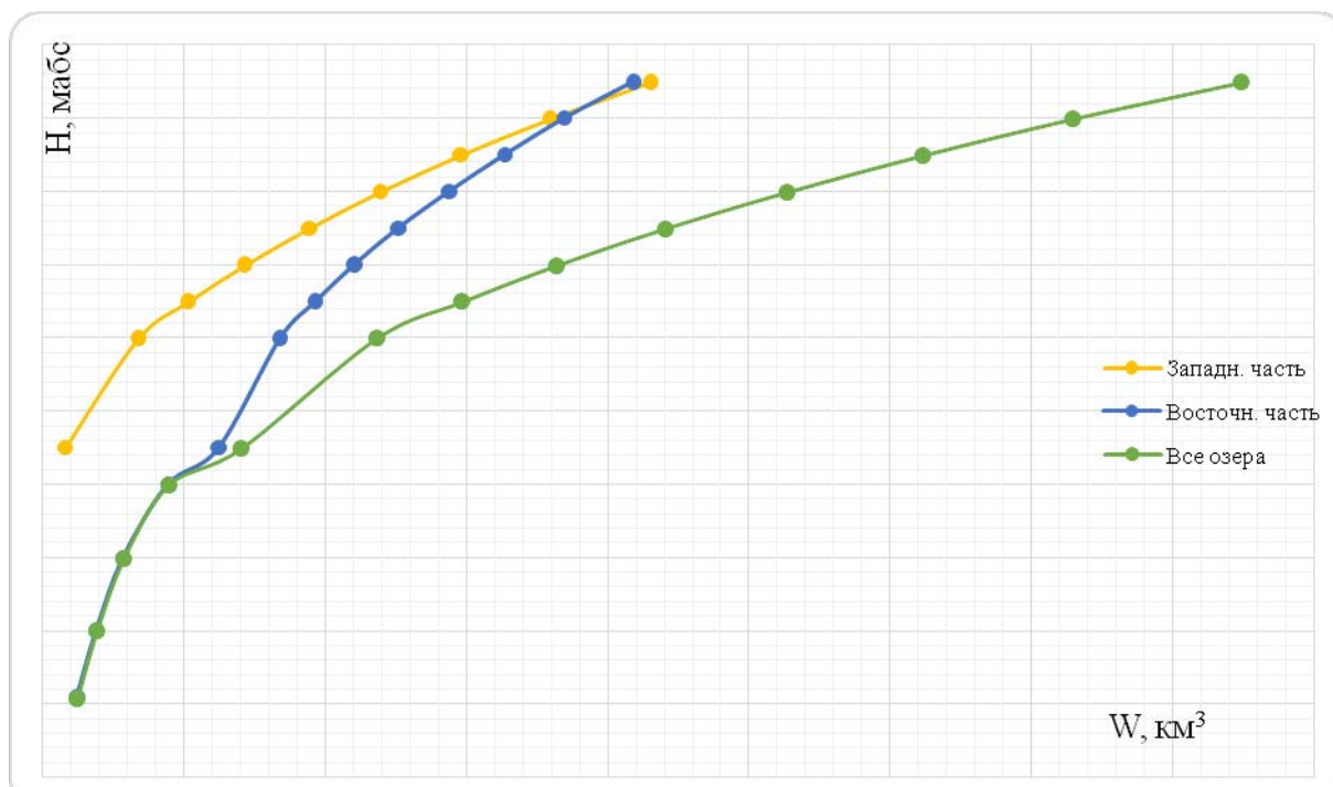
Рисунок 3 – Кривые зависимости площади зеркала озера Балхаш от уровня в нем
