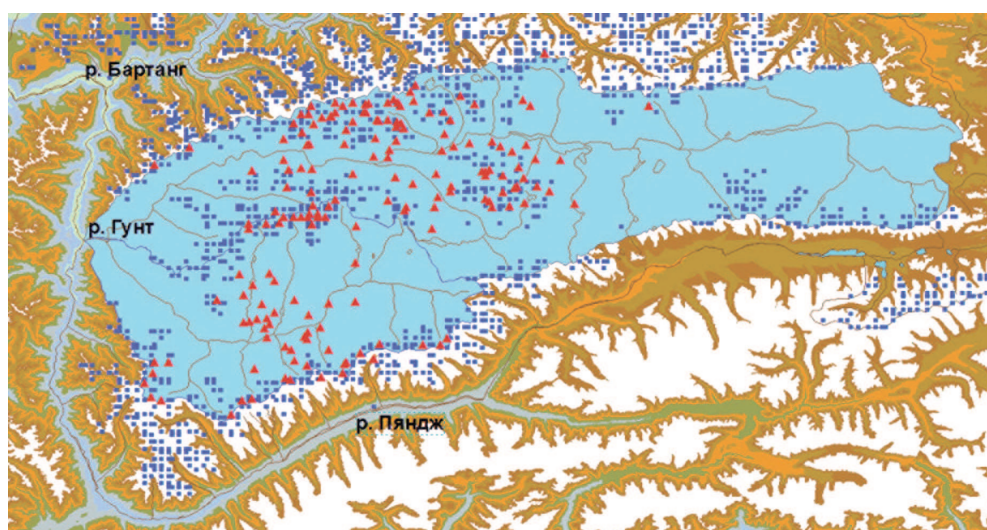
Рис. 1. Пример генерализации совокупности ледников в бассейне р. Гунт (Памир)
