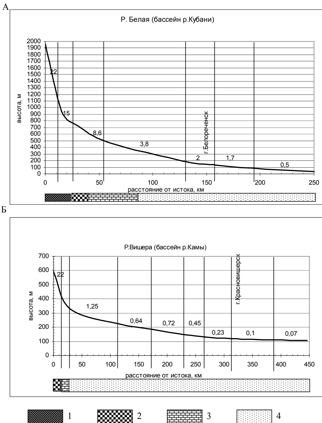
Рис. 3. Типичные продольные профили рек в переходных зонах Северного Кавказа (А) и западного склона Урала (Б). Морфодинамические типы русел: 1 – порожиисто-водопад-ные; 2 –
