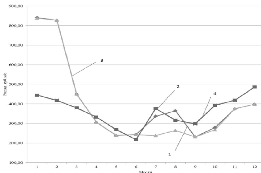
Рис. 1. График расходов ВВ и НВ в створе Курпсайской ГЭС: 1 – приток к створу в 2008 г., 2 – приток к створу в 2009 г., 3 – расход через гидроагрегаты в 2008 г., 4 – расход через гидроагрегаты в 2009 г.
