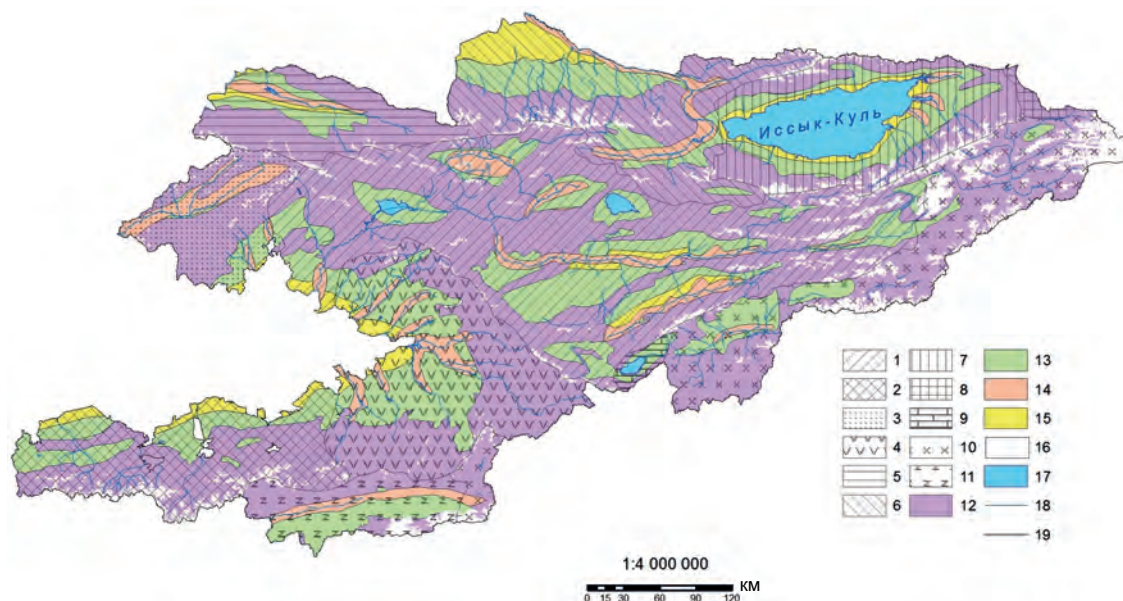
Рисунок 1. Карта геогидрологического районирования Кыргызской Республики. 1–11 гидрологические бассейны: 1 – р. Нарын; 2 – рек южного обрамления Ферганской долины (р. Сырдарья); 3 – рек северного обрамления Ферганской долины (р. Сырдарья); 4 – р. Карадарья; 5 – р. Талас; 6 – р. Чу; 7 – оз. Иссык-Куль; 8 – оз. Балхаш; 9 – оз. Чатыр-Куль; 10 – р. Тарим; 11 – р. Амударья; 12–17 – потоки подземных вод; 12 – гидрогеологических массивов; 13 – предгорного типа; 14 – речных долин; 15 – междуречные (водораздельные); 16 – ледники; 17 – озера; 18 – реки; 19 – границы потоков.
