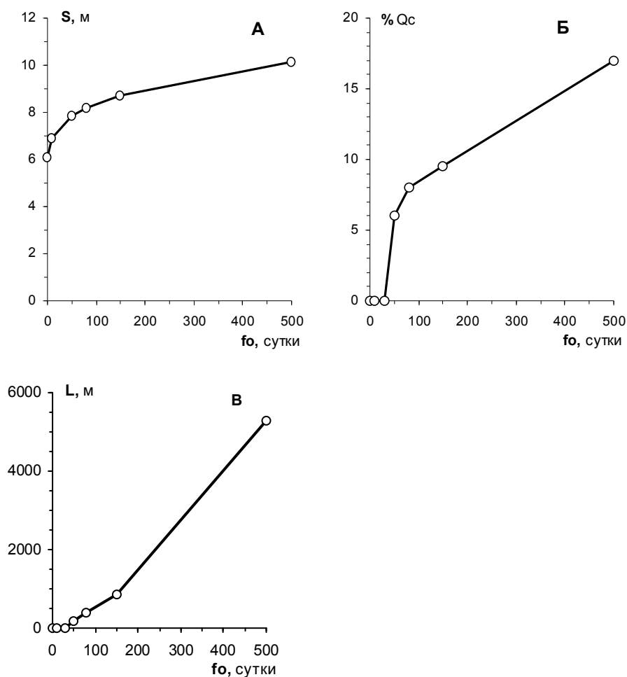
Рис. 7.11. Зависимости понижения уровня в водозаборе (А), доли притяжения из реки в свободном режиме (Б) и размера зоны отрыва (В) от удельного сопротивления экрана
