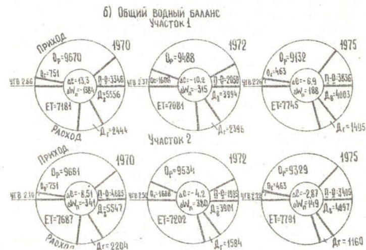
Рис. 4. Структура статей общего водного баланса зоны аэрации, м³/га: O_p - водоподачи в поле (нетто); O_a - атмосферные осадки; (-g) - питание грунтовых вод опускающейся почвенной влагой; D_g - дренажный сток; ET - эвапотранспирация; \Pi-O - разность подземного притока и оттока; \Delta W_n - изменение запасов влаги в расчетном слое; \Delta C - солевой режим. Знак - (минус) перед цифрами обозначает вынос солей; + (плюс) - накопление.
