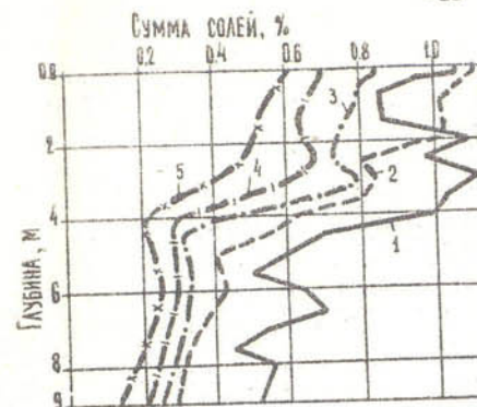
Рис. 1. Динамика рассоления почвогрунтов под влиянием вегетационных поливов и эксплуатационных промывок на фоне СВД: 1- весна 1970 г.; 2- осень 1970 г.; 3- осень 1972 г.; 4- осень 1974 г.; 5- осень 1980 г.
