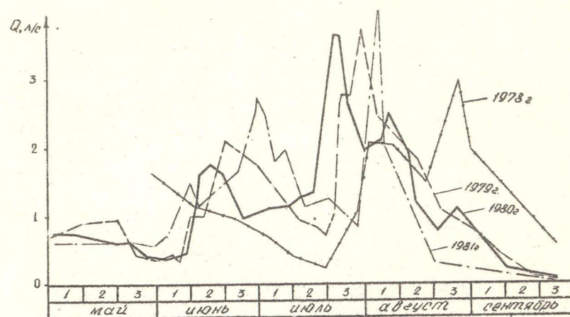
Рис. 7. Гидрографы дренажного стока дрен Iа-Д-85 из трубофильтров.
