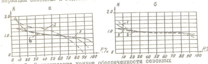
Рис.1. Эмпирические кривые обеспеченности сезонных значений дренажного модуля:
